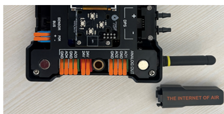
EUT Encloser Open
