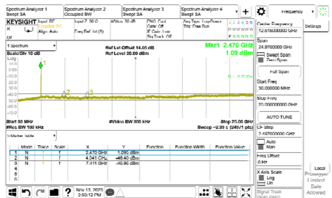
802.11ax_20MHz_WLAN2_2462MHz_RU52_40
