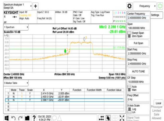
802.11ax_20MHz_WLAN1_2412MHz_RU26_0
