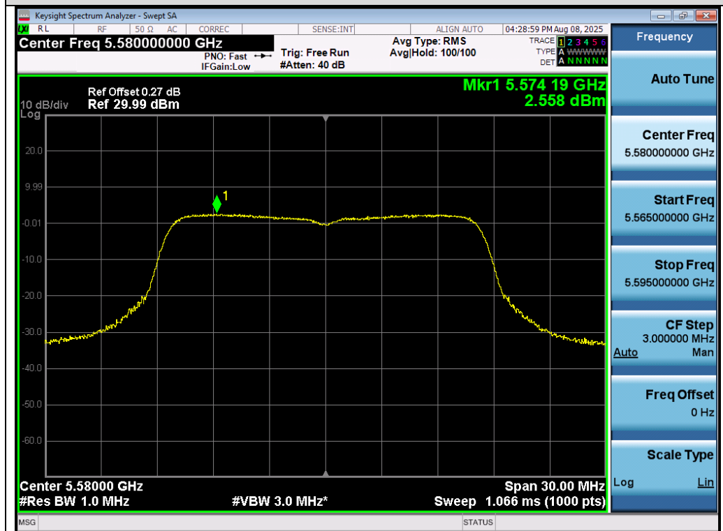
Test_Graph_802.11a_ANT1_5580_6Mbps_PSD
