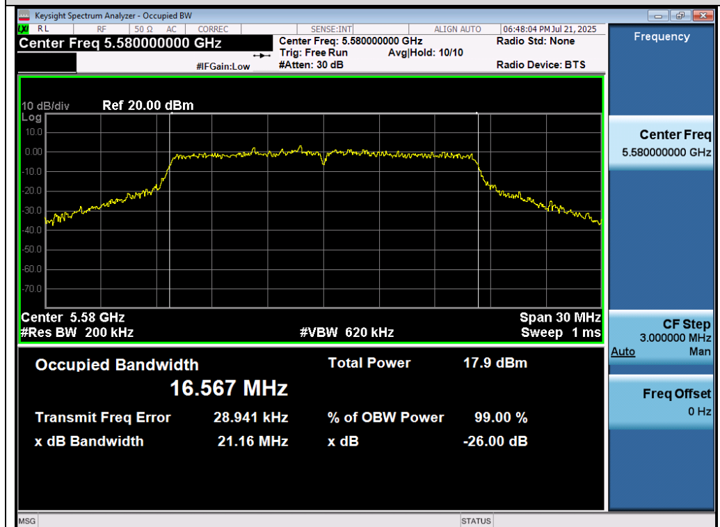
Test_Graph_802.11a_ANT1_5580_6Mbps_OBW
