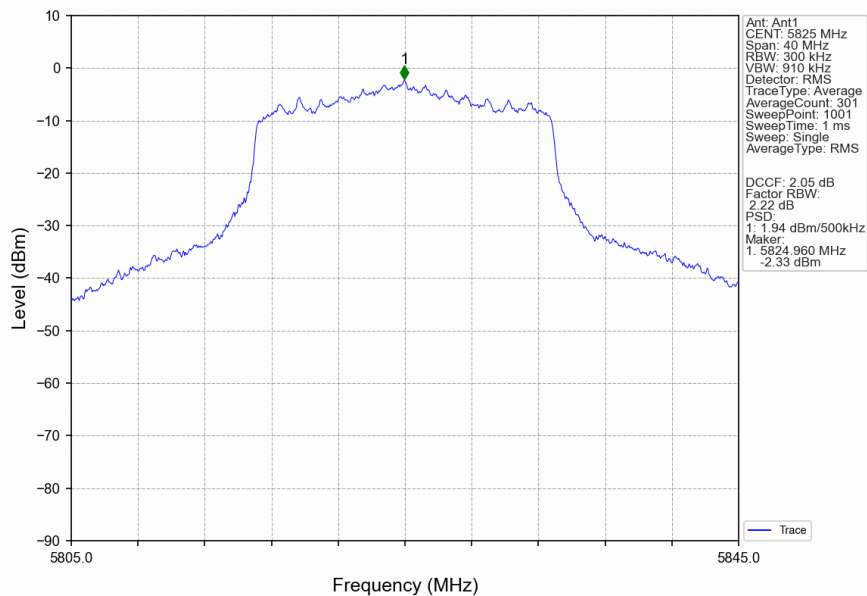
802.11n(HT20)_HCH_5825MHz_Ant1_NTNV
