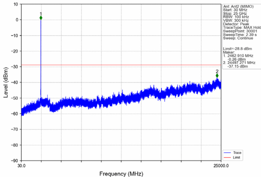
802.11n(HT20)_HCH_2462MHz_Ant2 (MIMO)_NTNV
