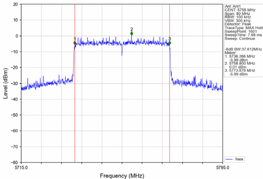
802.11ax(HEW40)_LCH_5755MHz_RU484_Left_Ant1_NTNV
