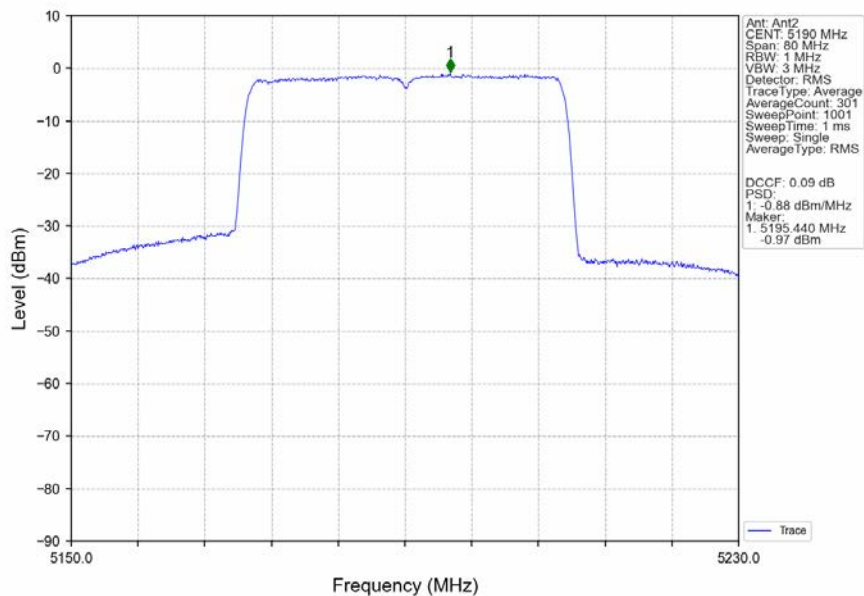
802.11ax(HEW40)_LCH_5190MHz_RU484_Left_Ant2_NTNV
