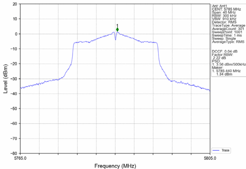
802.11n(HT20)_MCH_5785MHz_Ant1_NTNV
