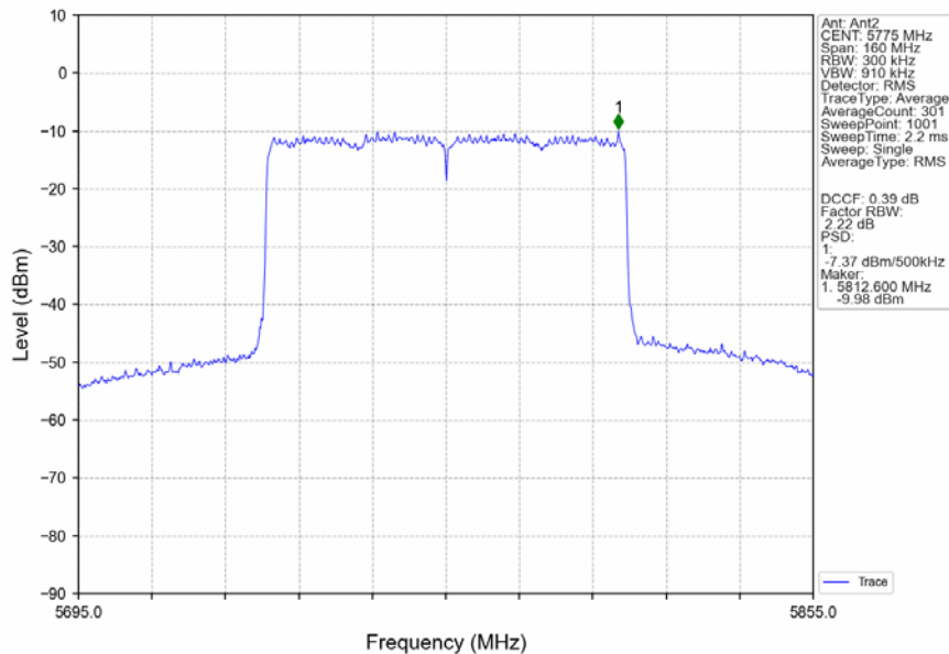
802.11ax(HEW80)_MCH_5775MHz_RU996_Left_Ant2_NTNV
