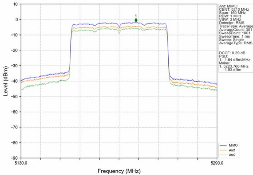
802.11ax(HEW80)_MCH_5210MHz_RU996_Left_MIMO_NTNV
