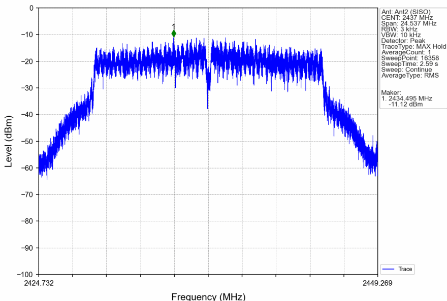
802.11g_MCH_2437MHz_Ant2 (SISO)_NTNV
