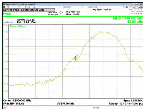
GPRS1900_Low_Band edge
