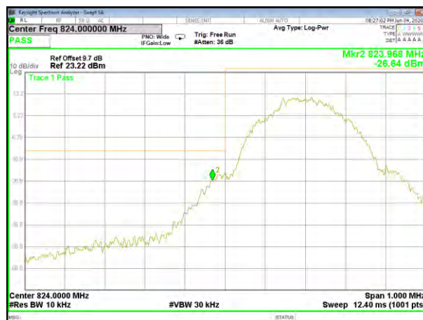
GPRS850_Low_Band edge
