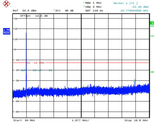
20MHz_Middle_QPSK_100@0
