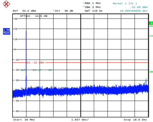
20MHz_Low_QPSK_100@0
