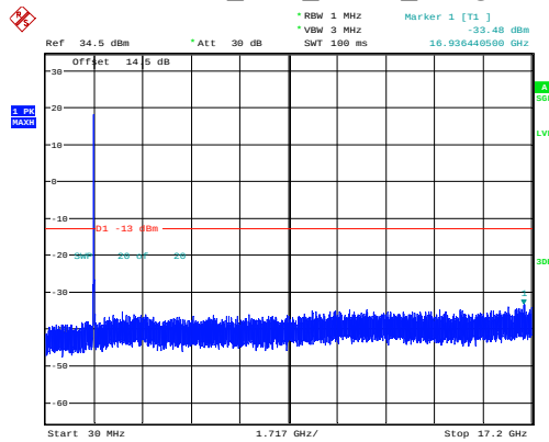
20MHz_Low_QPSK_100@0
