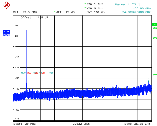
20MHz_Middle_QPSK_100@0
