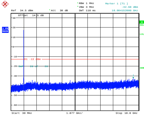
10MHz_Middle_QPSK_50@0
