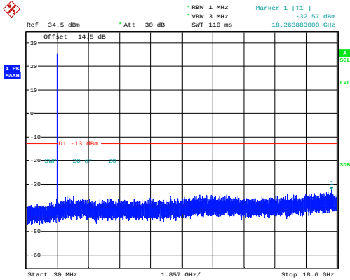
20MHz_Low_QPSK_1@0
