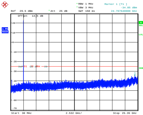
20MHz_Middle_QPSK_1@0
