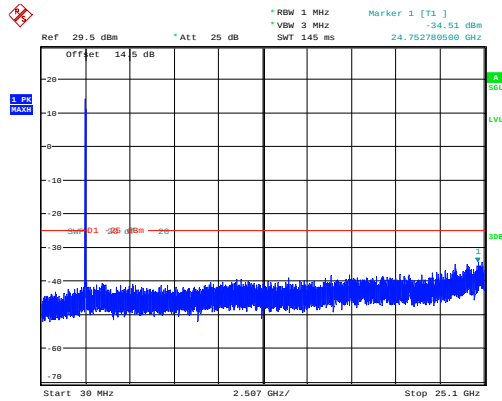
20MHz_Low_QPSK_100@0
