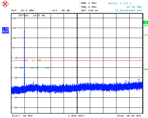
10MHz_Low_QPSK_50@0
