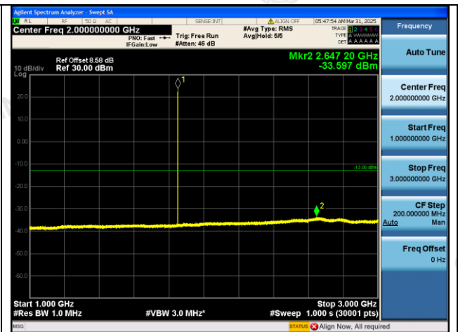
GPRS1900-512-0-1000~3000MHz-PASS
