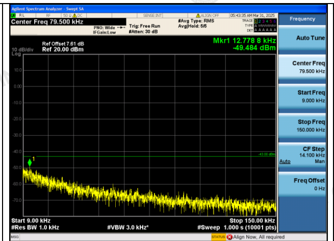
GPRS1900-810-0-0.009~0.15MHz-PASS
