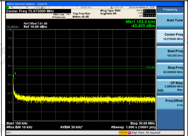
GPRS1900-810-0-0.15~30MHz-PASS
