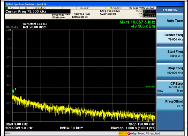
GPRS1900-661-0-0.009~0.15MHz-PASS
