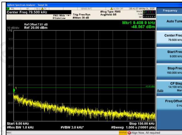
GSM1900-810-0-0.009~0.15MHz-PASS
