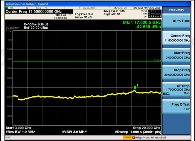
GPRS1900-512-0-3000~20000MHz-PASS
