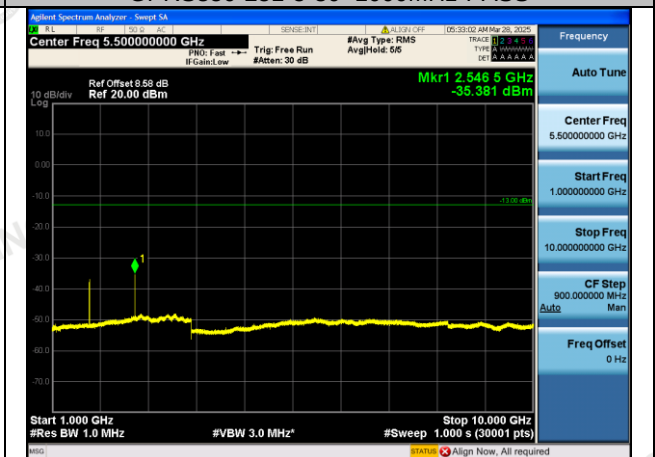
GPRS850-251-5-1000~10000MHz-PASS
