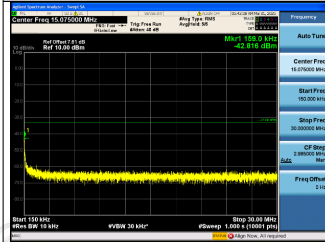
GSM1900-810-0-0.15~30MHz-PASS
