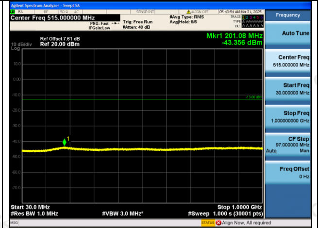
GPRS1900-810-0-30~1000MHz-PASS
