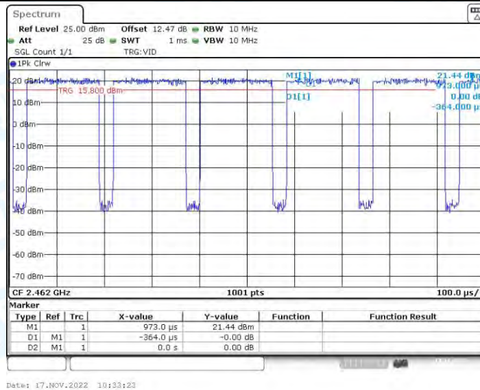
VHT20_Ant2_2462
