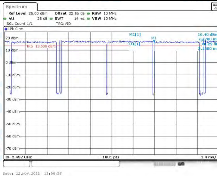
11AX20-BF_Ant2_2437
