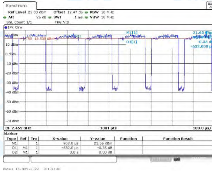
VHT40_Ant2_2452
