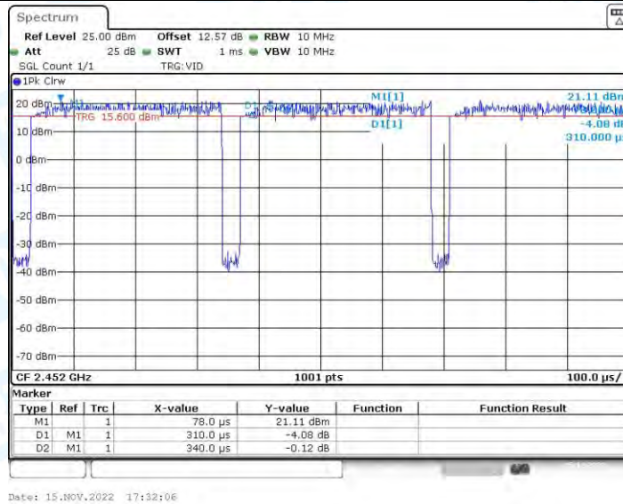
11AX40_Ant2_2452
