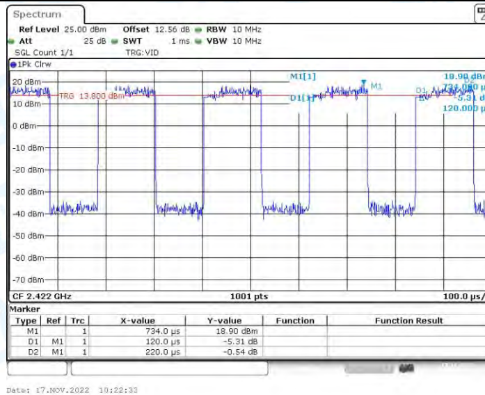
11N40_Ant2_2422
