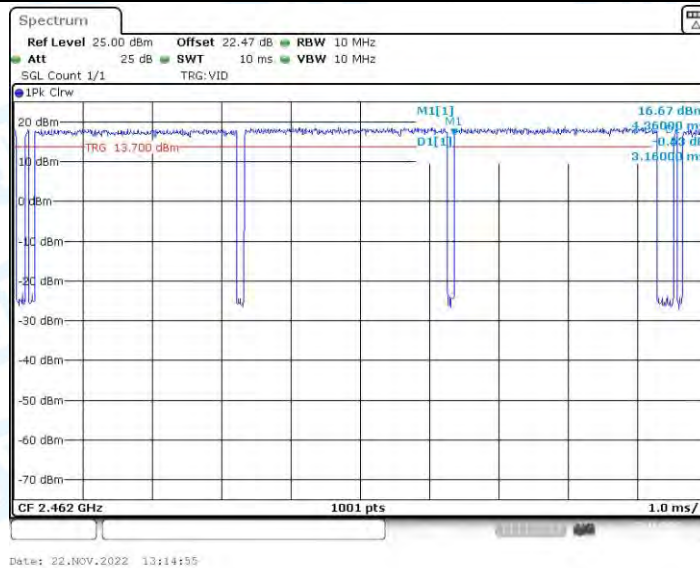
11AX20-BF_Ant2_2462
