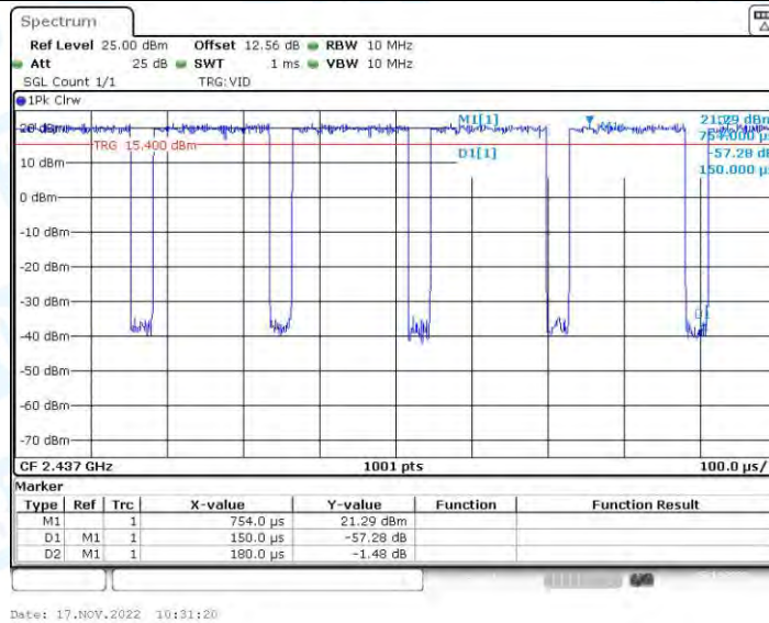
VHT20_Ant2_2437
