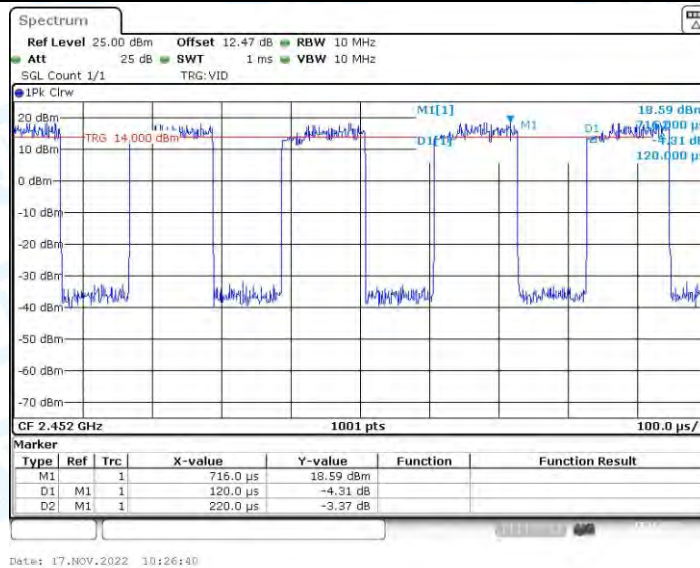
11N40_Ant2_2452
