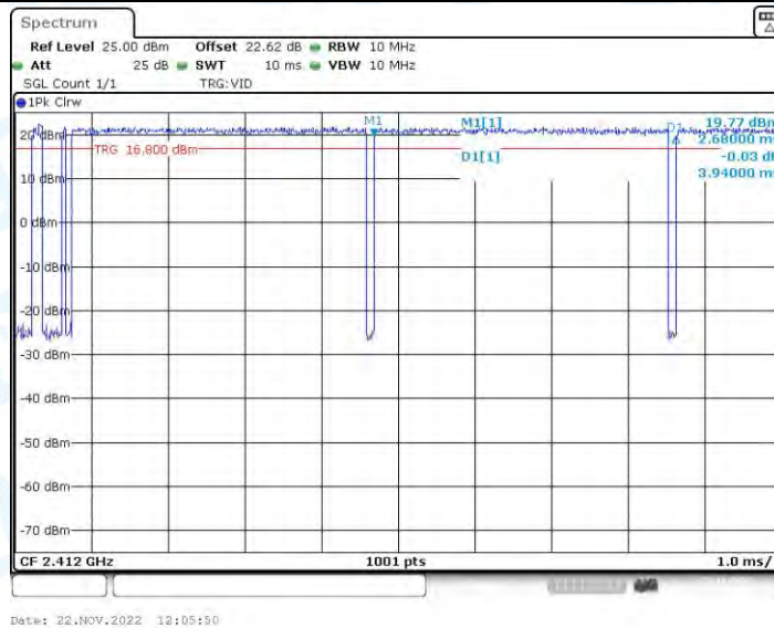
VHT20-BF_Ant2_2412
