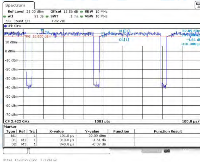
11AX40_Ant2_2422
