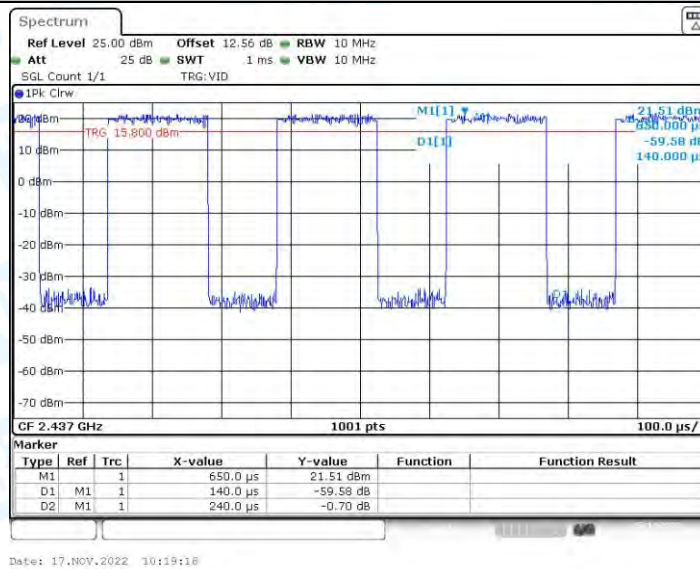
11N20_Ant2_2437
