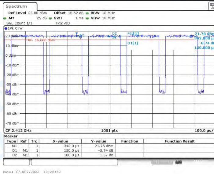
VHT20_Ant2_2412
