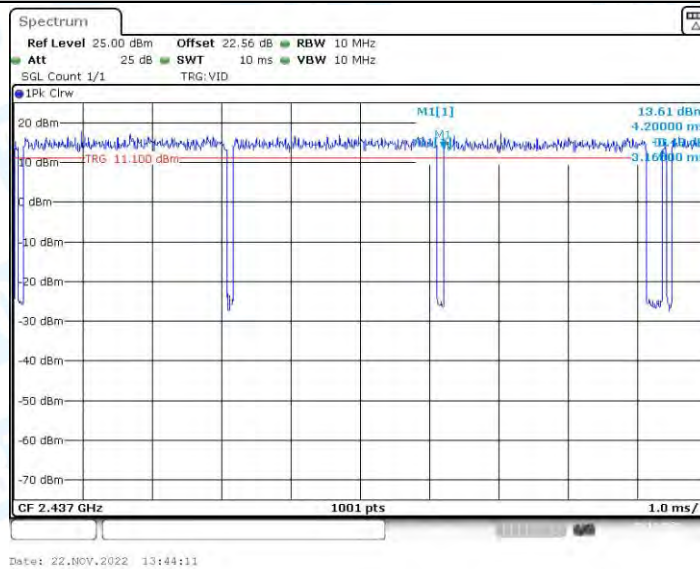
11AX40-BF_Ant2_2437
