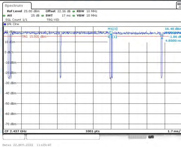
11N40-BF_Ant2_2437
