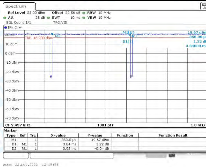
VHT20-BF_Ant2_2437
