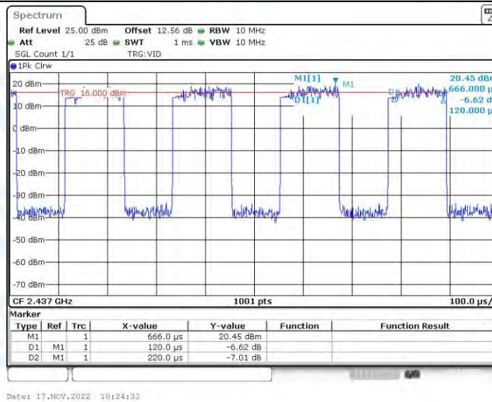
11N40_Ant2_2437
