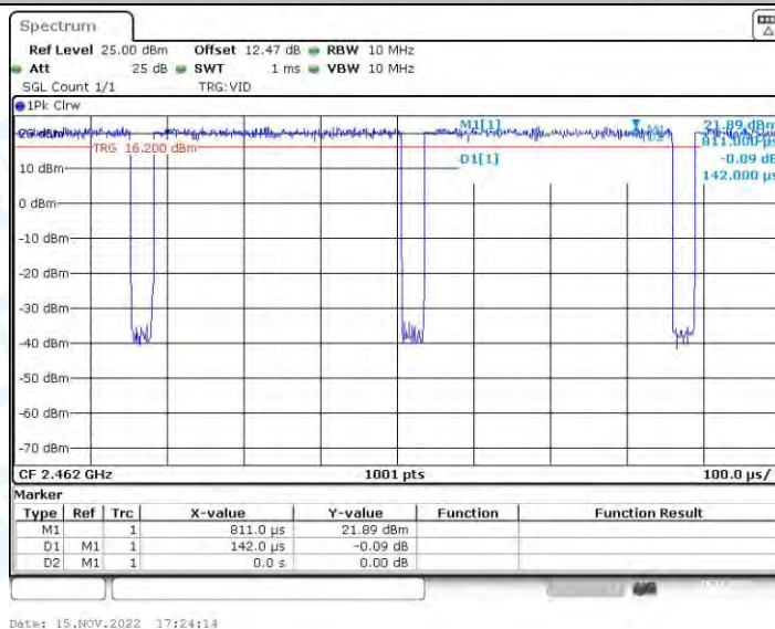
11AX20_Ant2_2462
