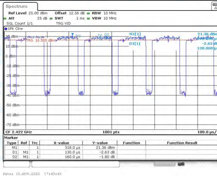
VHT40_Ant2_2422
