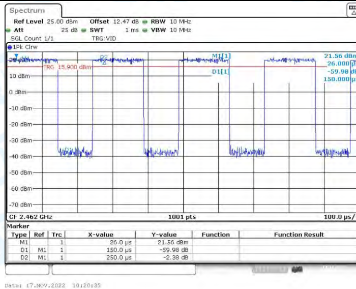
11N20_Ant2_2462
