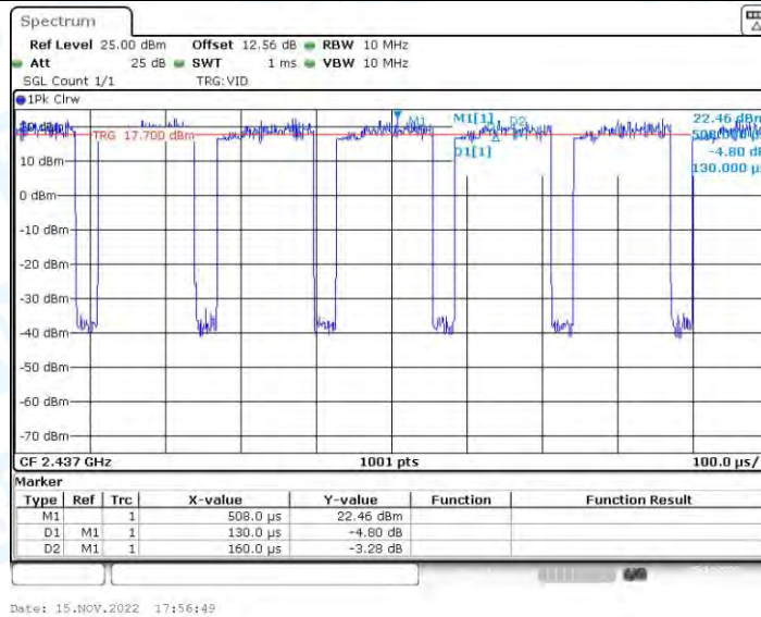
VHT40_Ant2_2437
