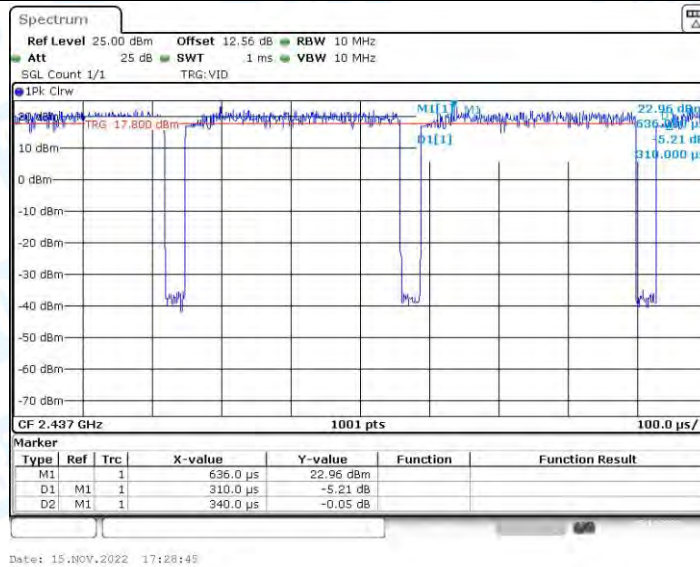
11AX40_Ant2_2437
