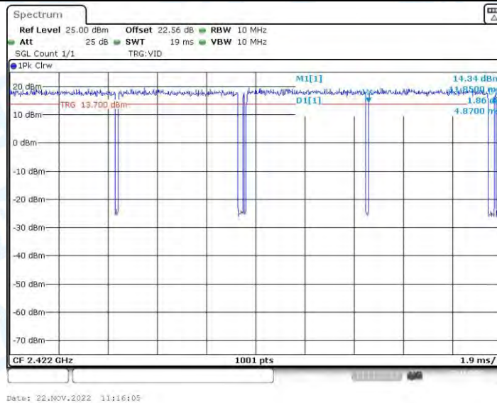
11N40-BF_Ant2_2422
