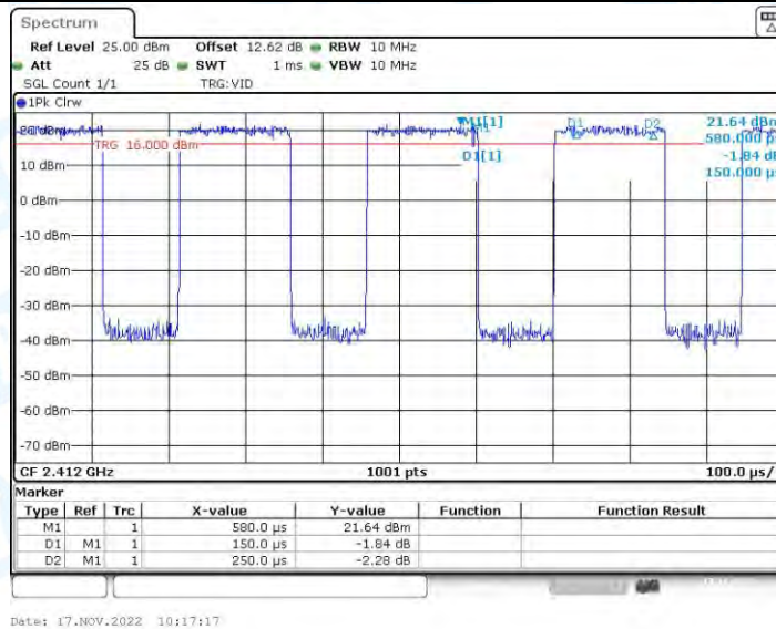
11N20_Ant2_2412
