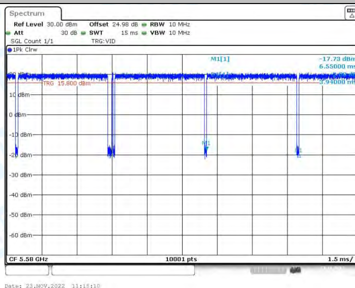
11N20-BF_Ant2_5580
