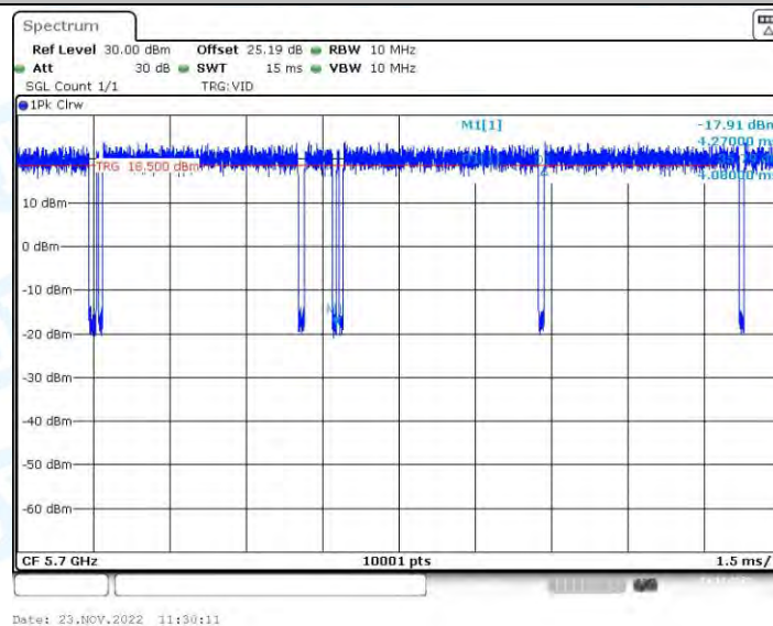
11N20-BF_Ant2_5700
