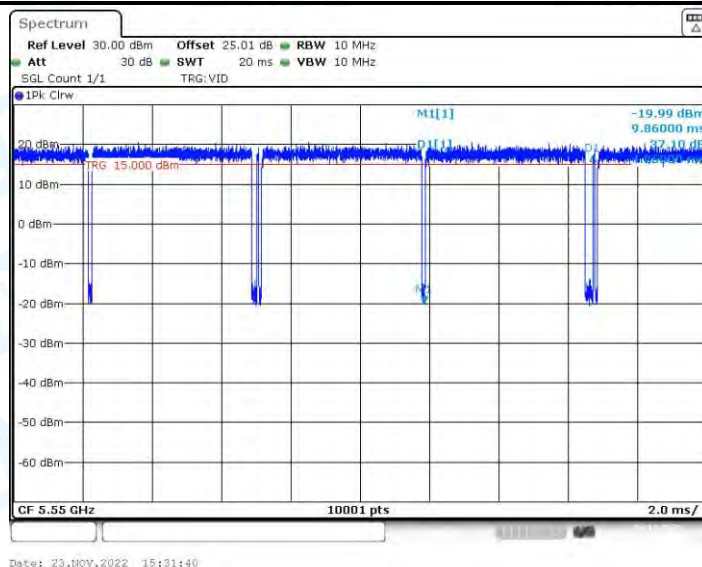
11N40-BF_Ant2_5550
