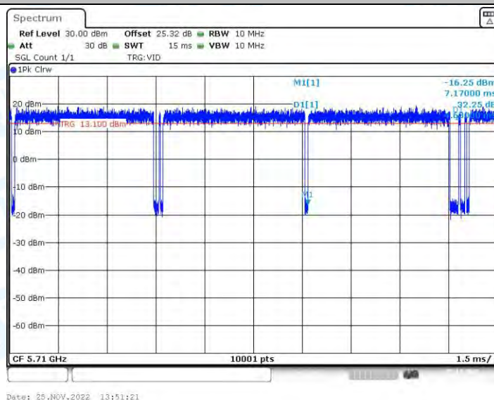
11AX40-BF_Ant2_5710
