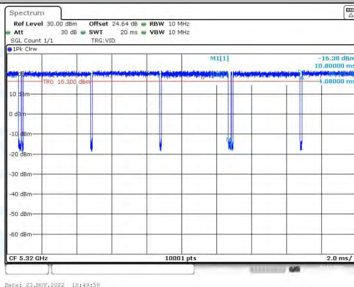
11N20-BF_Ant2_5320
