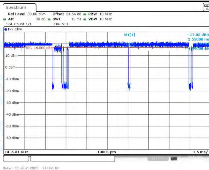
11AX40-BF_Ant2_5310
