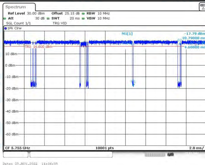
11AX40-BF_Ant2_5755
