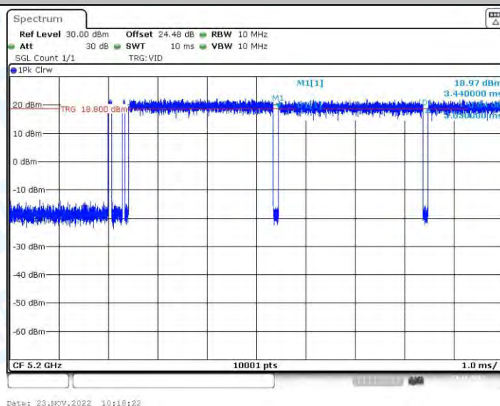
11AX20-BF_Ant2_5200
