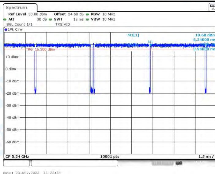
11AC20-BF_Ant2_5240
