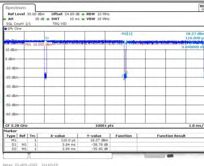
11N20-BF_Ant2_5280
