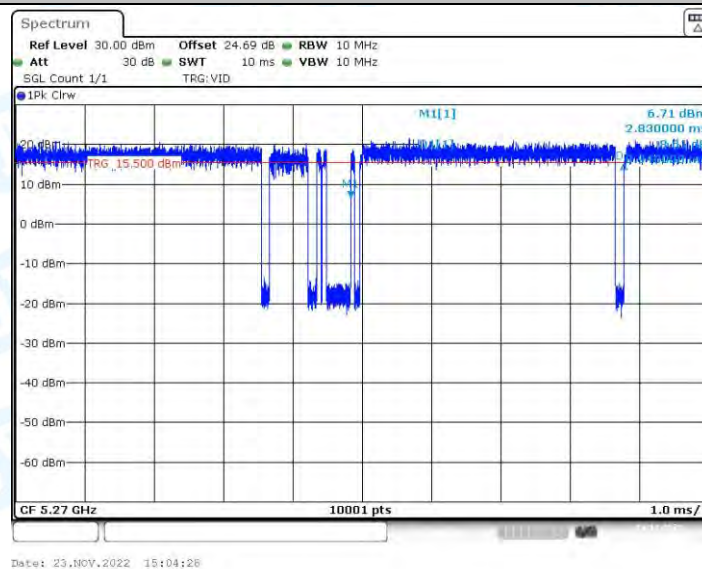
11AC40-BF_Ant2_5270
