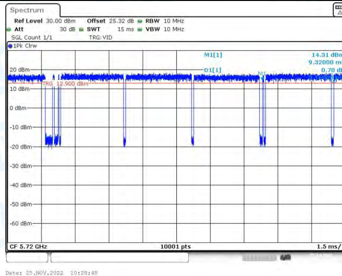
11AX20-BF_Ant2_5720
