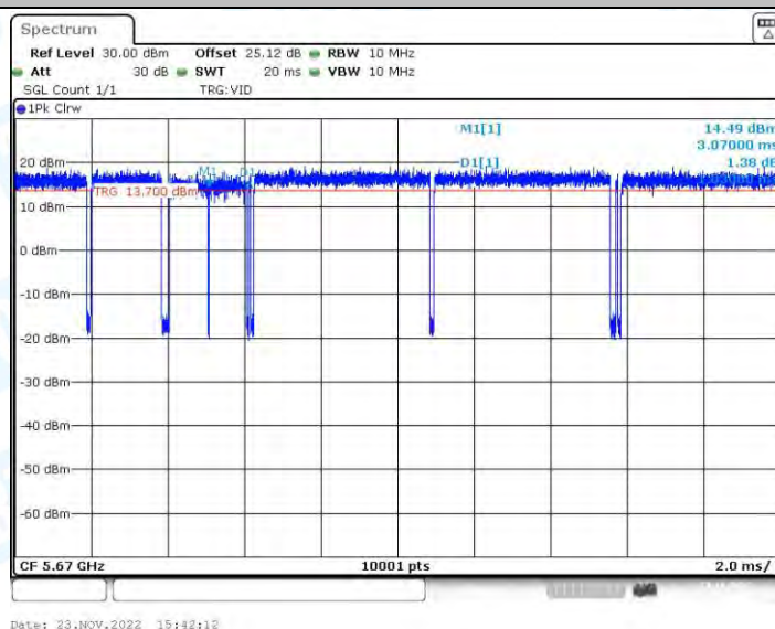
11N40-BF_Ant2_5670
