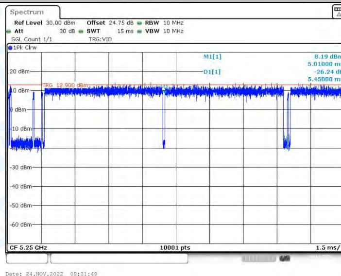
11AC160-BF_Ant2_5250
