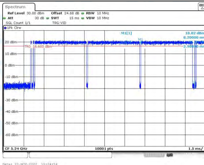
11N20-BF_Ant2_5240
