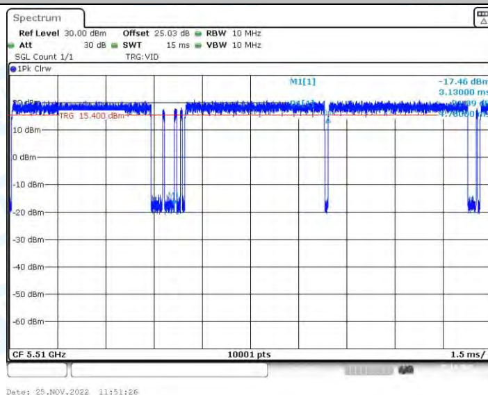
11AX40-BF_Ant2_5510
