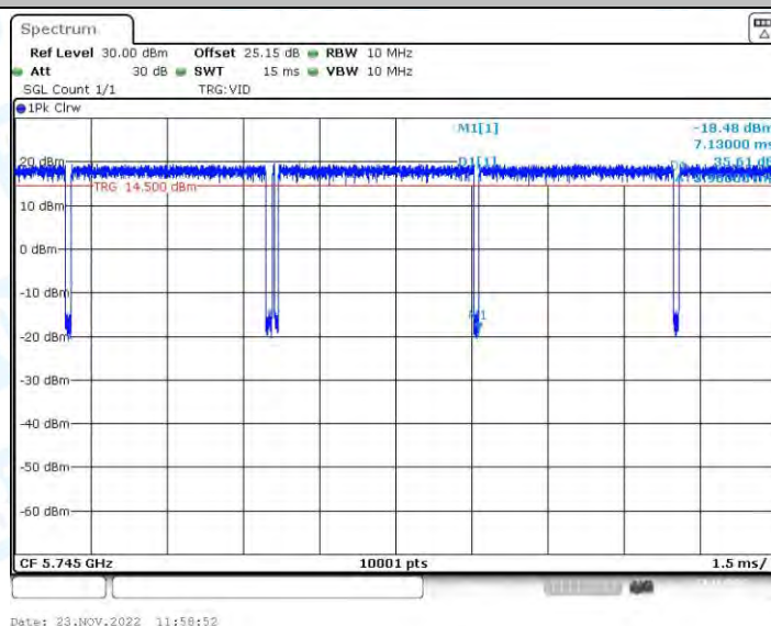
11N20-BF_Ant2_5745
