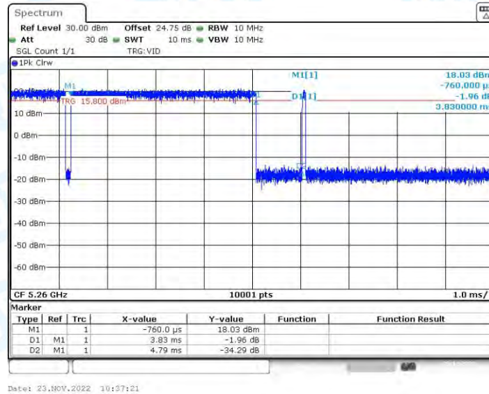
11AC20-BF_Ant2_5260
