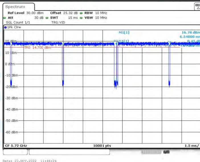
11N20-BF_Ant2_5720
