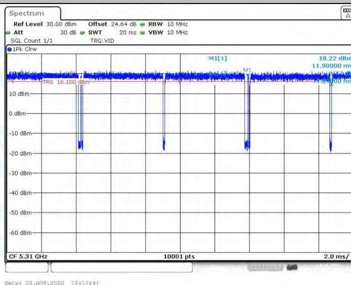
11N40-BF_Ant2_5310
