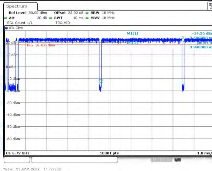
11AC20-BF_Ant2_5720
