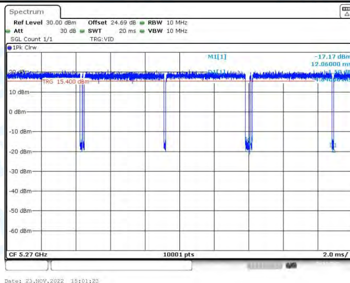
11N40-BF_Ant2_5270
