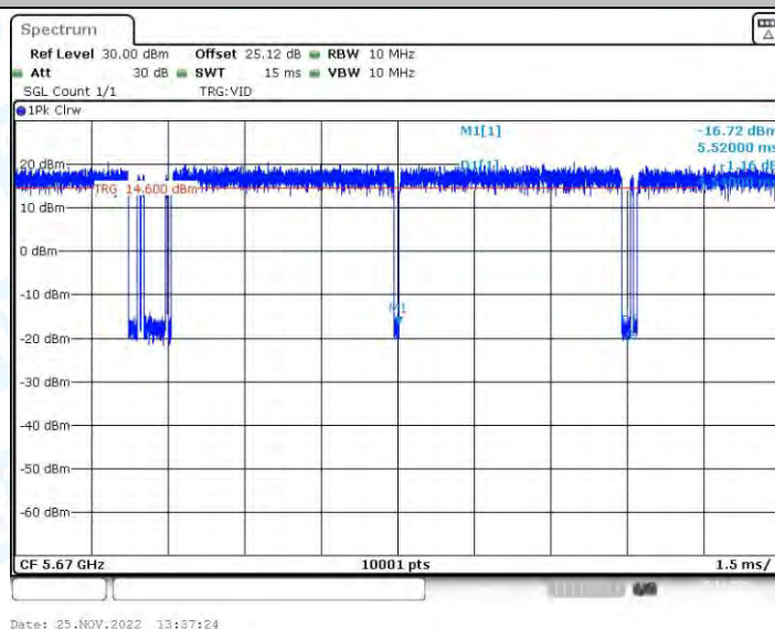
11AX40-BF_Ant2_5670
