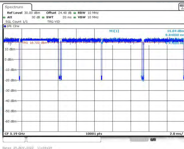
11AX40-BF_Ant2_5190
