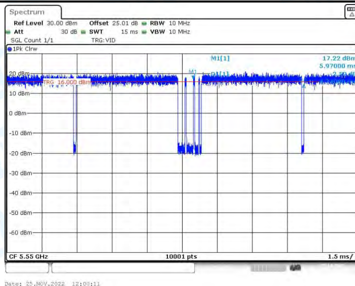
11AX40-BF_Ant2_5550
