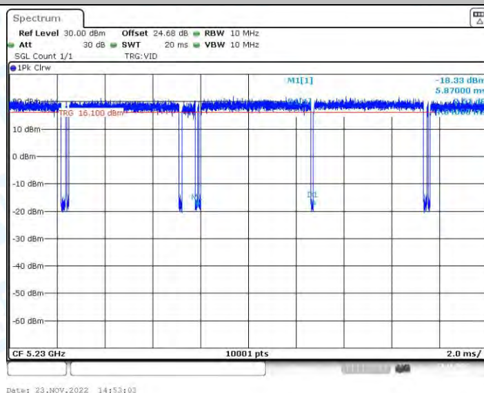
11AC40-BF_Ant2_5230
