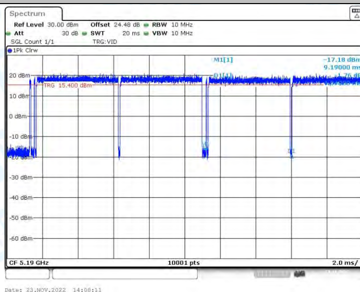
11N40-BF_Ant2_5190
