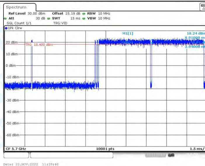
11AC20-BF_Ant2_5700
