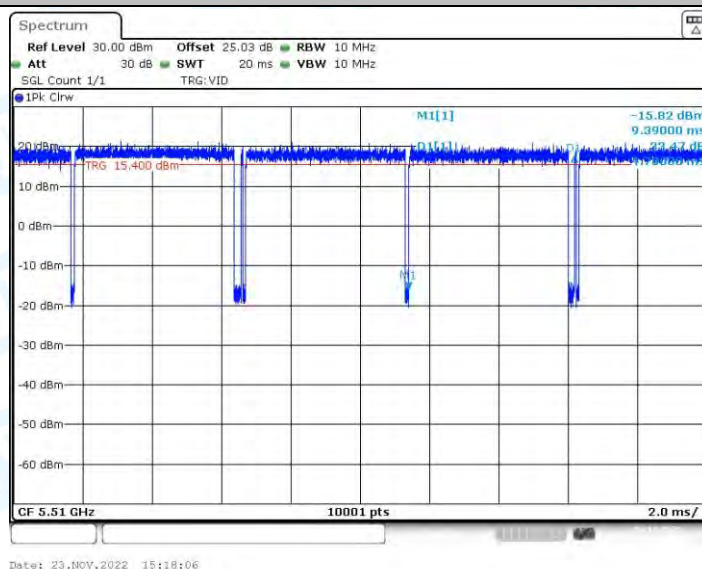
11N40-BF_Ant2_5510
