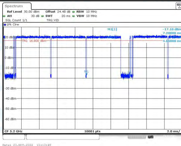
11AC20-BF_Ant2_5200
