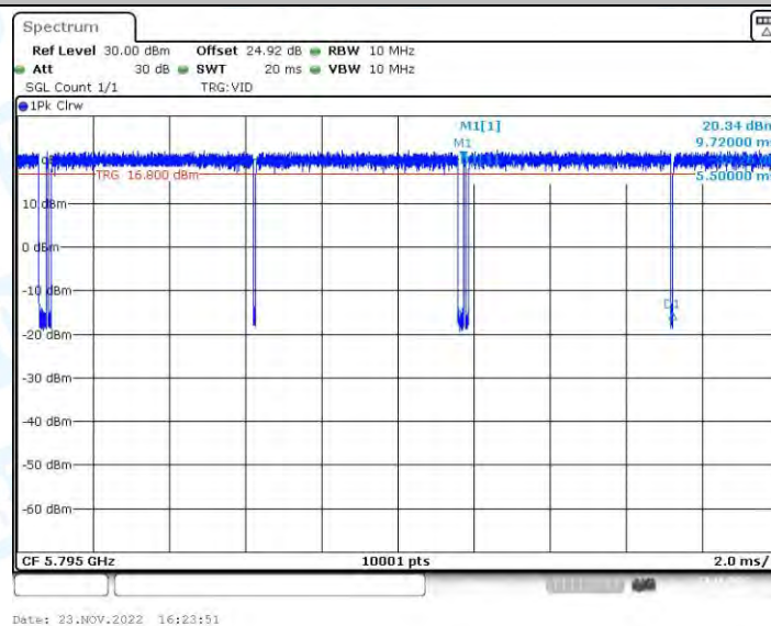
11N40-BF_Ant2_5795
