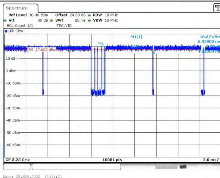
11AX40-BF_Ant2_5230
