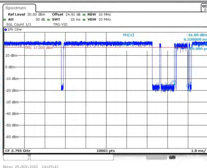
11AX40-BF_Ant2_5795
