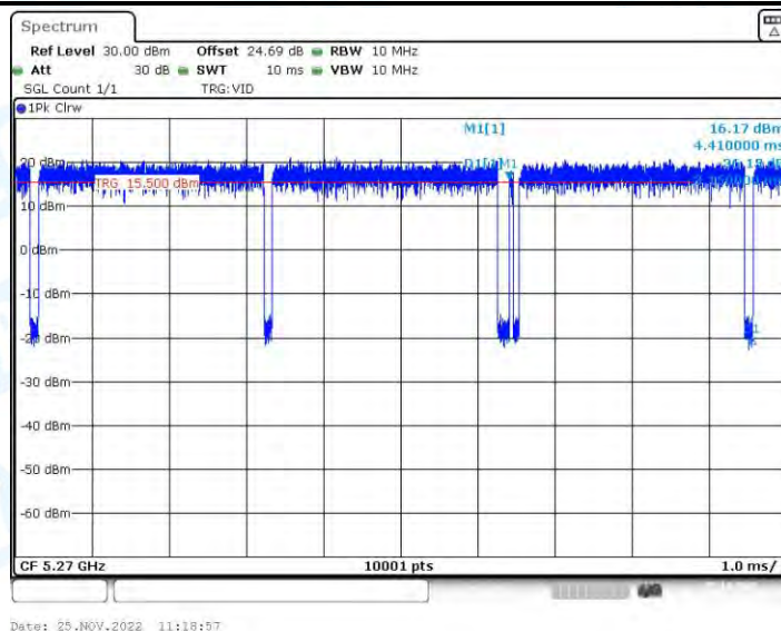
11AX40-BF_Ant2_5270
