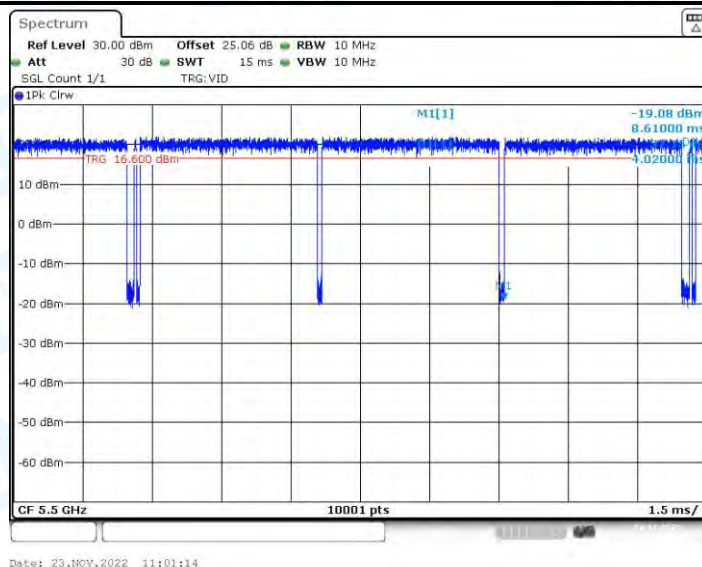
11N20-BF_Ant2_5500
