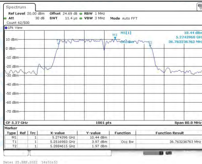
11N40-SDM_Ant2_5270
