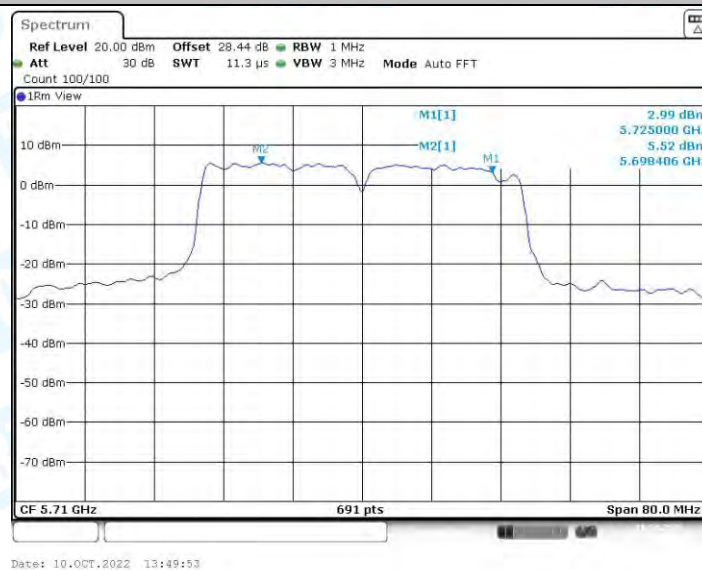
11N40-SDM_Ant1_5710_UNII-3
