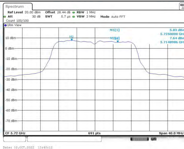
11N20-SDM_Ant1_5720_UNII-3
