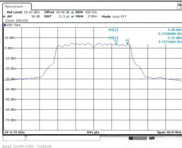
11A_Ant2_5720_UNII-3
