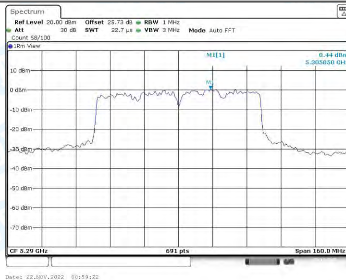
11AC80-CDD_Ant2_5290
