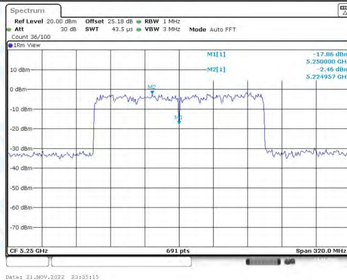
11AX160-CDD_Ant2_5250_UNII-1
