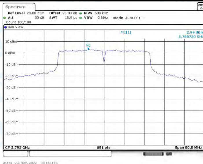
11N40-BF_Ant2_5795
