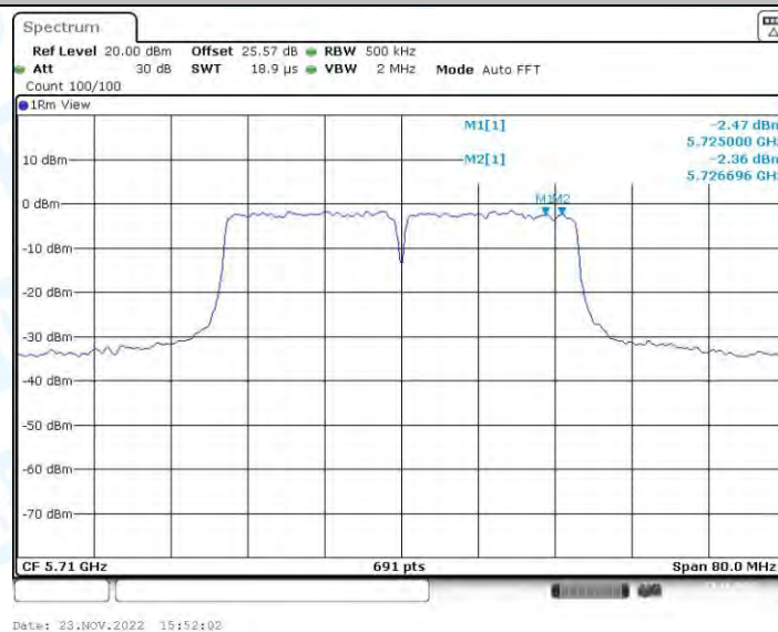
11N40-BF_Ant2_5710_UNII-3
