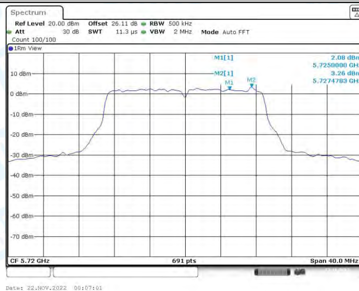
11AC20-CDD_Ant2_5720_UNII-3
