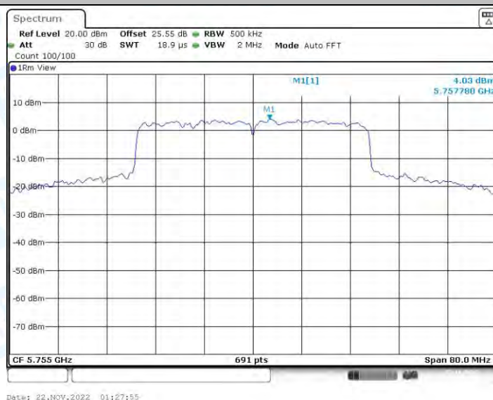
11AX40-CDD_Ant2_5755
