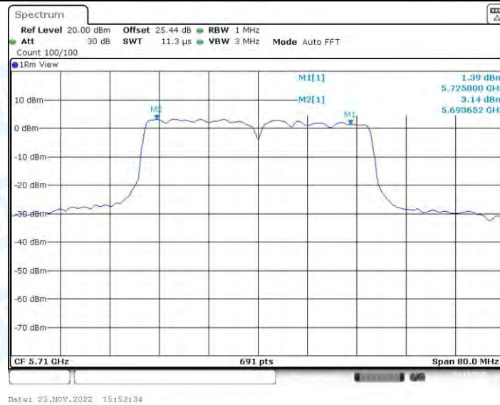
11N40-BF_Ant1_5710_UNII-3
