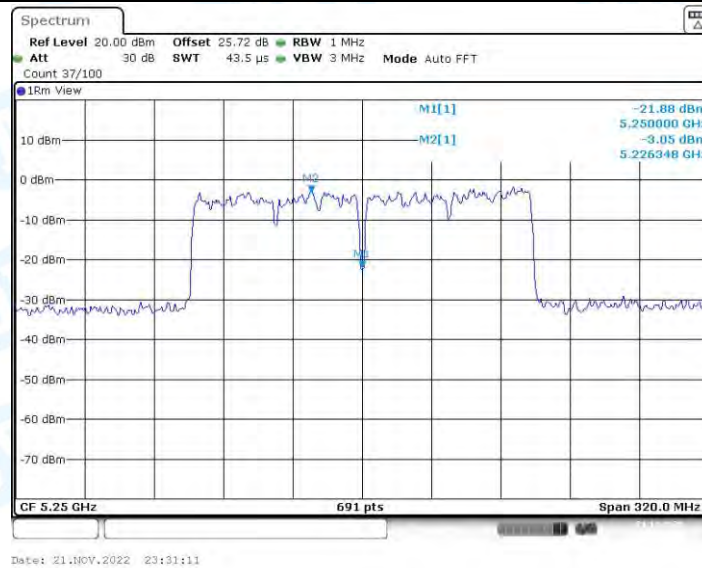
11AC160-CDD_Ant2_5250_UNII-1
