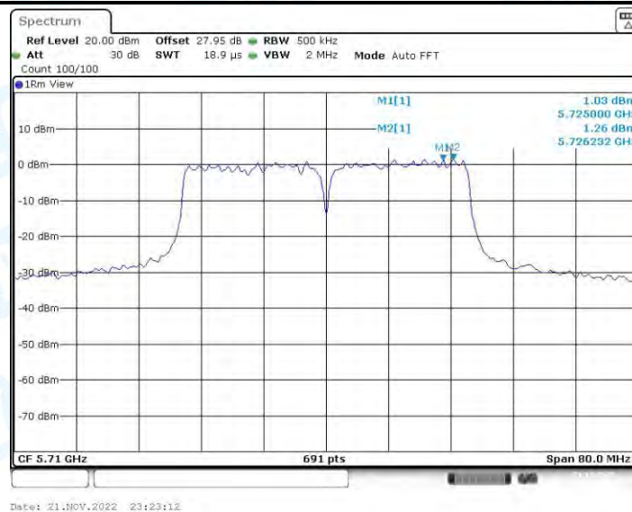
11N40-CDD_Ant2_5710_UNII-3
