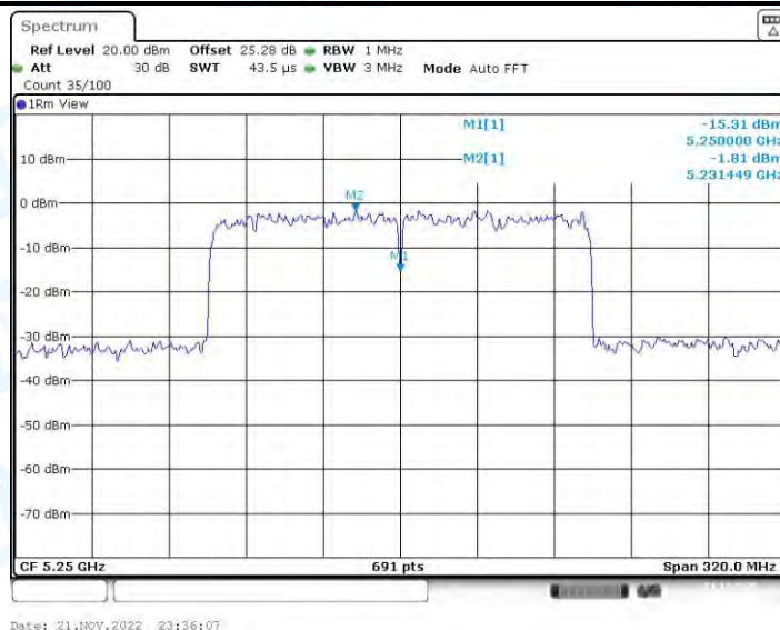
11AX160-CDD_Ant1_5250_UNII-2A
