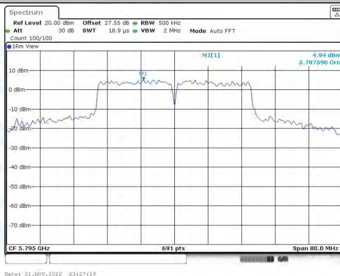
11N40-CDD_Ant2_5795
