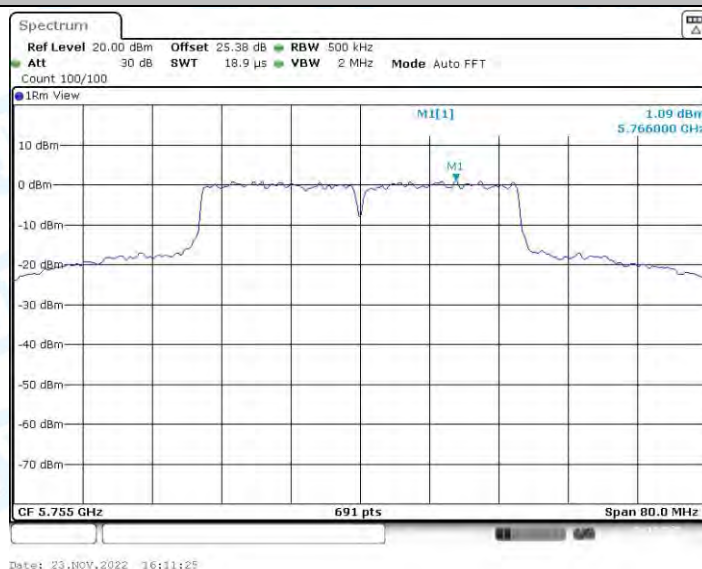
11N40-BF_Ant2_5755
