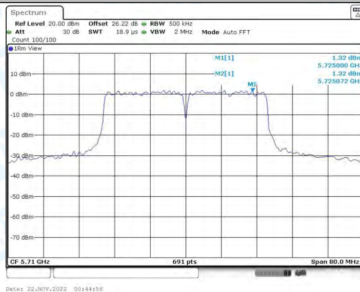
11AC40-CDD_Ant2_5710_UNII-3
