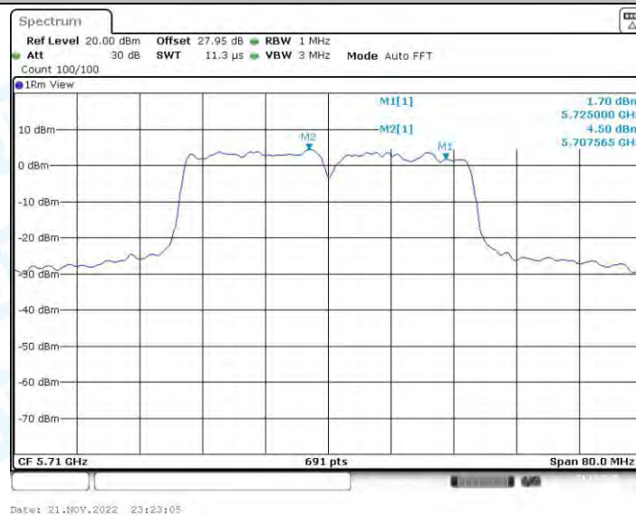
11N40-CDD_Ant2_5710_UNII-2C
