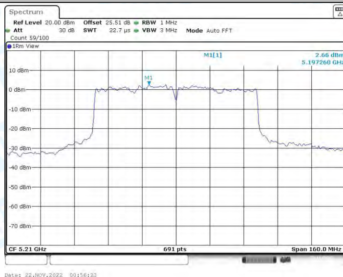
11AC80-CDD_Ant2_5210
