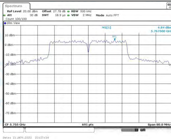
11N40-CDD_Ant2_5755
