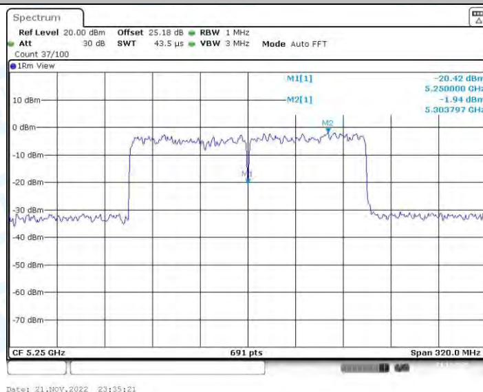
11AX160-CDD_Ant2_5250_UNII-2A
