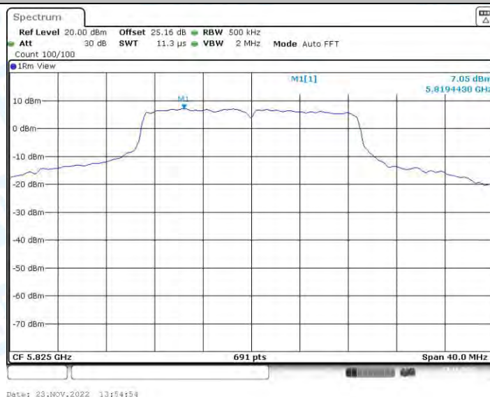
11N20-BF_Ant2_5825
