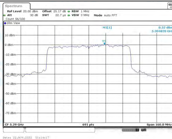
11AX80-CDD_Ant2_5290
