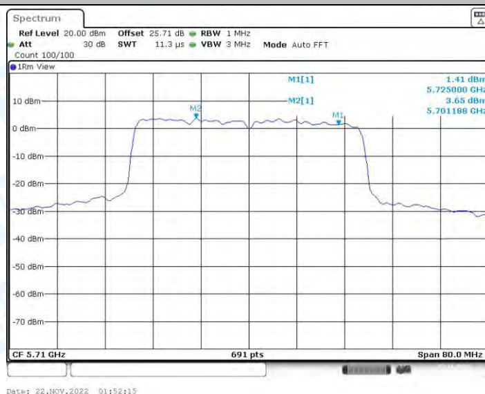
11AX40-CDD_Ant1_5710_UNII-3
