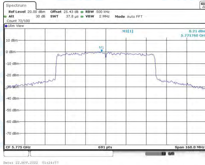
11AX80-CDD_Ant2_5775
