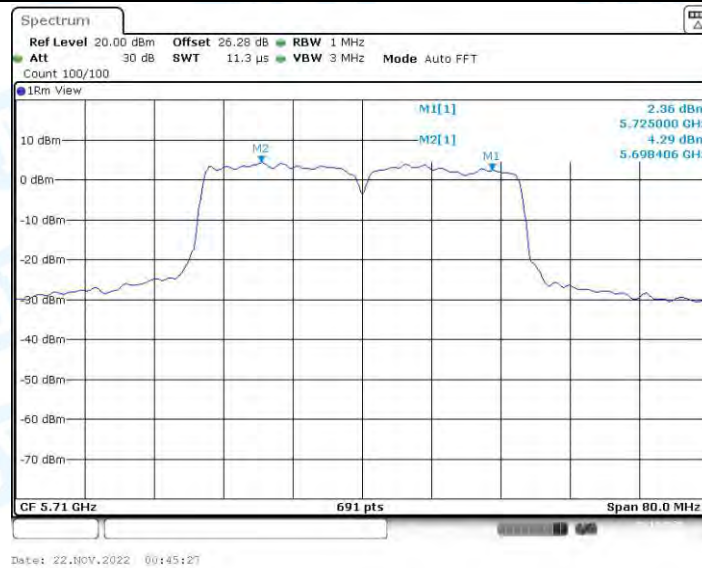
11AC40-CDD_Ant1_5710_UNII-3
