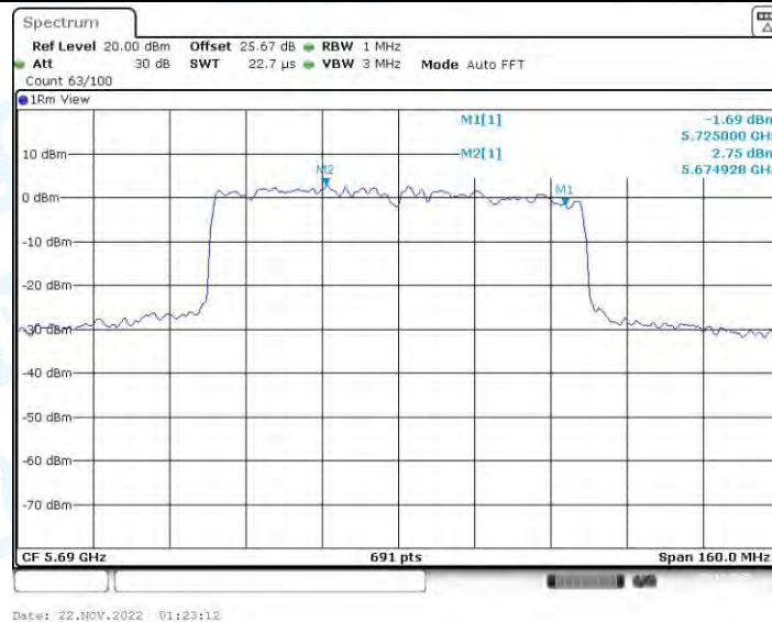
11AX80-CDD_Ant1_5690_UNII-3
