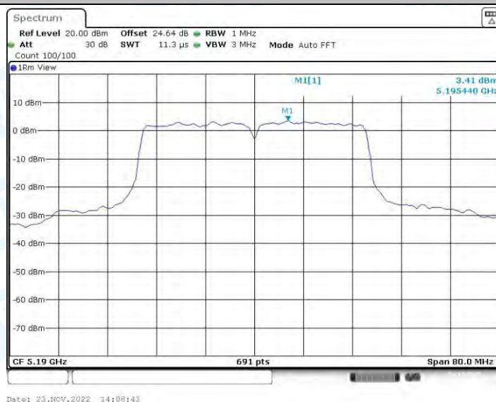
11N40-BF_Ant2_5190
