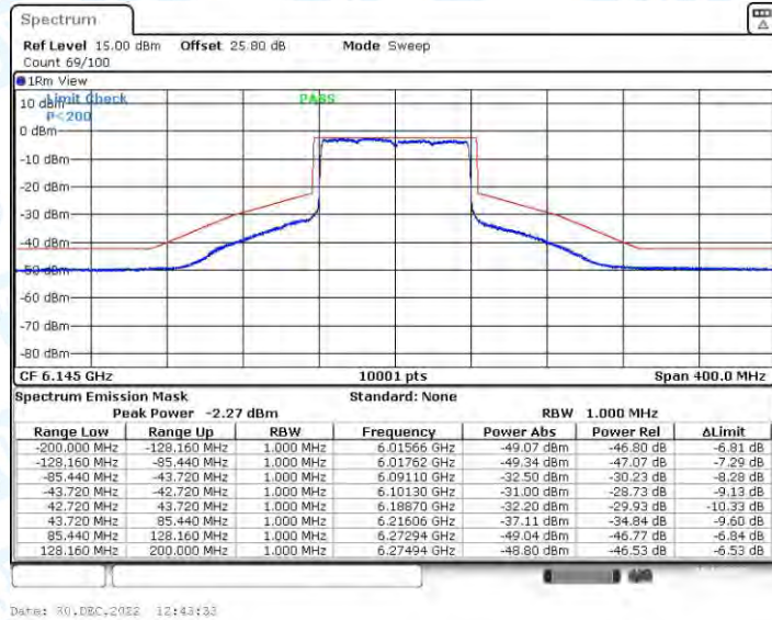
11AX80CDD_Ant3_6145
