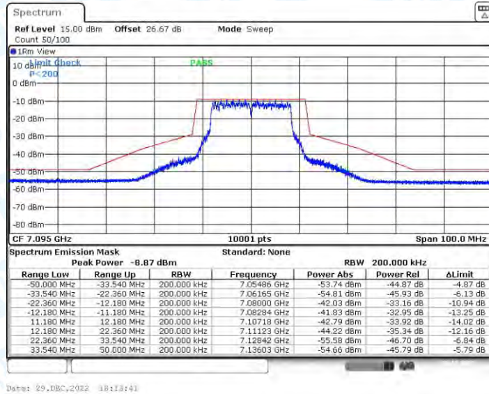
11A-CDD_Ant4_7095
