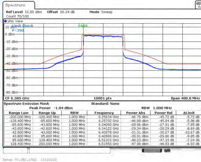
11AX80CDD_Ant2_6385
