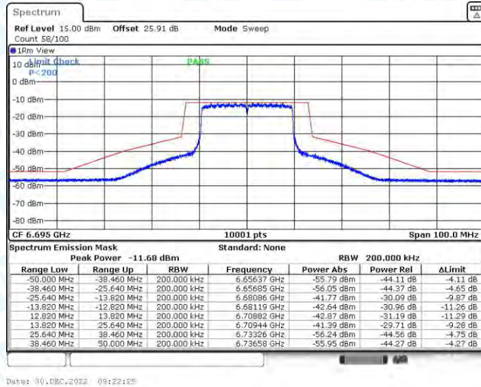
11AX20CDD_Ant2_6695
