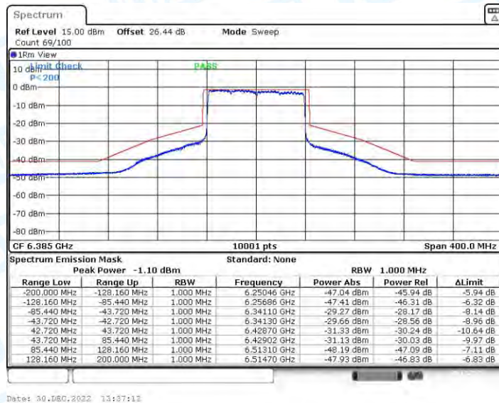
11AX80CDD_Ant4_6385
