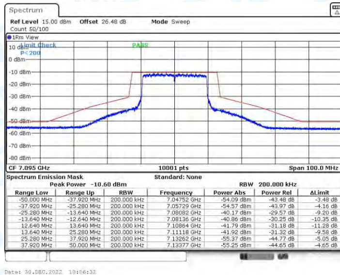
11AX20CDD_Ant2_7095
