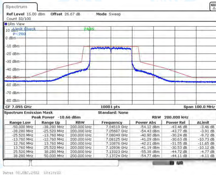
11AX20CDD_Ant4_7095
