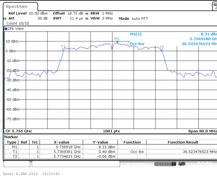
11N40-CDD_Ant2_5755
