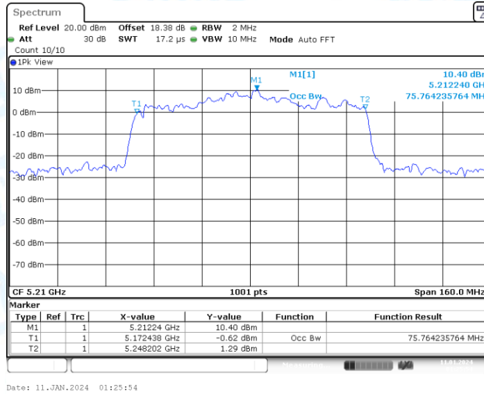
11AC80-CDD_Ant2_5210
