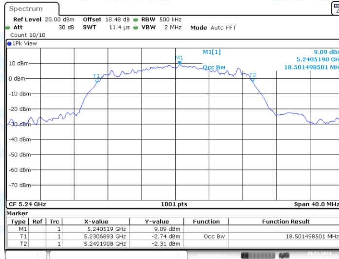
11AC20-CDD_Ant2_5240
