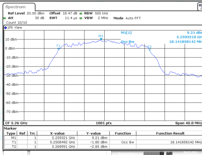
11AC20-CDD_Ant1_5260
