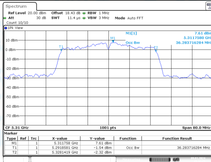
11AC40-CDD_Ant1_5310
