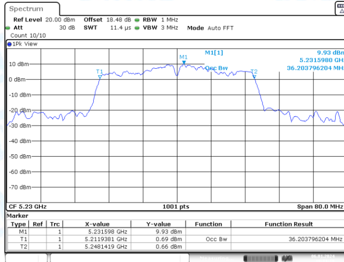
11AC40-CDD_Ant2_5230
