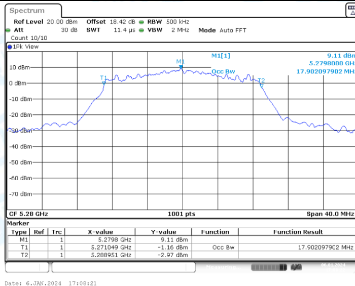
11AC20-CDD_Ant2_5280
