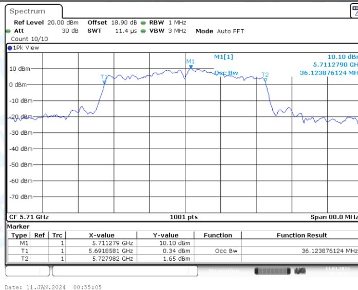
11N40-CDD_Ant2_5710
