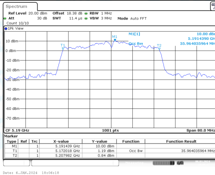
11AC40-CDD_Ant2_5190
