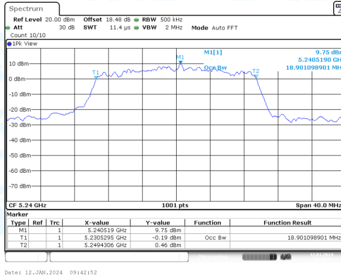
11AX20-CDD_Ant2_5240
