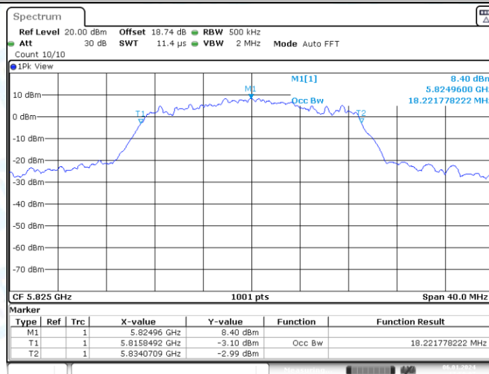
11AC20-CDD_Ant1_5825
