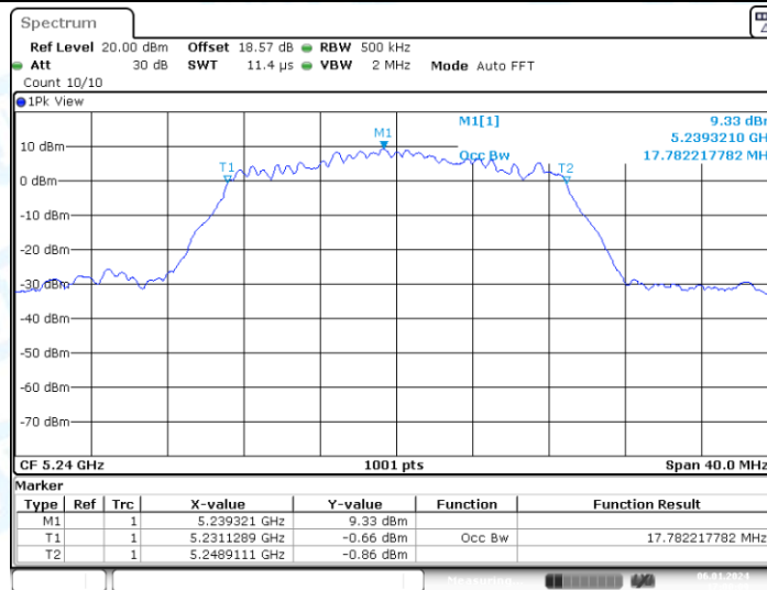
11AC20-CDD_Ant2_5240
