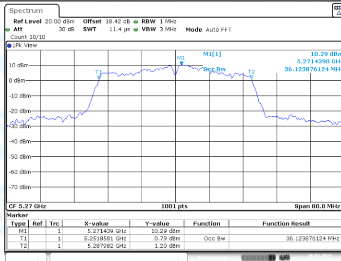
11AC40-CDD_Ant1_5270
