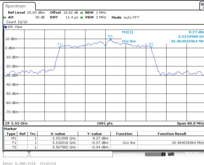
11N40-CDD_Ant2_5550
