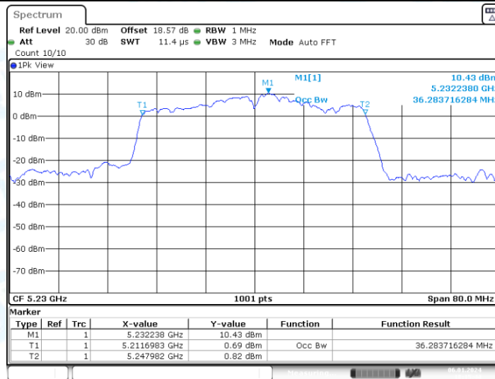
11AC40-CDD_Ant2_5230
