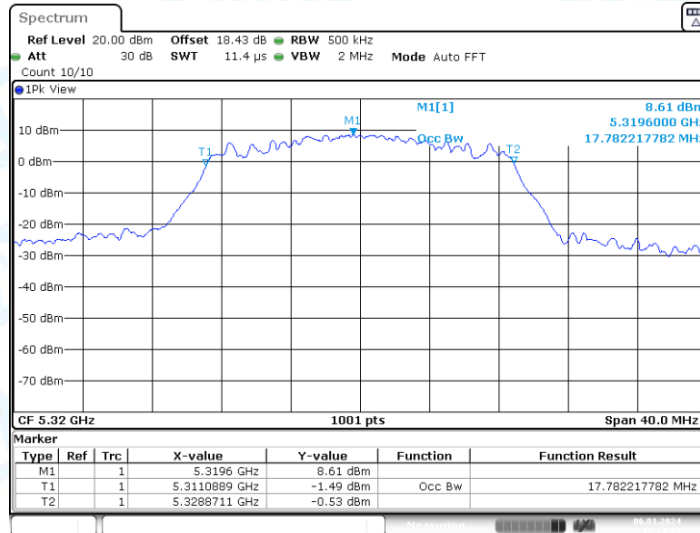
11AC20-CDD_Ant2_5320
