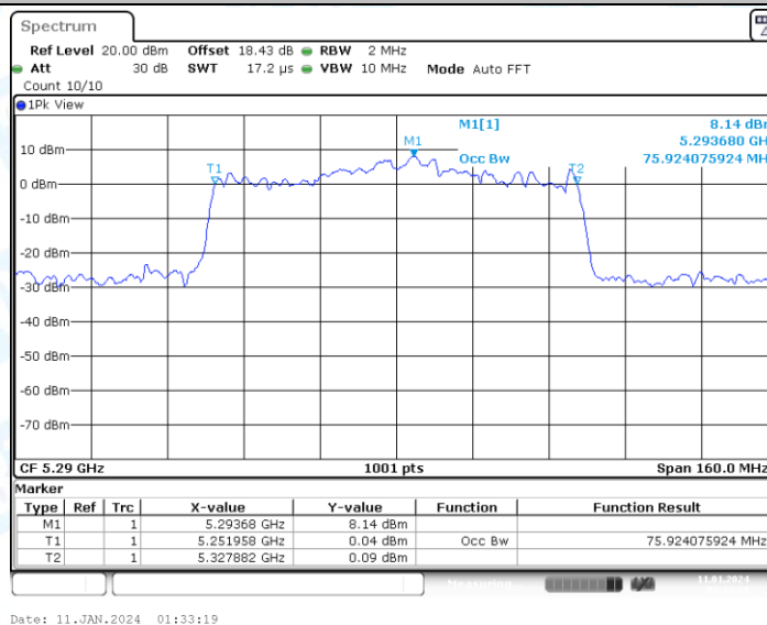
11AC80-CDD_Ant2_5290
