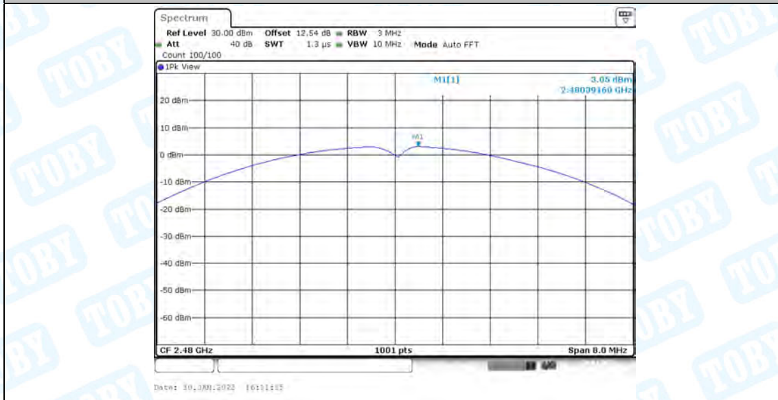
3DH5_AntA_2480
