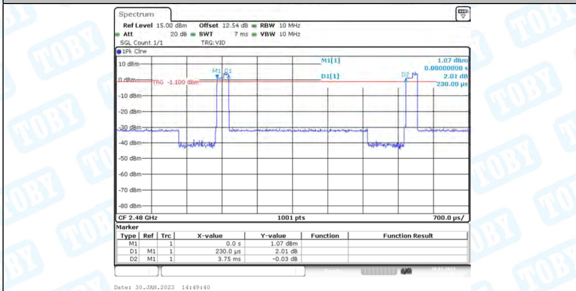
3DH5_AntA_2480
