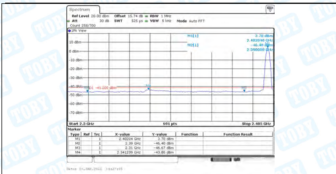
2DH5_AntA_Low_2402_Peak
