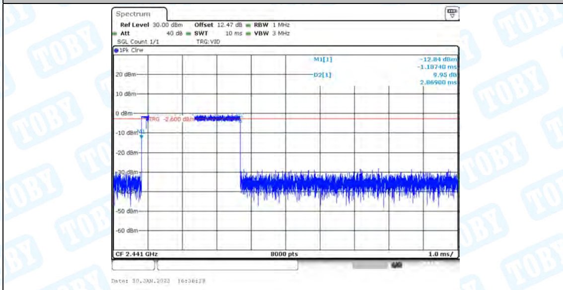
3DH5_AntA_Hop
