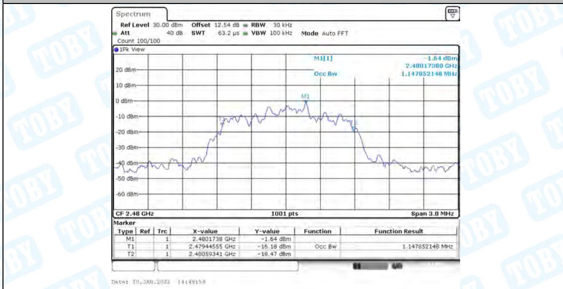
3DH5_AntA_2480
