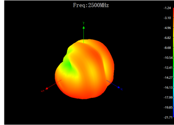
XYZ face @2500MHz
