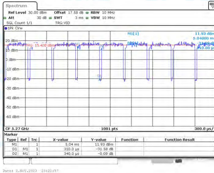
11AX40_Ant3_5270
