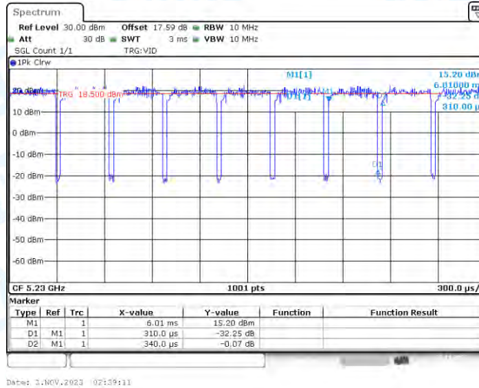
11AX40_Ant2_5230
