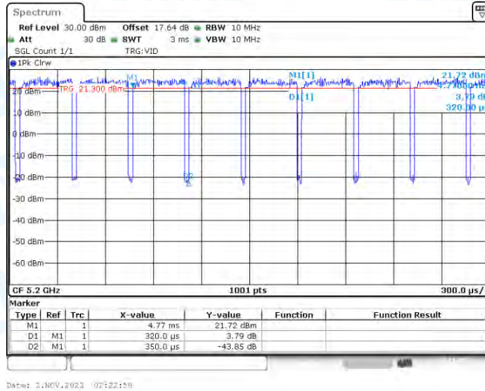
11AX20_Ant3_5200
