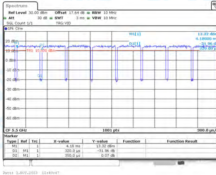
11AX20_Ant3_5500
