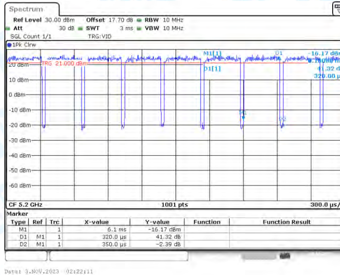
11AX20_Ant2_5200
