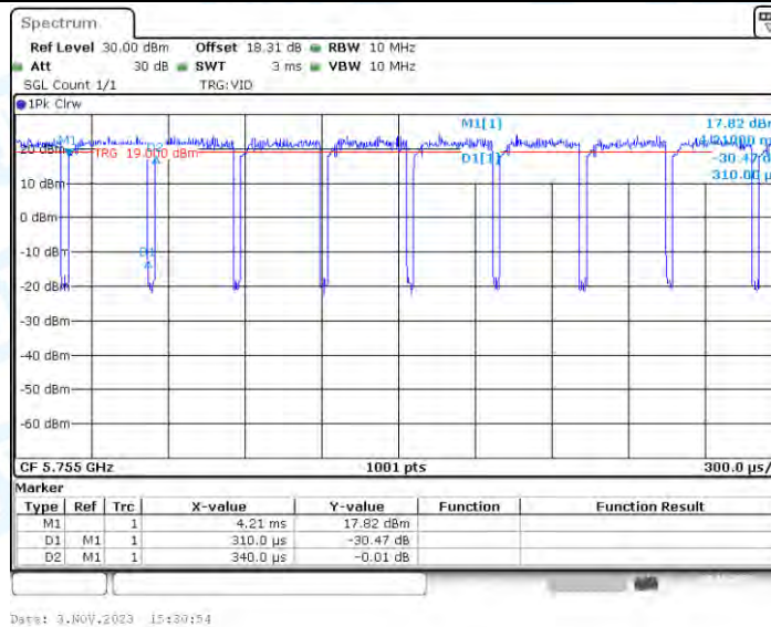
11AX40_Ant2_5755
