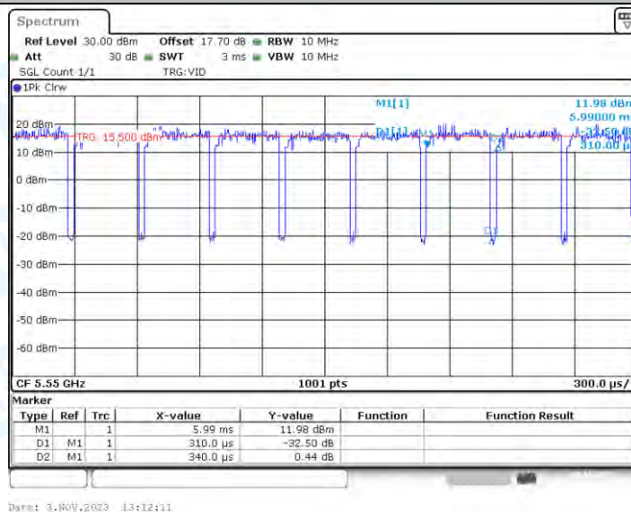
11AX40_Ant3_5550
