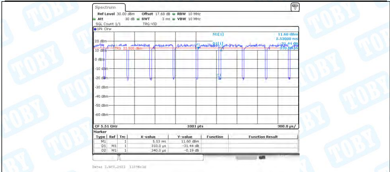
11AX40_Ant2_5510
