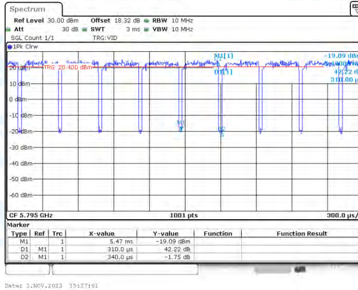
11AX40_Ant3_5795
