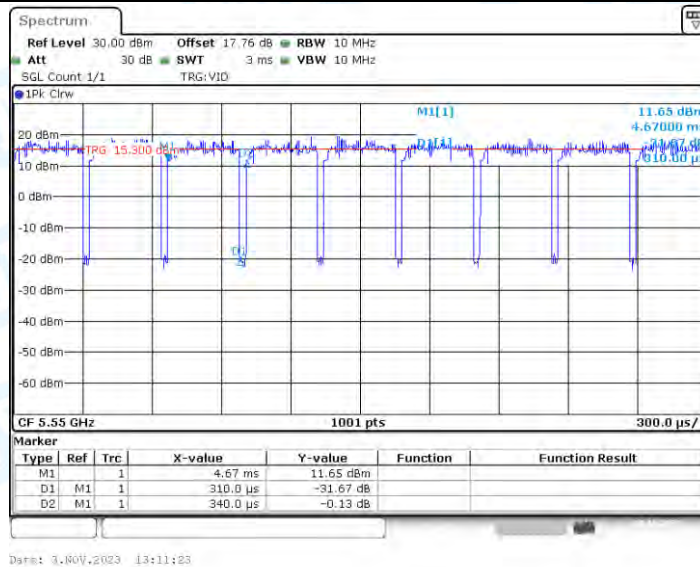
11AX40_Ant2_5550
