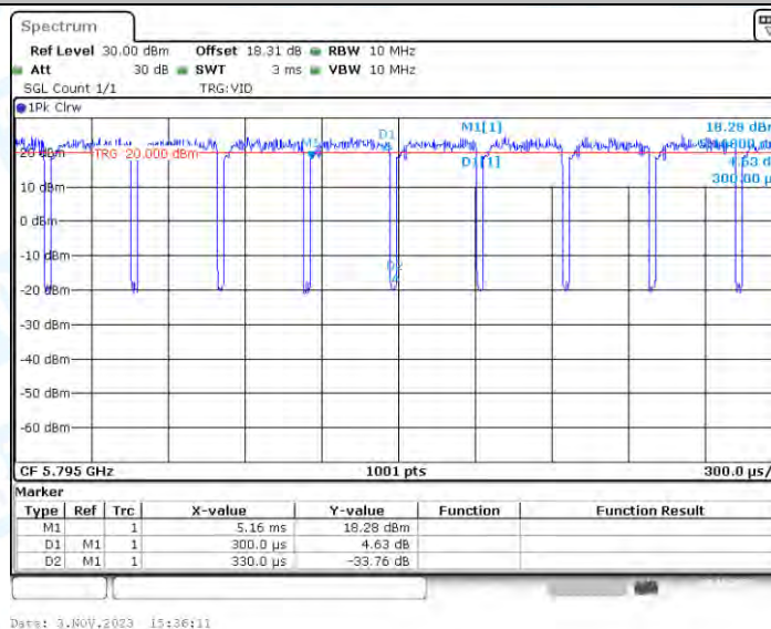
11AX40_Ant2_5795
