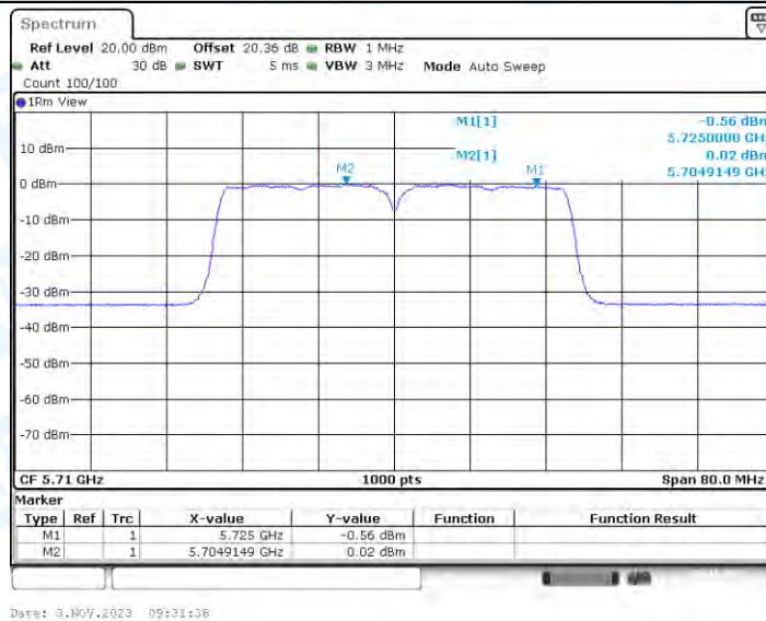
11N40-CDD_Ant3_5710_UNII-2C
