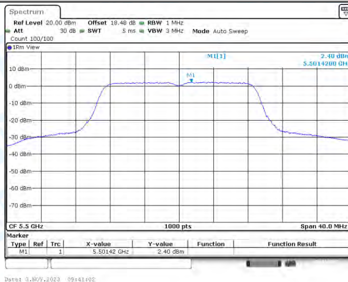
11AC20-CDD_Ant2_5500
