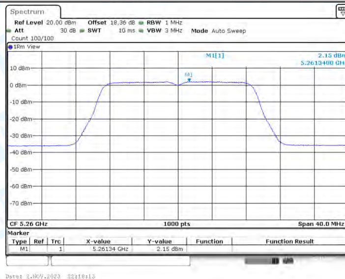
11AC20-CDD_Ant2_5260
