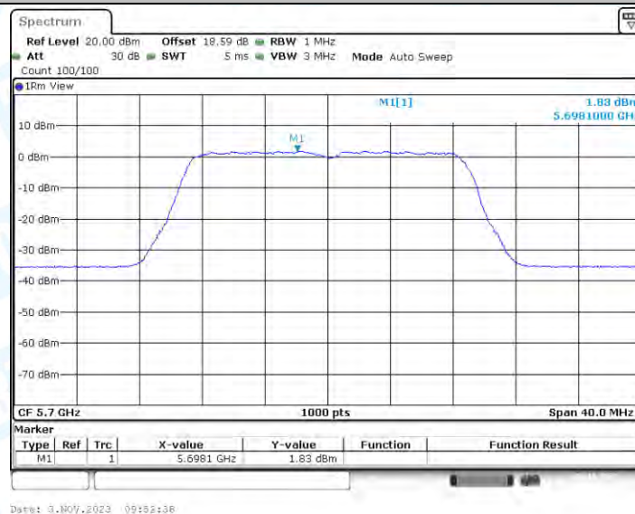
11AC20-CDD_Ant3_5700
