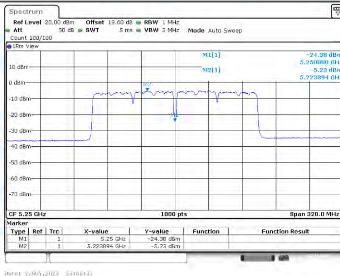
11AC160-CDD_Ant3_5250_UNII-1
