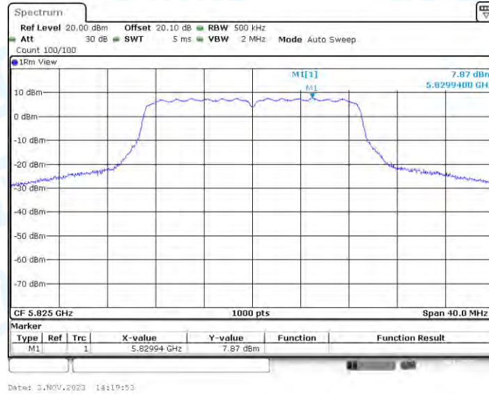
11N20-CDD_Ant3_5825
