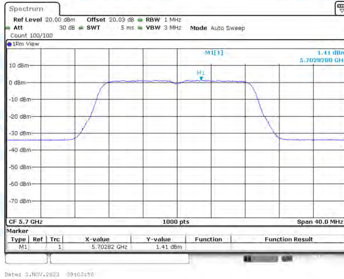
11N20-CDD_Ant2_5700
