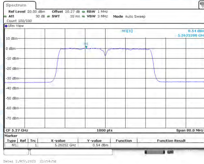
11N40-CDD_Ant4_5270
