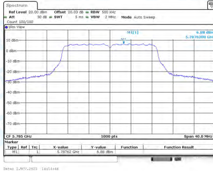
11N20-CDD_Ant2_5785
