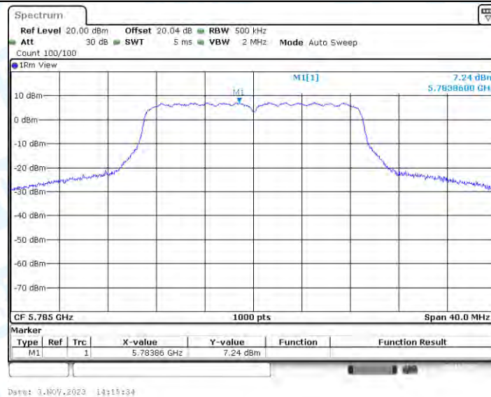
11N20-CDD_Ant3_5785
