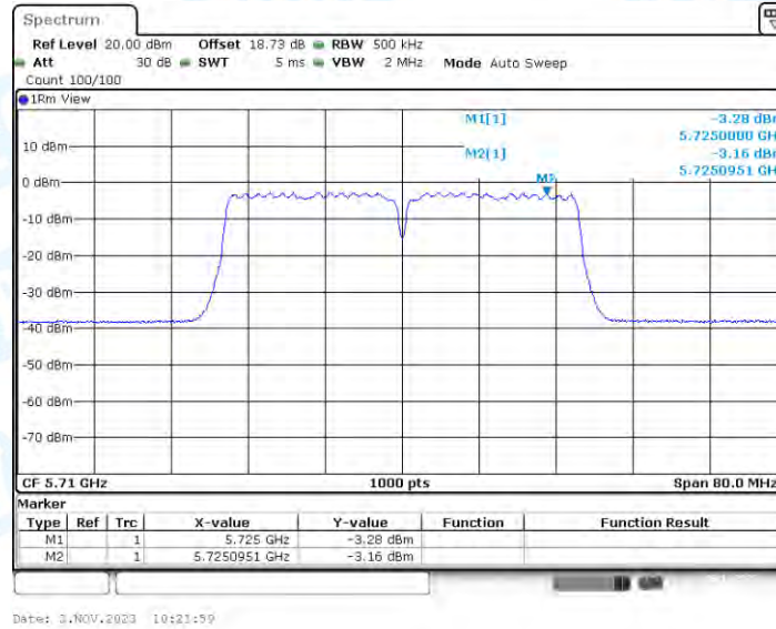
11AC40-CDD_Ant2_5710_UNII-3
