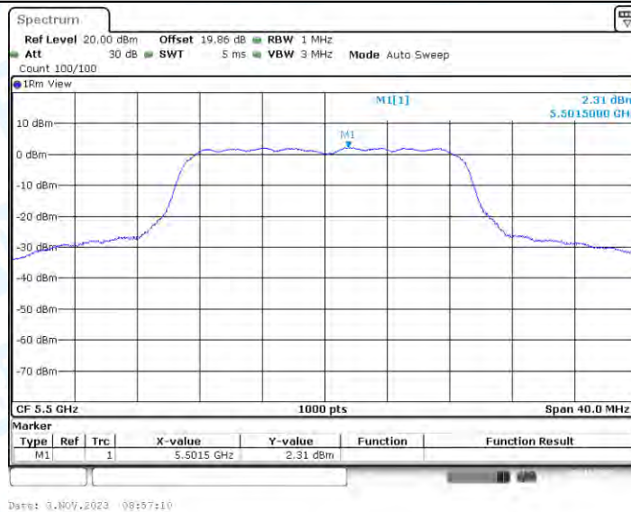
11N20-CDD_Ant3_5500
