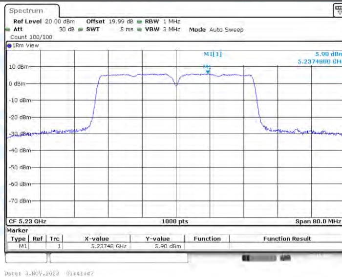
11N40-CDD_Ant3_5230
