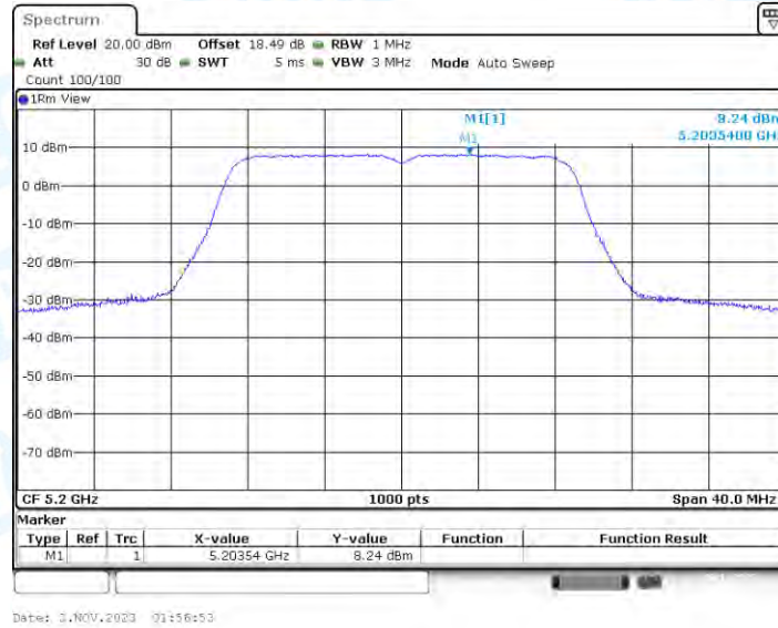
11AC20-CDD_Ant2_5200
