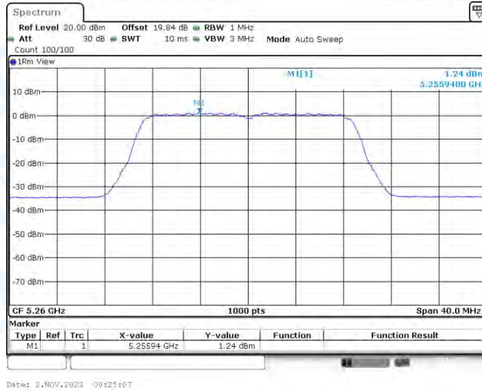
11N20-CDD_Ant4_5260
