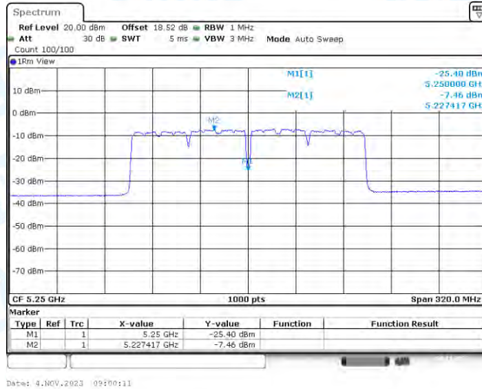
11AC160-BF_Ant3_5250_UNII-1
