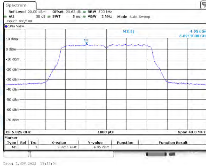
11N20-BF_Ant2_5825
