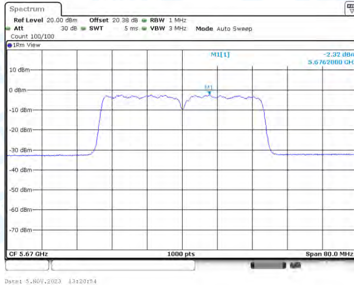
11N40-BF_Ant2_5670
