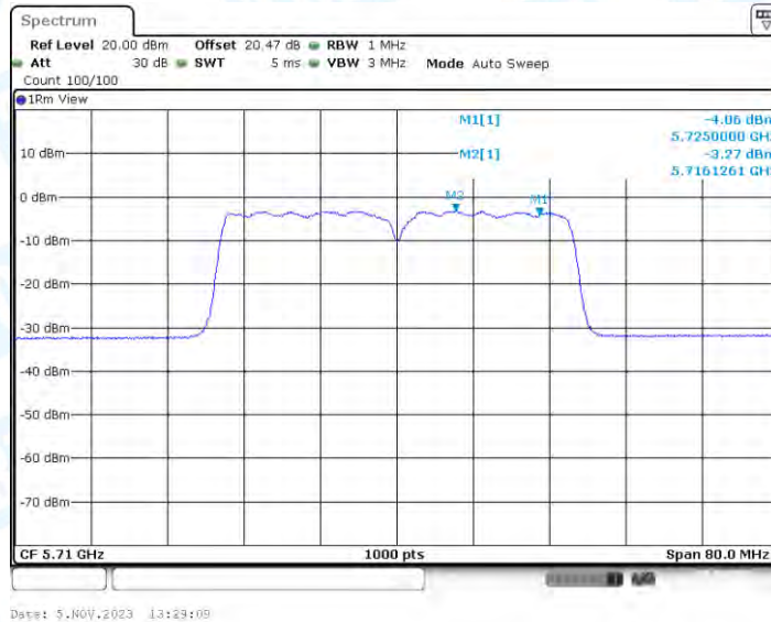
11N40-BF_Ant1_5710_UNII-3
