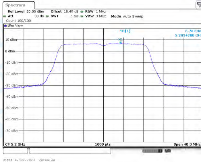
11AC20-BF_Ant2_5200
