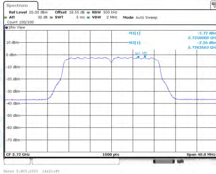
11AC20-BF_Ant2_5720_UNII-3
