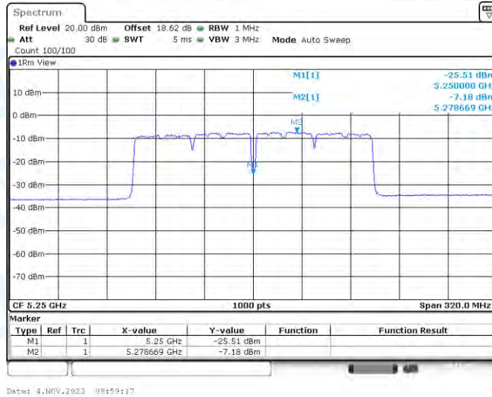
11AC160-BF_Ant2_5250_UNII-2A
