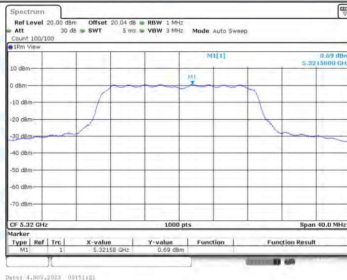
11N20-BF_Ant3_5320
