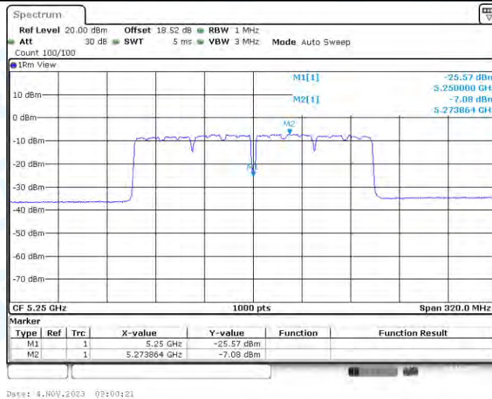
11AC160-BF_Ant3_5250_UNII-2A
