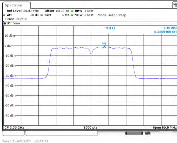
11N40-BF_Ant3_5550
