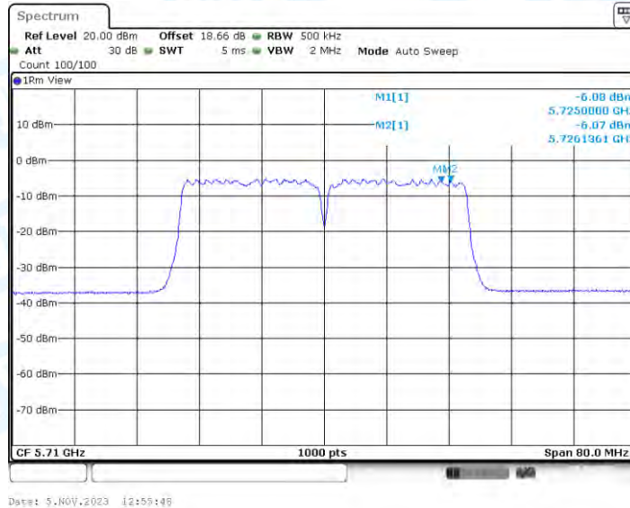
11AC40-BF_Ant2_5710_UNII-3
