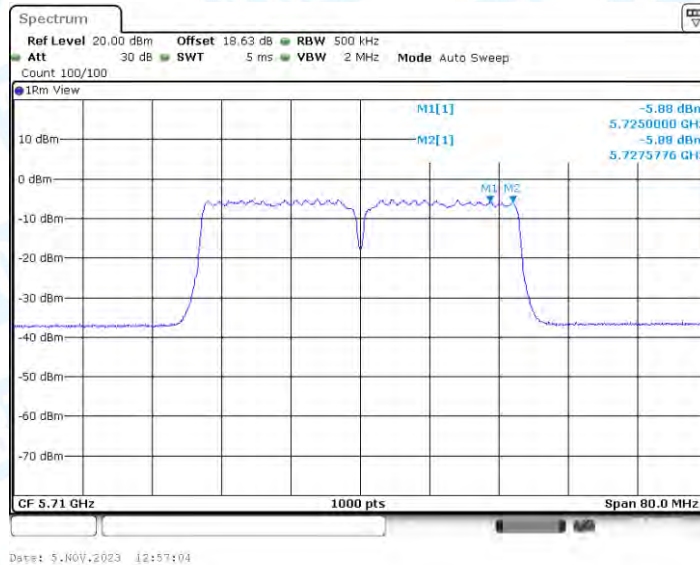
11AC40-BF_Ant3_5710_UNII-3
