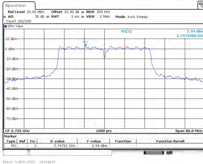
11N40-BF_Ant3_5755
