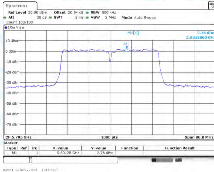
11N40-BF_Ant2_5795
