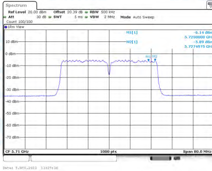
11N40-BF_Ant2_5710_UNII-3
