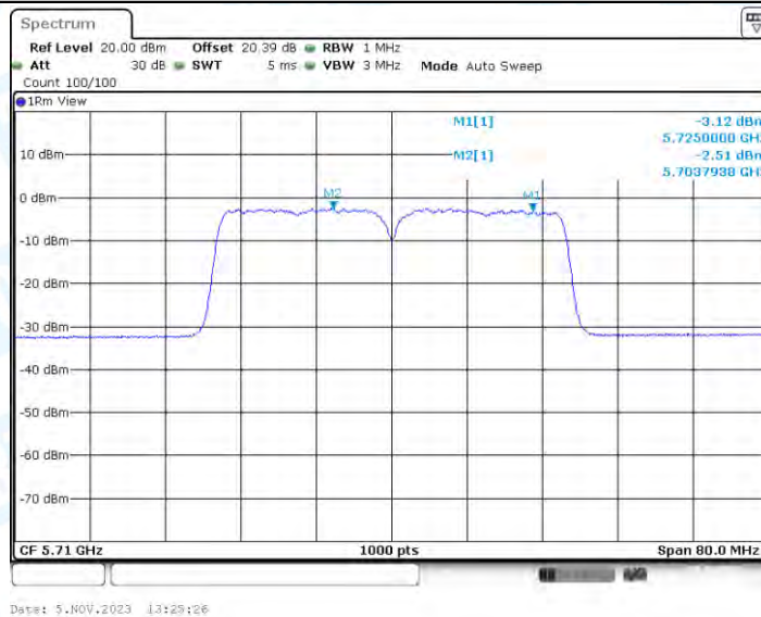
11N40-BF_Ant2_5710_UNII-2C
