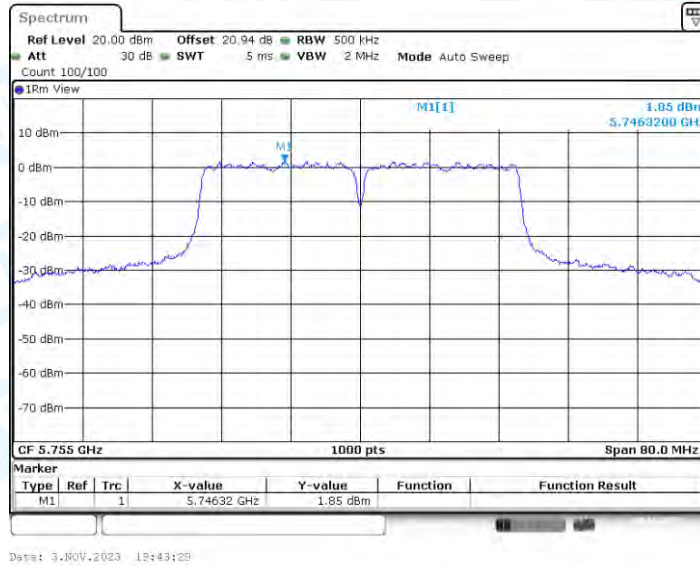
11N40-BF_Ant2_5755
