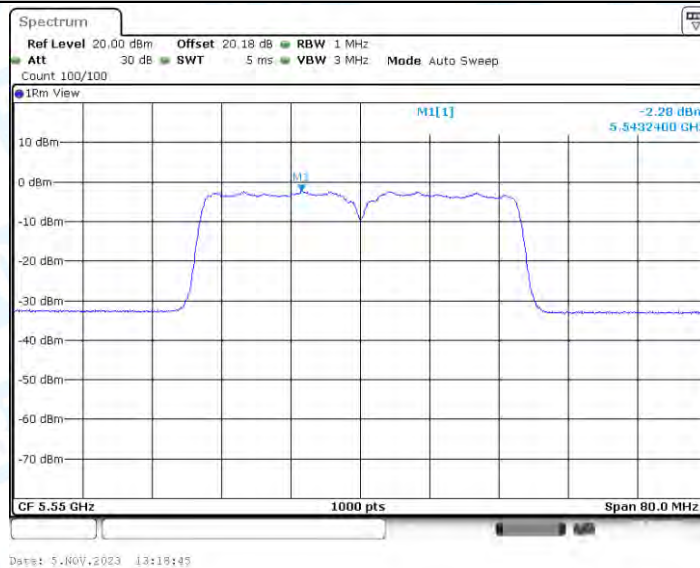
11N40-BF_Ant4_5550
