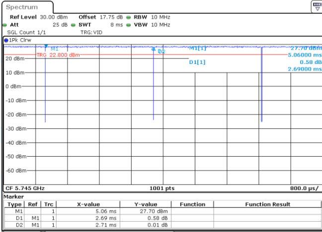
NTNV-11A-Ant1-5745
