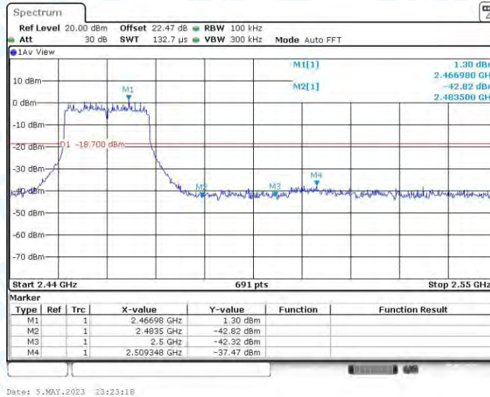
11AX20MIMO_Ant2_High_2462
