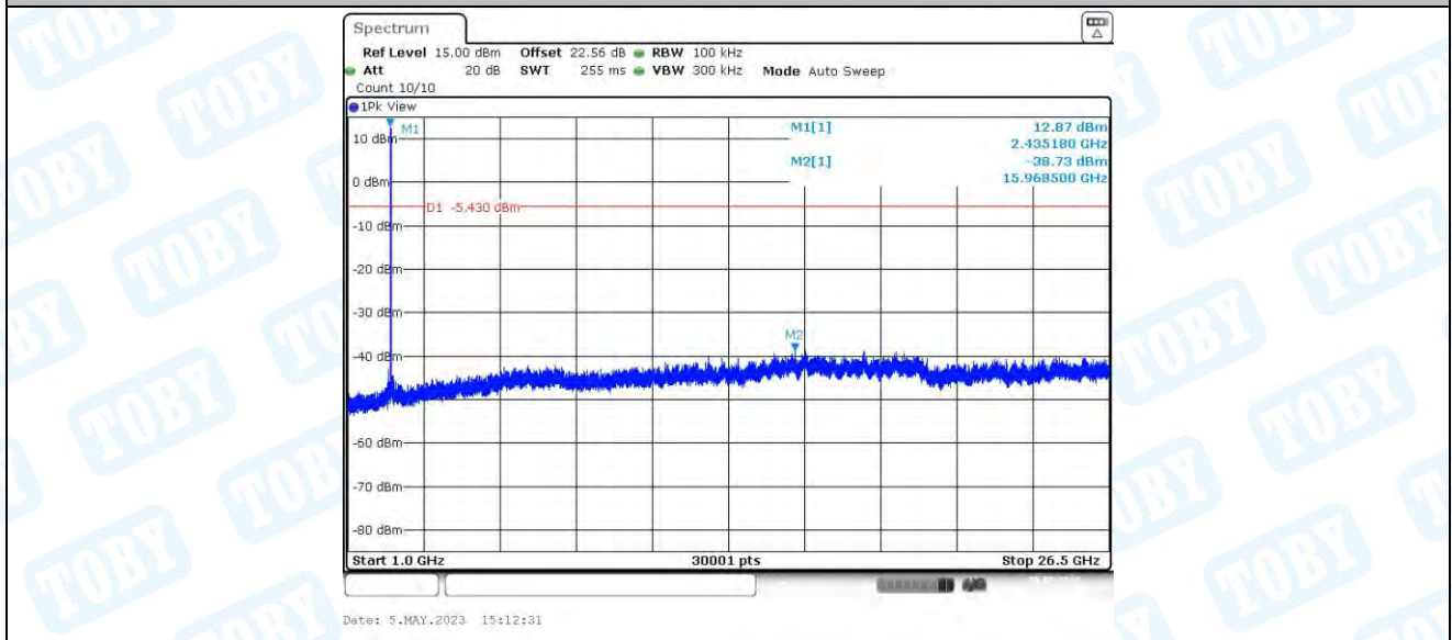
11B_Ant2_2437_0~Reference
