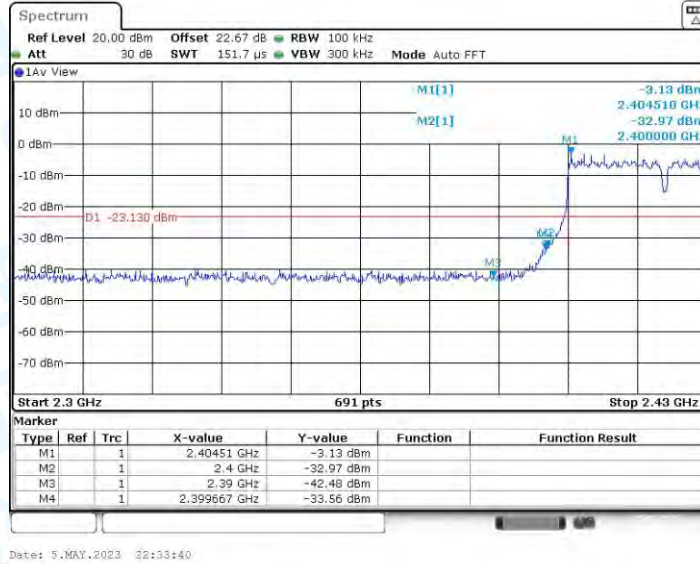
11N40MIMO_Ant3_Low_2422
