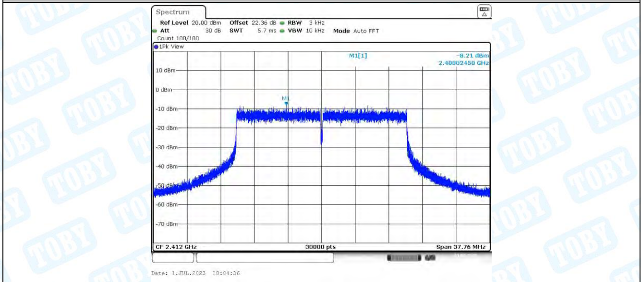
11AX20MIMO_Ant3_2412
