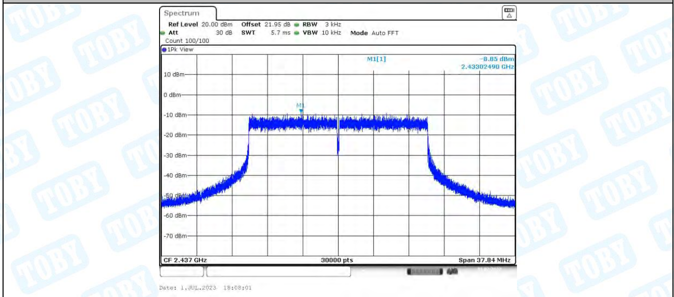
11AX20MIMO_Ant3_2437
