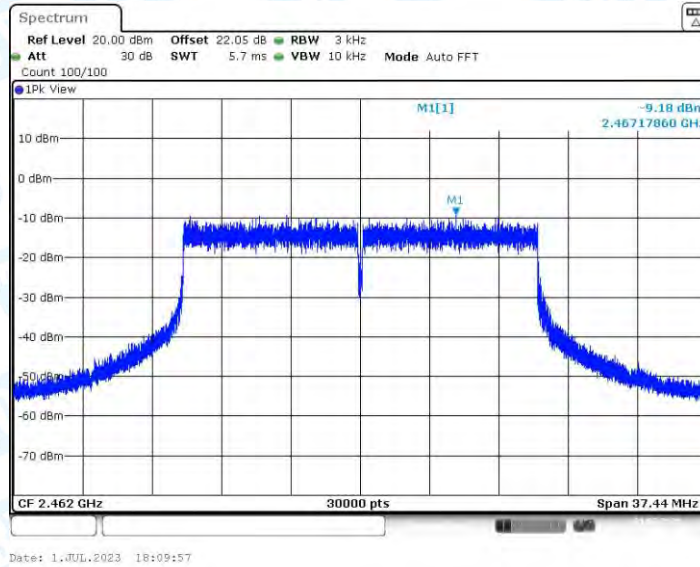
11AX20MIMO_Ant3_2462
