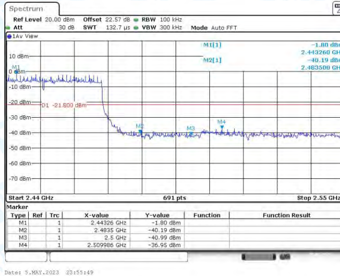
11AX40MIMO_Ant3_High_2452
