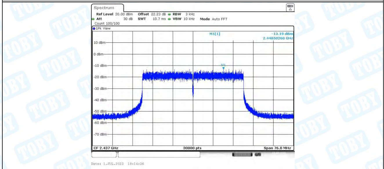
11AX40MIMO_Ant2_2437
