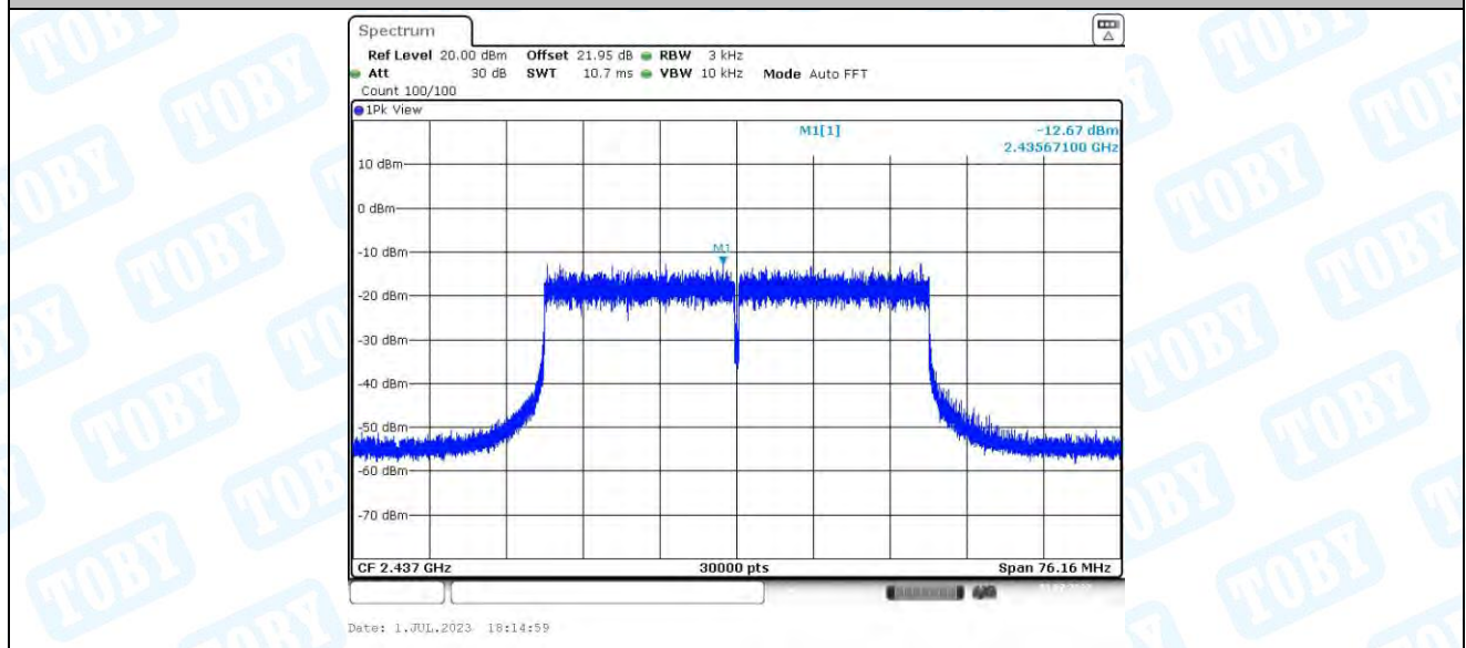
11AX40MIMO_Ant3_2437
