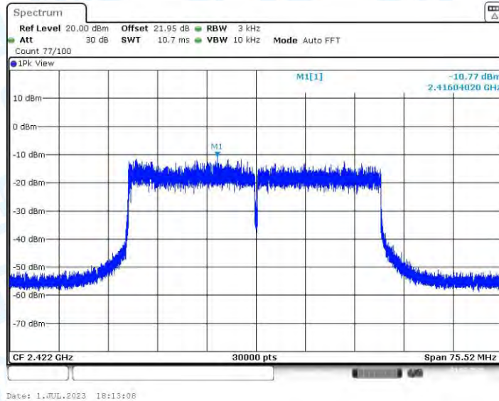
11AX40MIMO_Ant3_2422
