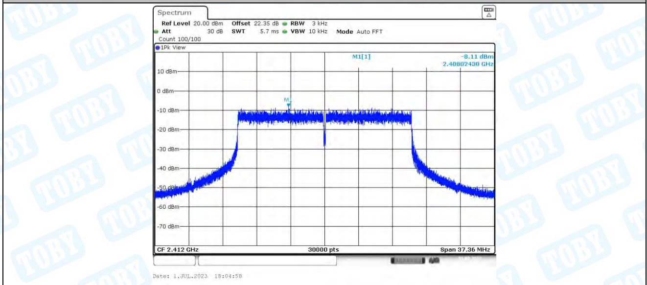
11AX20MIMO_Ant4_2412
