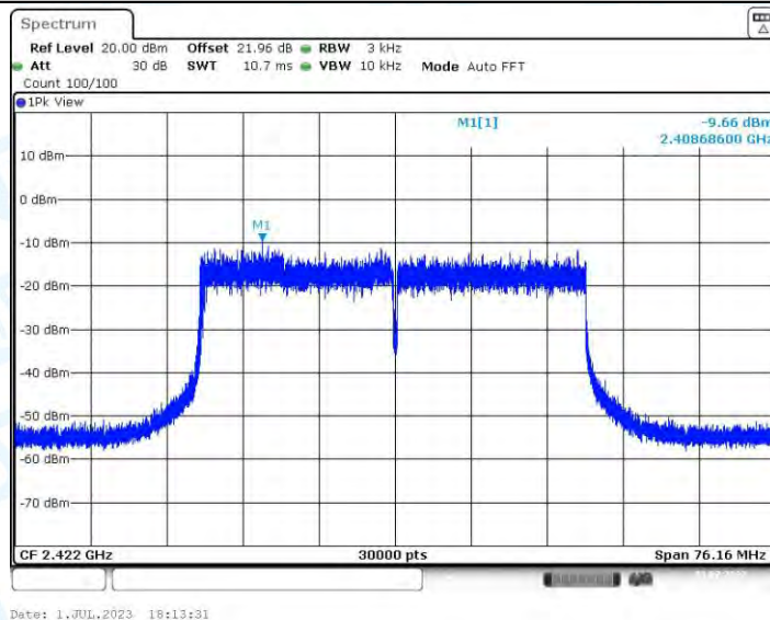
11AX40MIMO_Ant4_2422
