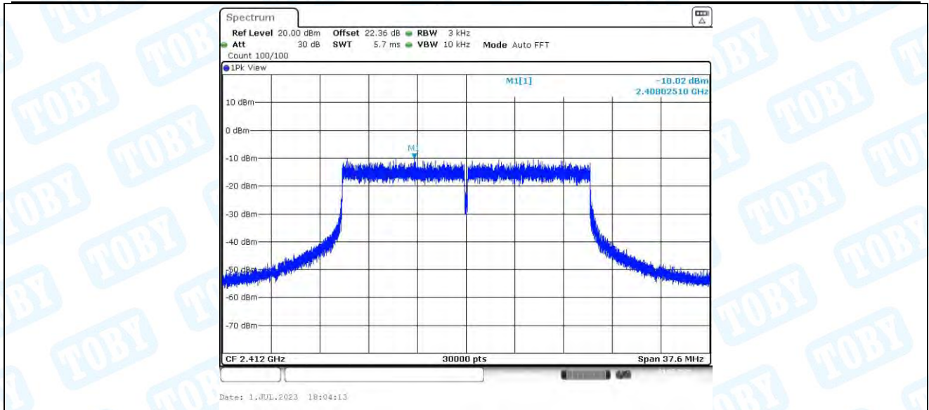
11AX20MIMO_Ant2_2412
