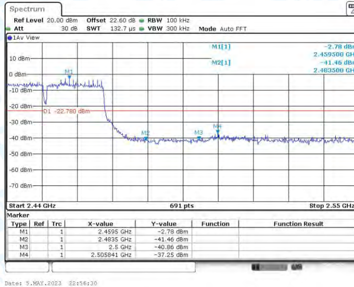
11N40MIMO_Ant4_High_2452
