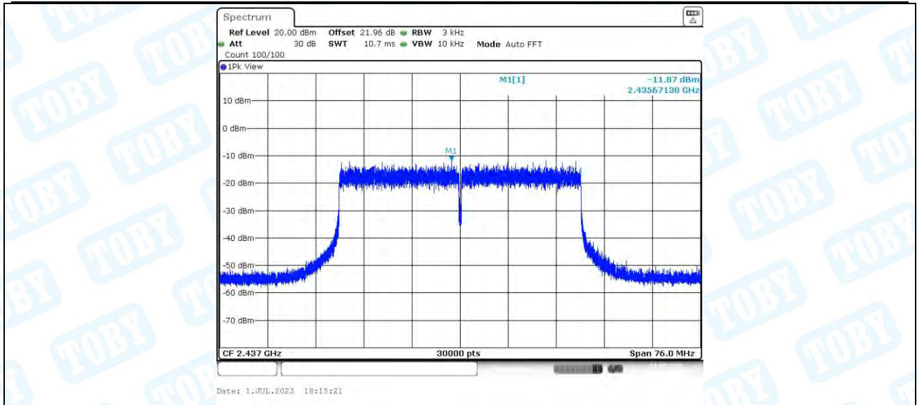
11AX40MIMO_Ant4_2437
