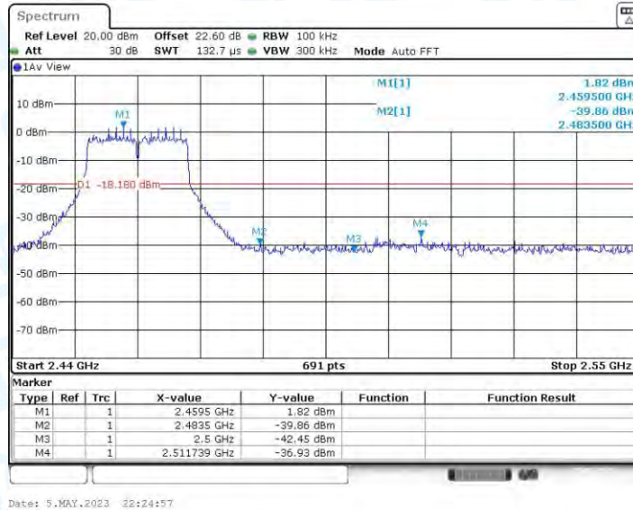
11N20MIMO_Ant4_High_2462
