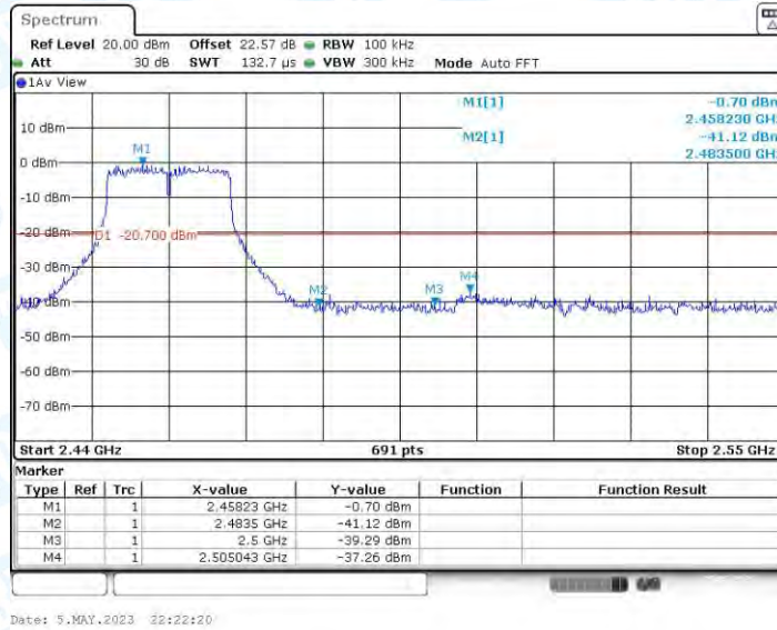
11N20MIMO_Ant3_High_2462
