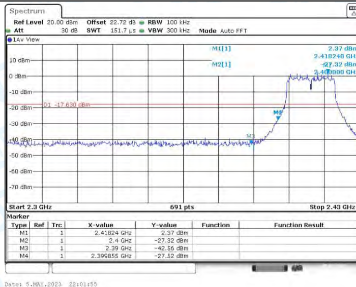
11N20MIMO_Ant3_Low_2412
