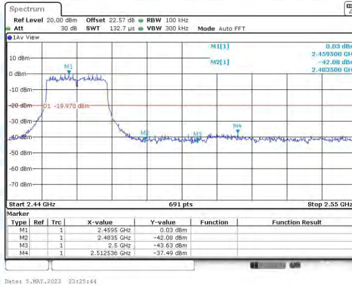
11AX20MIMO_Ant3_High_2462
