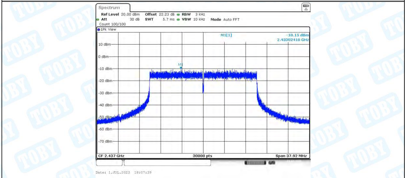
11AX20MIMO_Ant2_2437
