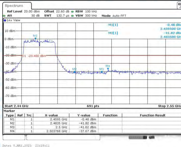
11AX20MIMO_Ant4_High_2462
