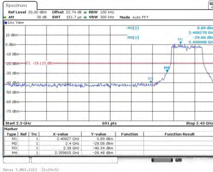
11AX20MIMO_Ant4_Low_2412
