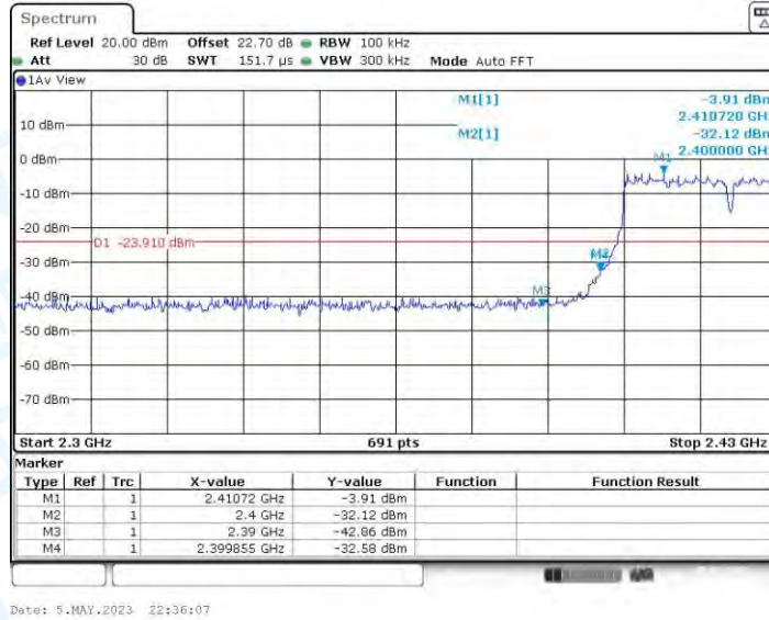
11N40MIMO_Ant4_Low_2422
