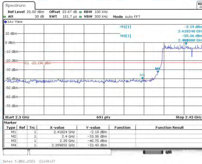
11AX40MIMO_Ant3_Low_2422
