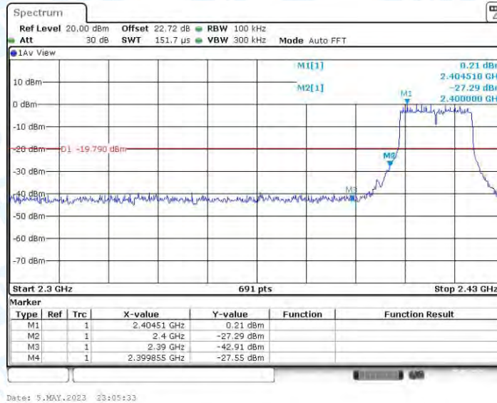
11AX20MIMO_Ant3_Low_2412
