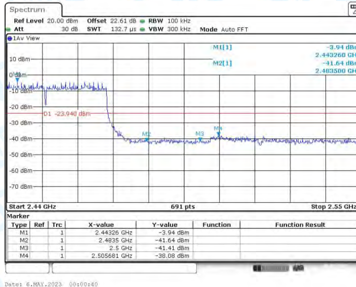
11AX40MIMO_Ant4_High_2452
