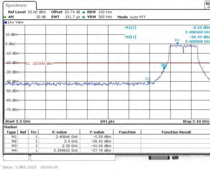
11N20MIMO_Ant4_Low_2412
