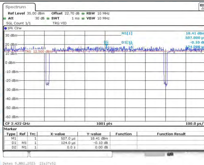
11AX40MIMO_Ant4_2422
