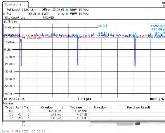
11AX20MIMO_Ant4_2412
