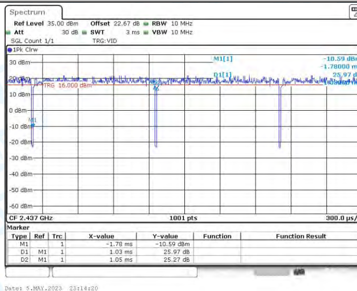
11AX20MIMO_Ant3_2437
