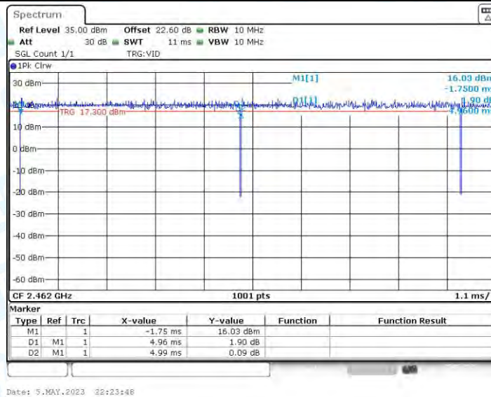
11N20MIMO_Ant4_2462
