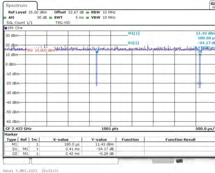
11N40MIMO_Ant3_2422
