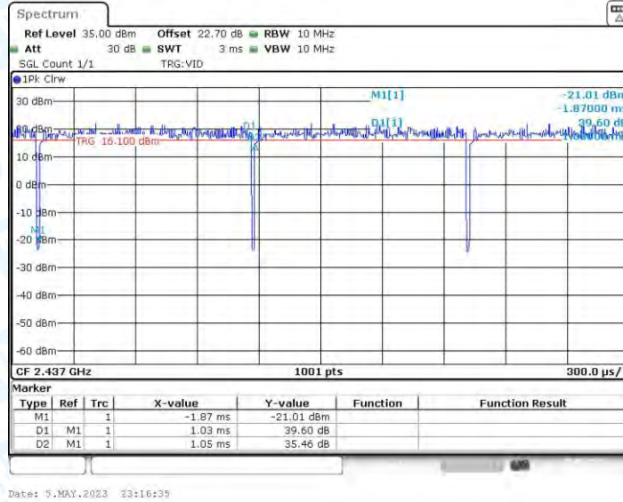
11AX20MIMO_Ant4_2437
