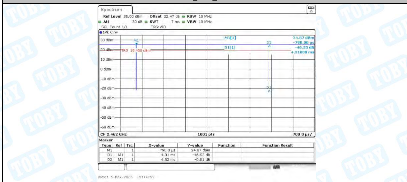
11B_Ant2_2462
