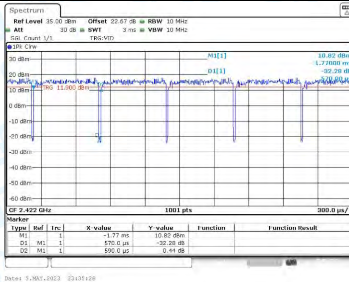
11AX40MIMO_Ant3_2422
