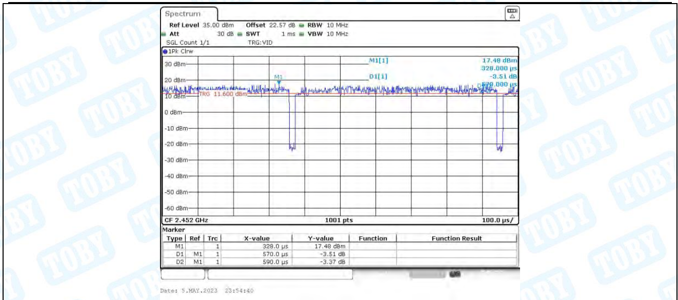
11AX40MIMO_Ant3_2452
