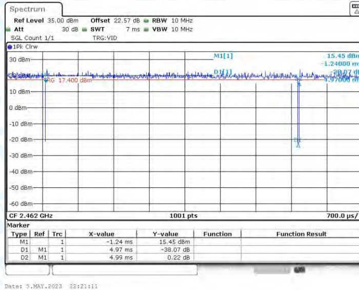
11N20MIMO_Ant3_2462
