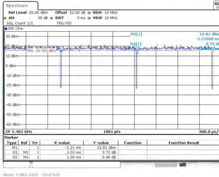
11AX20MIMO_Ant4_2462
