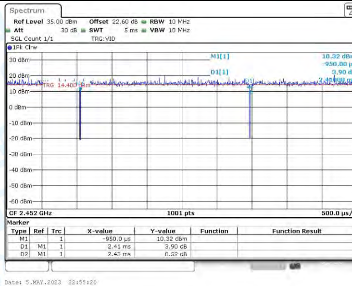
11N40MIMO_Ant4_2452
