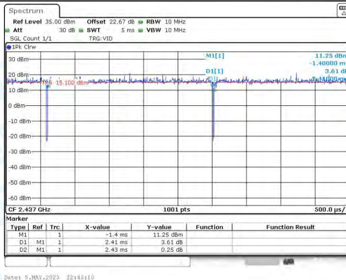
11N40MIMO_Ant3_2437
