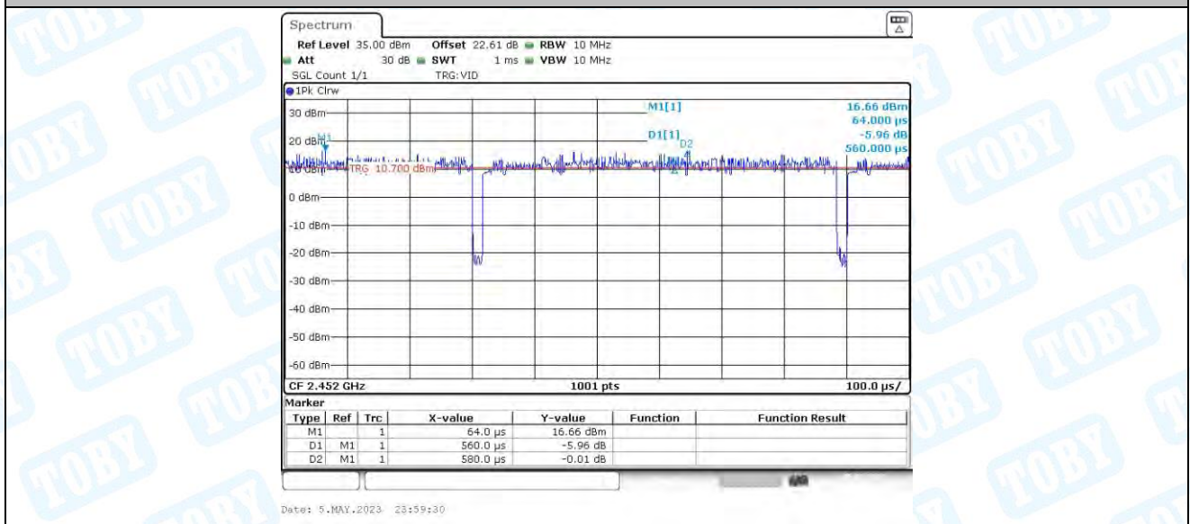
11AX40MIMO_Ant4_2452
