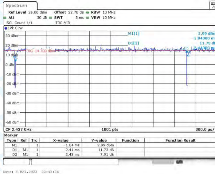
11N40MIMO_Ant4_2437
