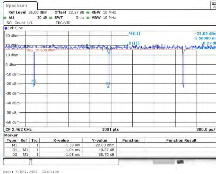
11AX20MIMO_Ant3_2462
