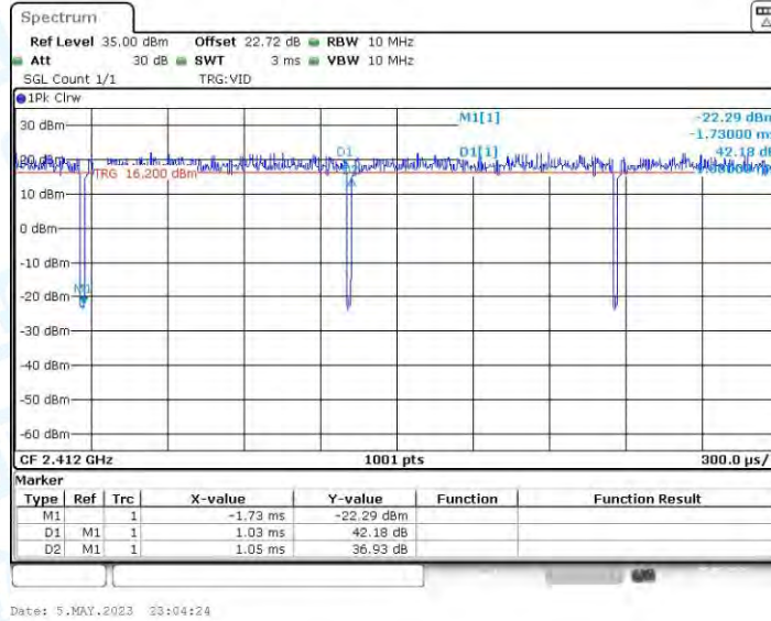
11AX20MIMO_Ant3_2412
