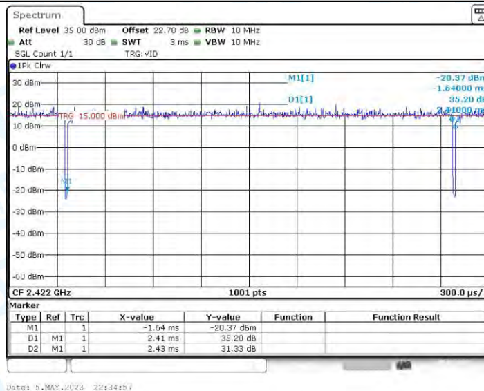
11N40MIMO_Ant4_2422
