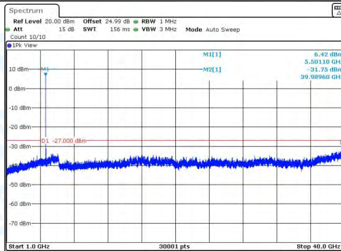
11AC20MIMO_Ant1_5500_1000~40000
