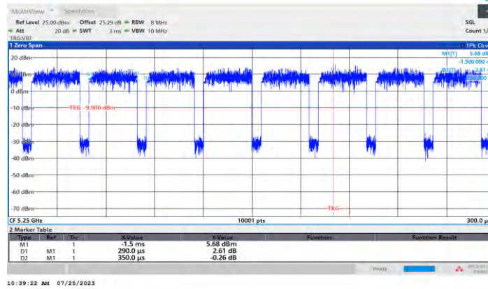
11AX160MIMO_Ant0_5250
