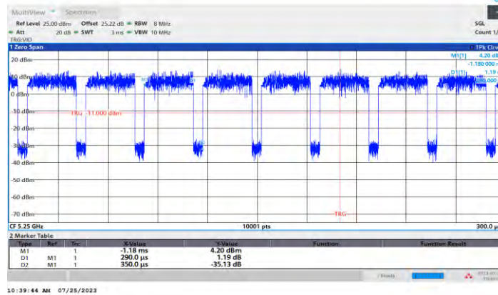
11AX160MIMO_Ant1_5250
