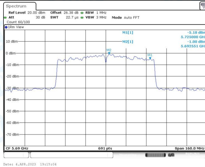
11AC80MIMO_Ant2_5690_UNII-2C
