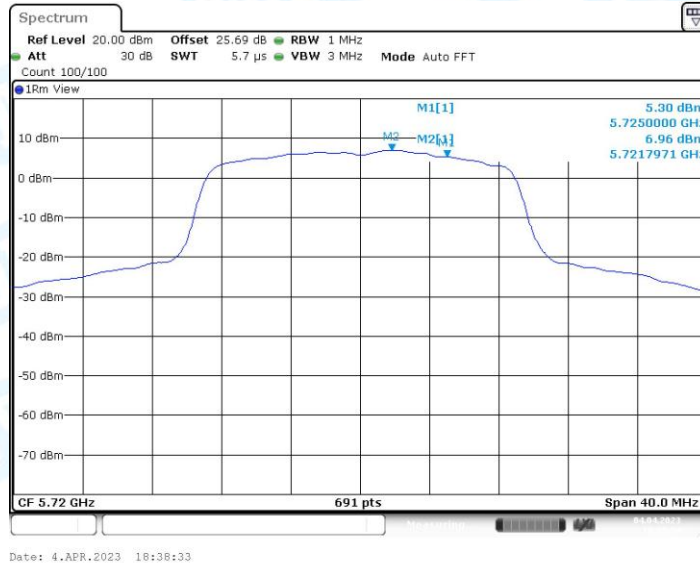
11AC20MIMO_Ant2_5720_UNII-2C
