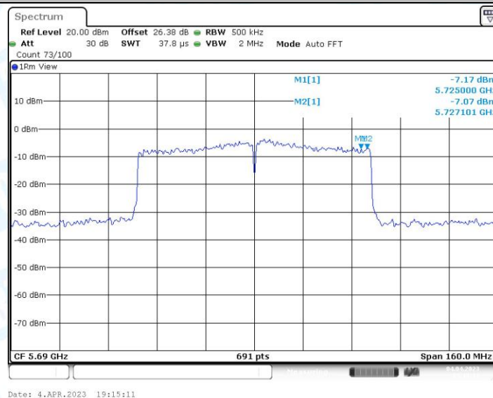
11AC80MIMO_Ant2_5690_UNII-3
