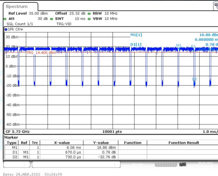
11N20MIMO_Ant2_5720
