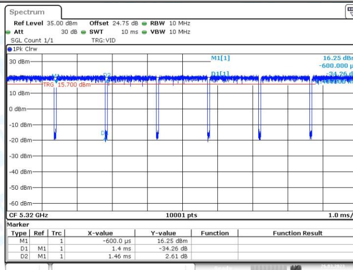
11A_Ant2_5320
