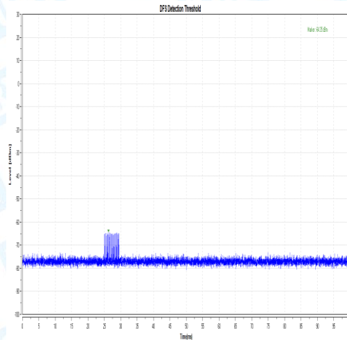
11AC40-5270-Type2
