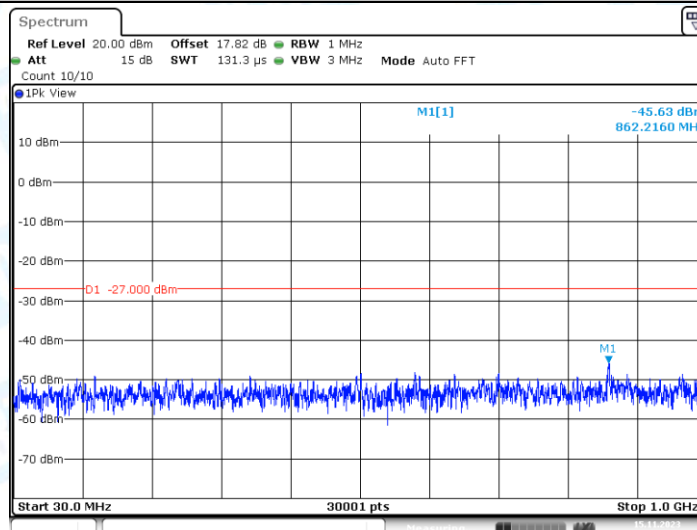
11N20MIMO_Ant2_5785_30~1000
