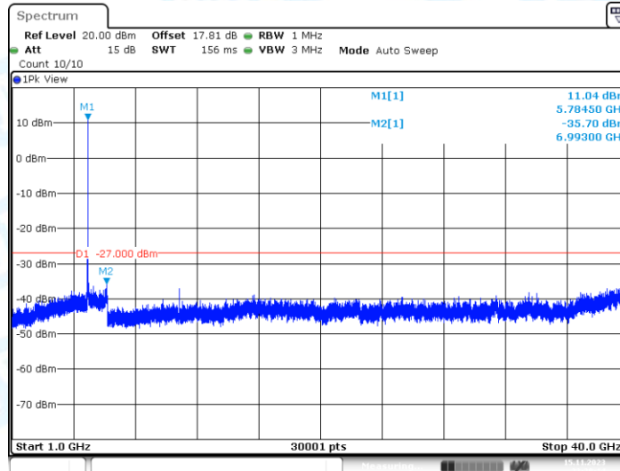
11N20MIMO_Ant1_5785_1000~40000
