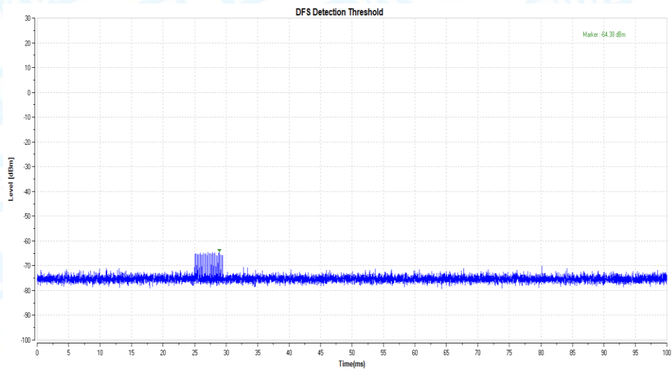
11N40_5270_Type3
