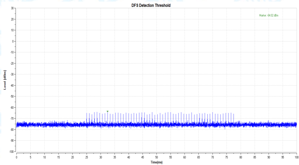
11N40_5510_Type2
