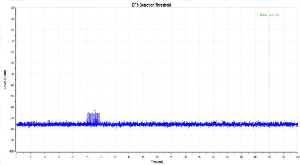
11A_5500_Type3
