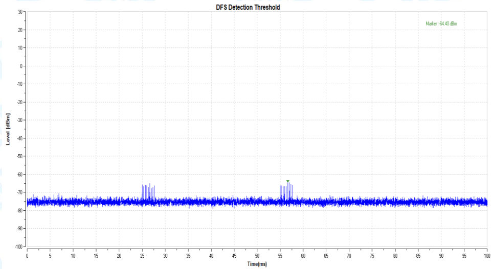
11A_5500_Type0
