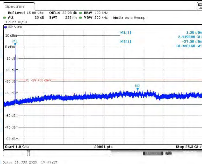
11N40-CDD_Ant2_2422_0~Reference
