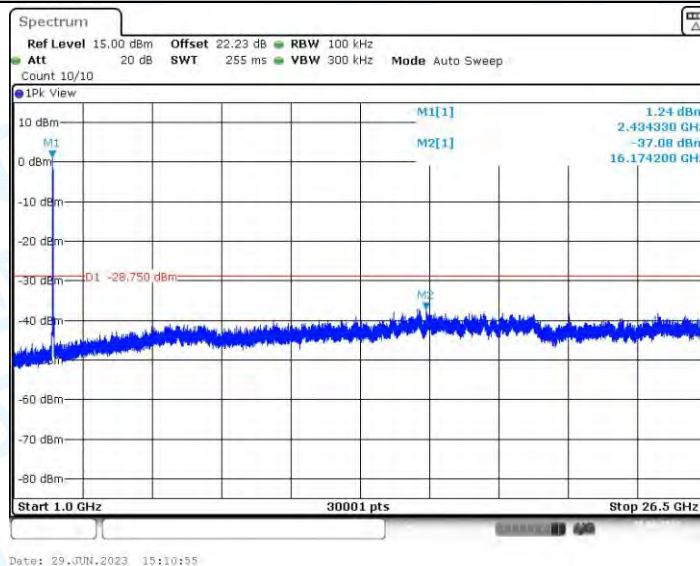
11N40-CDD_Ant2_2437_0~Reference
