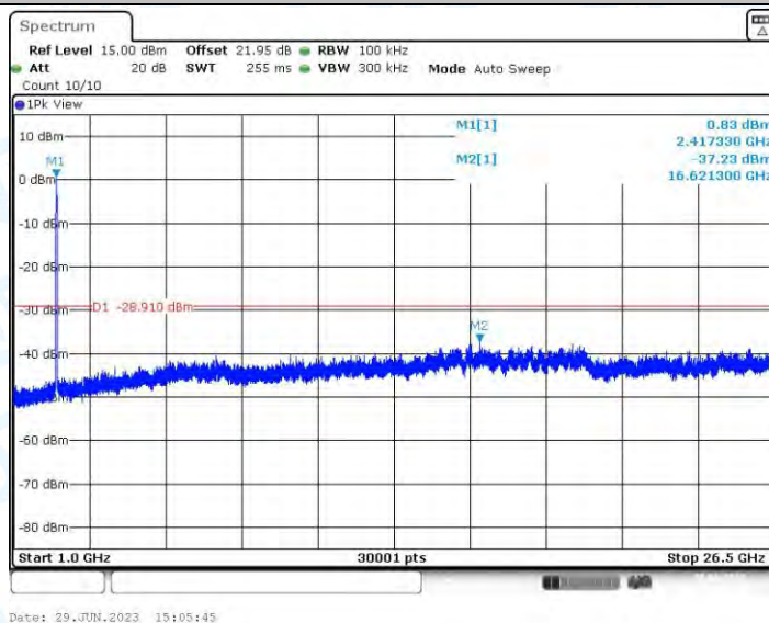
11N40-CDD_Ant1_2437_0~Reference
