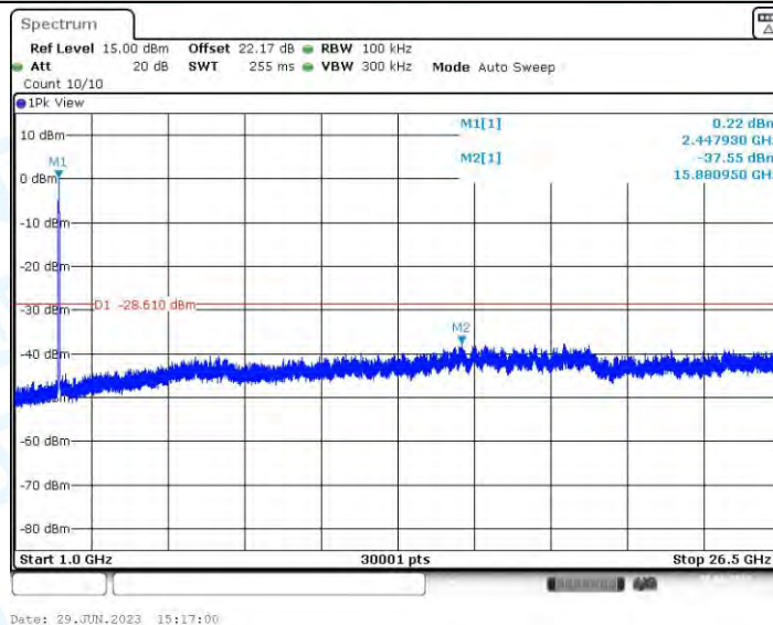
11N40-CDD_Ant2_2452_0~Reference
