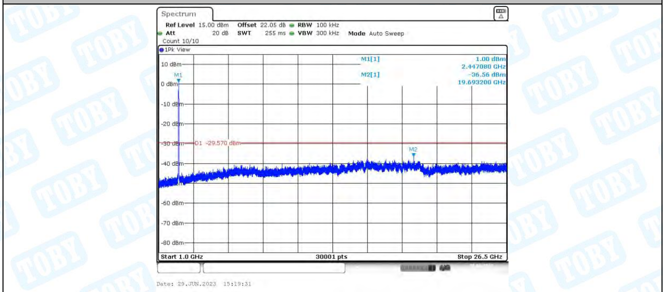
11N40-CDD_Ant2_2452_1000~26500
