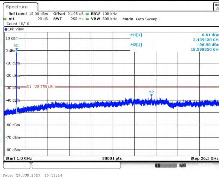
11N40-CDD_Ant1_2452_0~Reference
