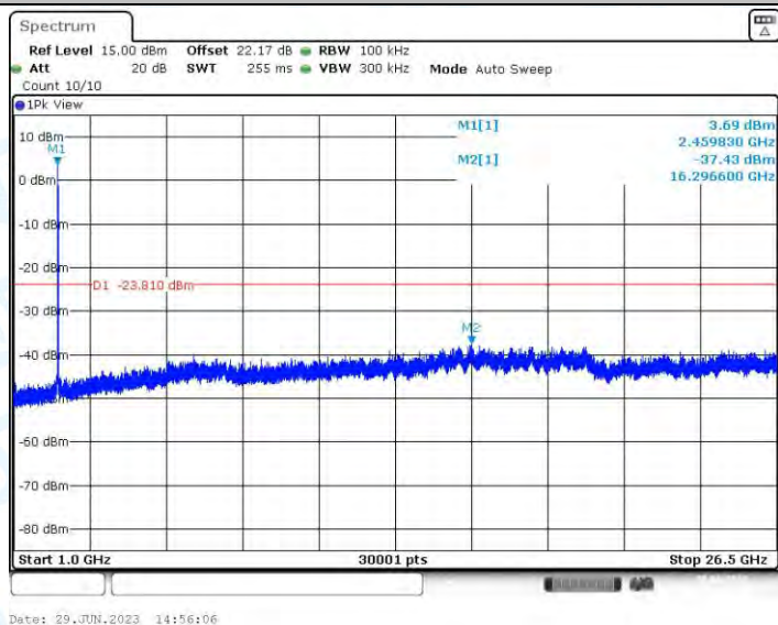
11N20-CDD_Ant2_2462_0~Reference
