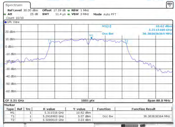
11N40-CDD-Ant1-5310
