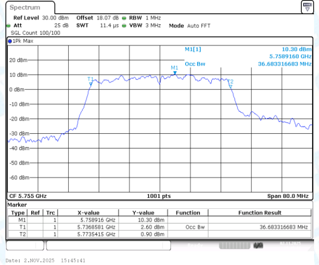
11N40-CDD-Ant1-5755
