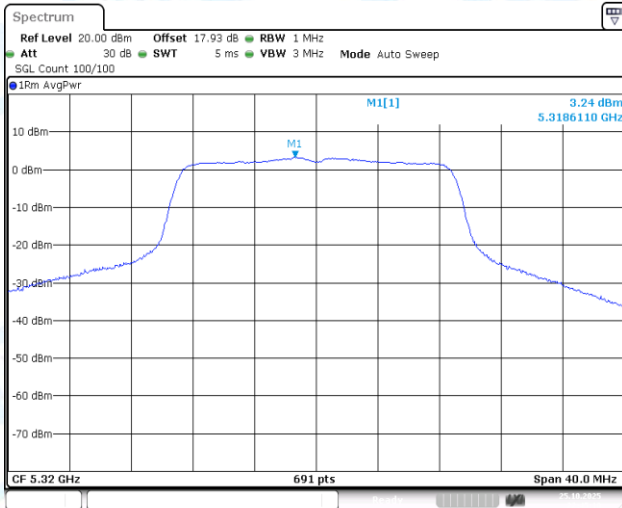
11N20-CDD-Ant1-5320-PASS
