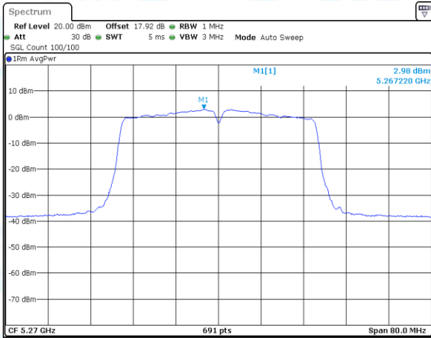
11N40-CDD-Ant1-5270-PASS
