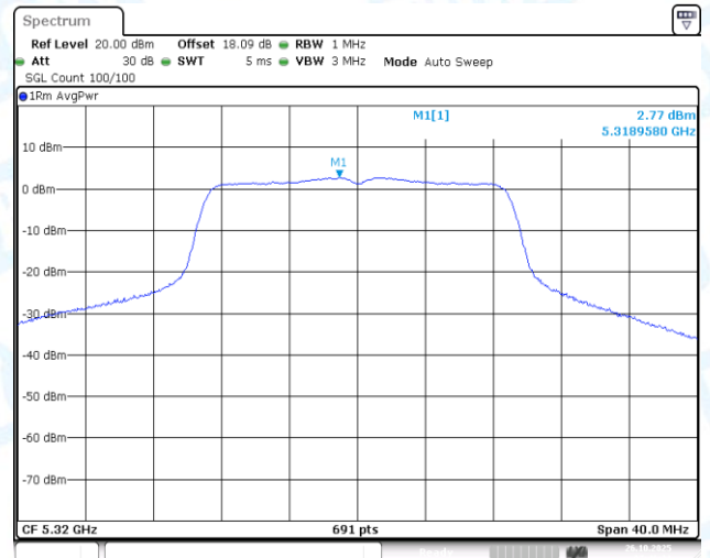
11AC20-CDD-Ant1-5320-PASS
