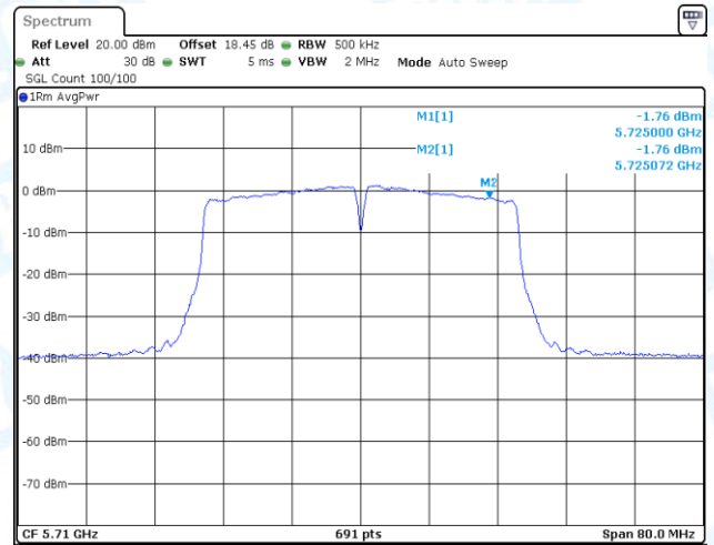
11N40-CDD-Ant1-5710_UNII-3-PASS
