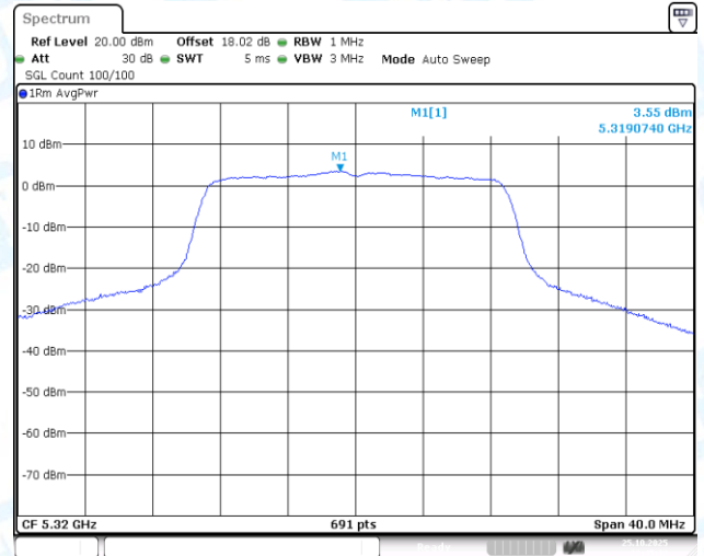
11N20-CDD-Ant2-5320-PASS
