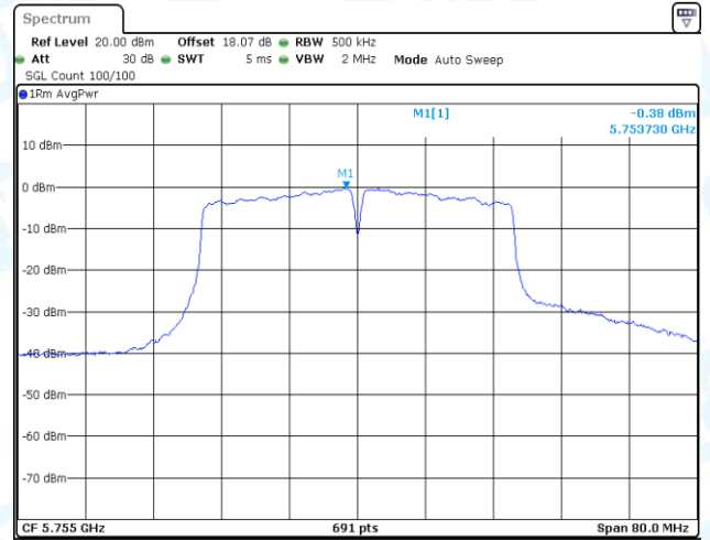
11N40-CDD-Ant2-5755-PASS
