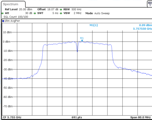
11N40-CDD-Ant1-5755-PASS
