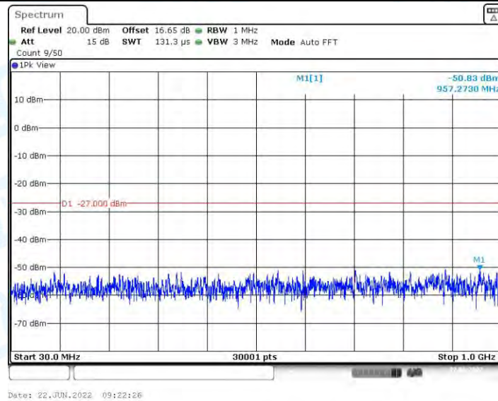
11N20MIMO_Ant1_5745_30~1000
