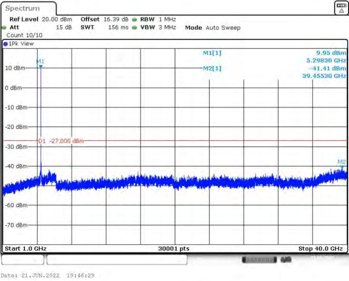
11N20MIMO_Ant2_5300_1000~40000
