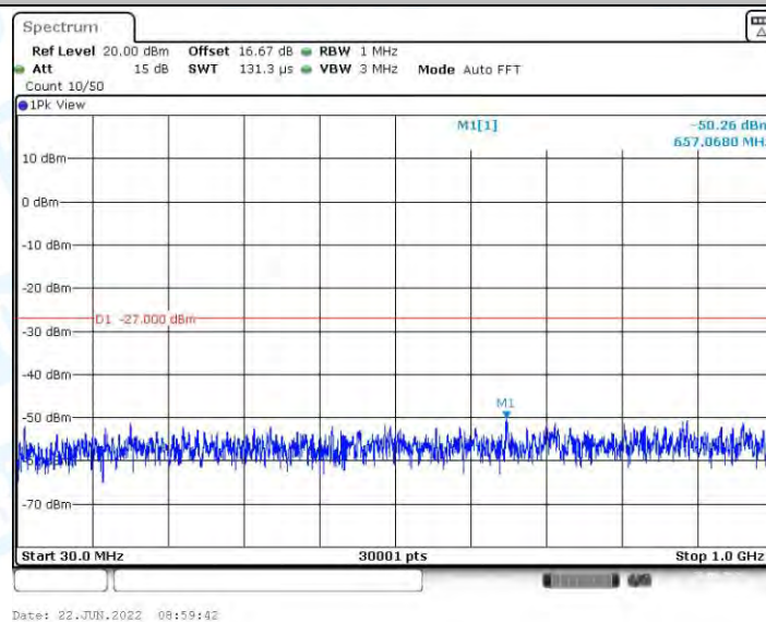
11N20MIMO_Ant2_5500_30~1000
