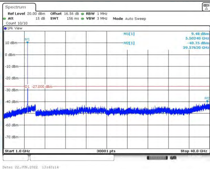
11AC20MIMO_Ant1_5500_1000~40000
