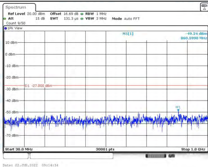
11N20MIMO_Ant1_5700_30~1000
