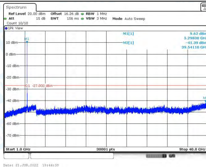
11N20MIMO_Ant1_5300_1000~40000
