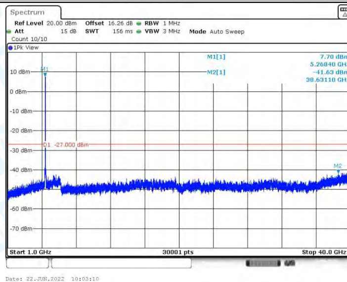
11N40MIMO_Ant2_5270_1000~40000
