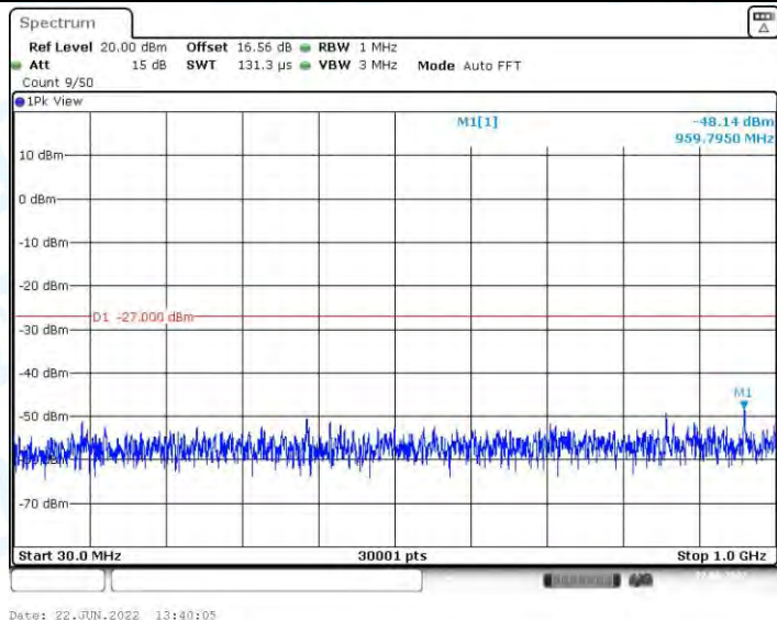
11AC20MIMO_Ant1_5500_30~1000
