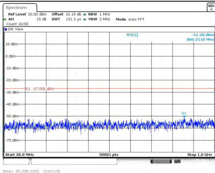
11N40MIMO_Ant1_5270_30~1000
