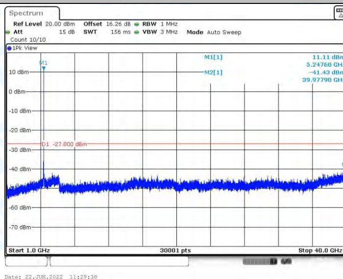
11AC20MIMO_Ant2_5240_1000~40000
