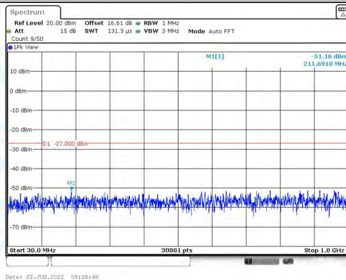
11N20MIMO_Ant2_5745_30~1000
