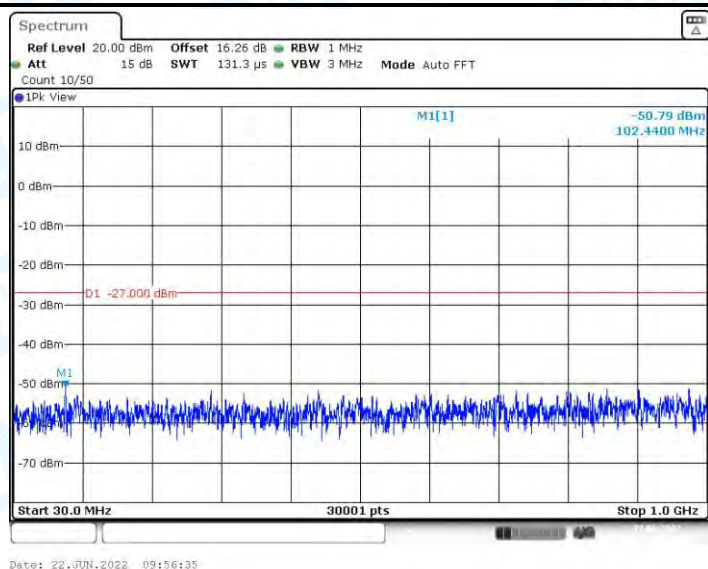
11N40MIMO_Ant2_5230_30~1000
