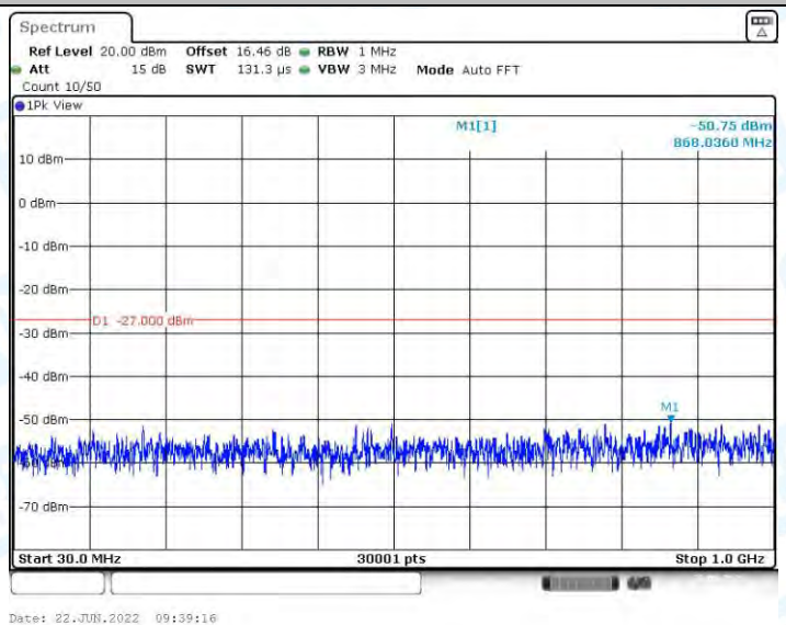
11N20MIMO_Ant1_5825_30~1000
