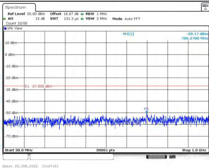
11AC20MIMO_Ant2_5500_30~1000
