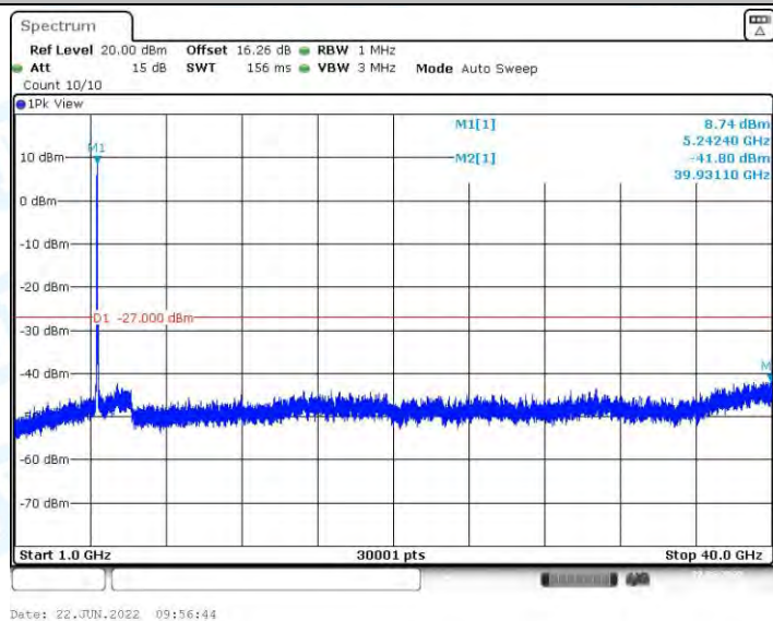
11N40MIMO_Ant2_5230_1000~40000
