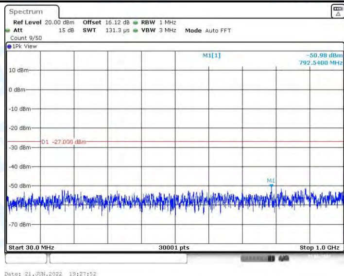
11N20MIMO_Ant2_5220_30~1000
