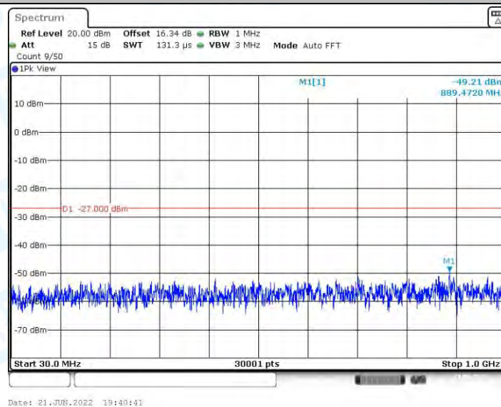
11N20MIMO_Ant2_5260_30~1000
