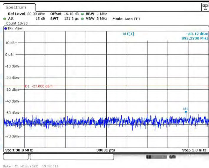
11N20MIMO_Ant1_5240_30~1000
