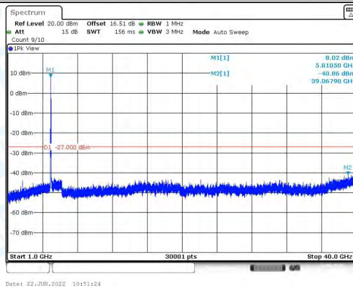
11N40MIMO_Ant2_5795_1000~40000
