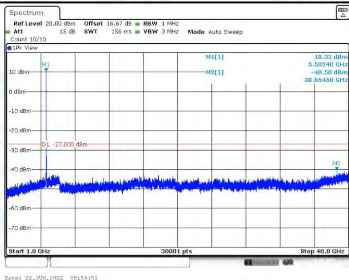
11N20MIMO_Ant2_5500_1000~40000
