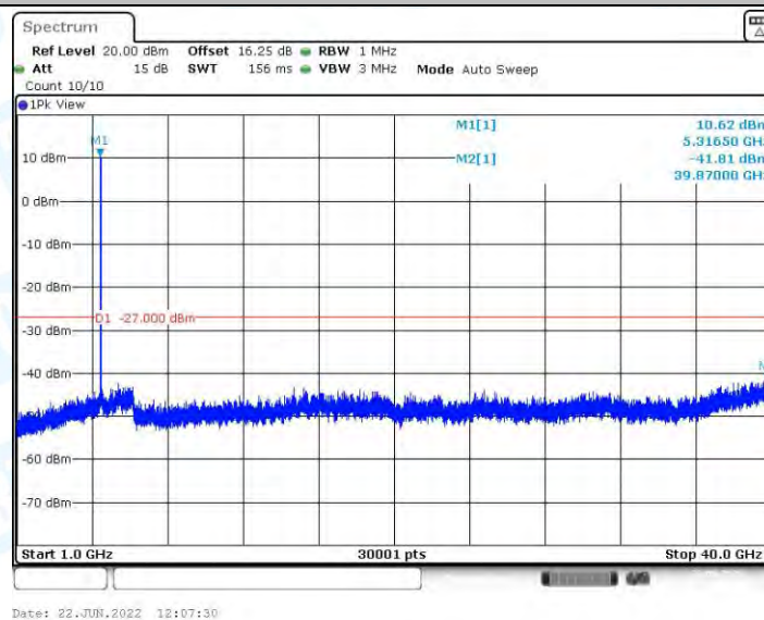
11AC20MIMO_Ant2_5320_1000~40000
