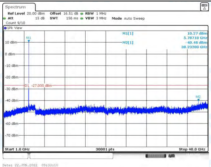
11N20MIMO_Ant2_5785_1000~40000
