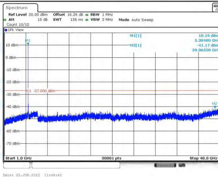
11AC20MIMO_Ant1_5300_1000~40000
