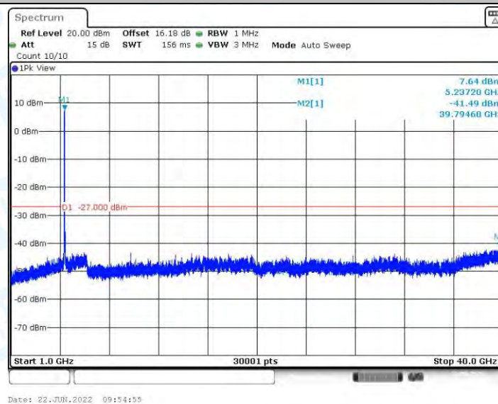
11N40MIMO_Ant1_5230_1000~40000
