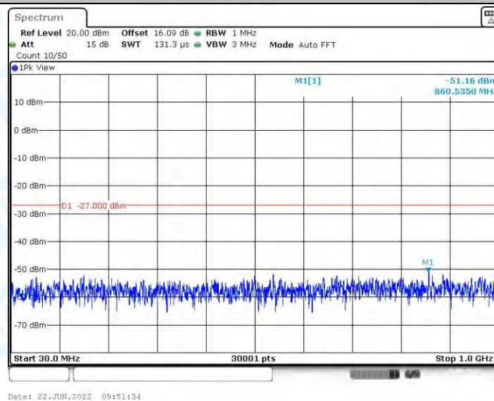
11N40MIMO_Ant2_5190_30~1000
