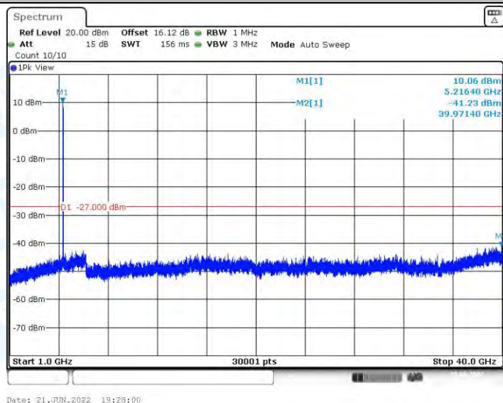
11N20MIMO_Ant2_5220_1000~40000
