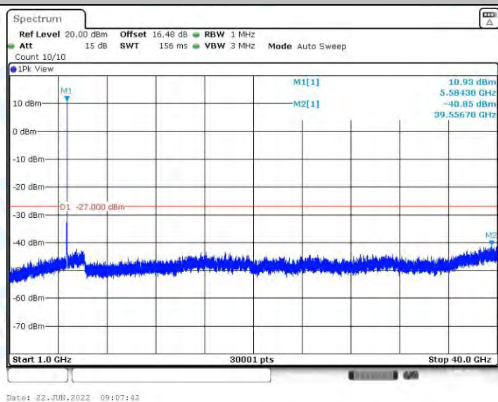
11N20MIMO_Ant1_5580_1000~40000
