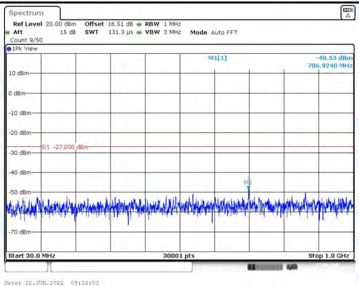
11N20MIMO_Ant2_5785_30~1000
