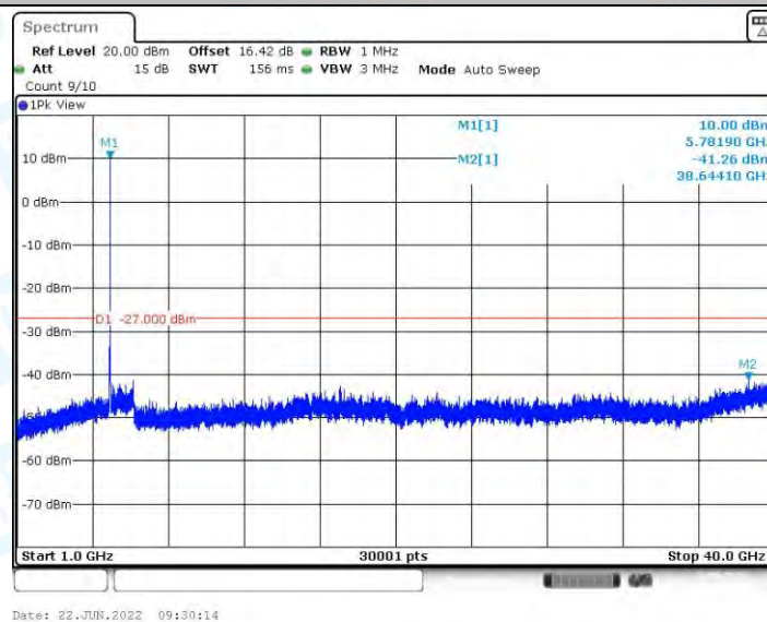
11N20MIMO_Ant1_5785_1000~40000
