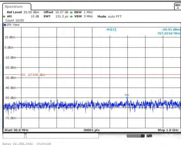
11AC20MIMO_Ant2_5825_30~1000
