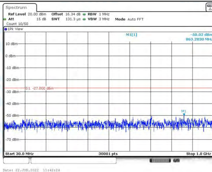
11AC20MIMO_Ant2_5260_30~1000
