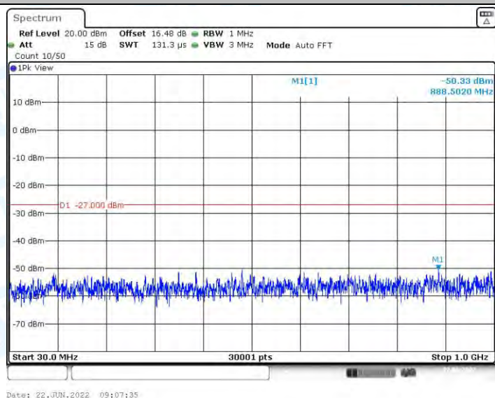
11N20MIMO_Ant1_5580_30~1000
