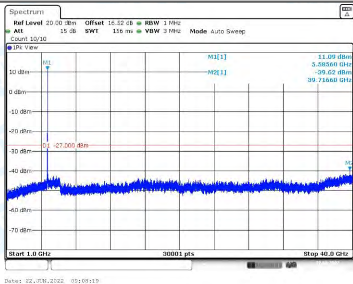
11N20MIMO_Ant2_5580_1000~40000
