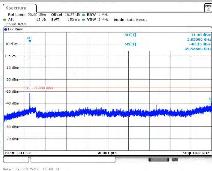
11AC20MIMO_Ant2_5825_1000~40000
