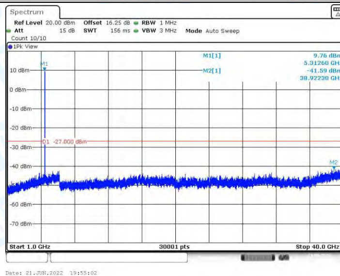
11N20MIMO_Ant2_5320_1000~40000
