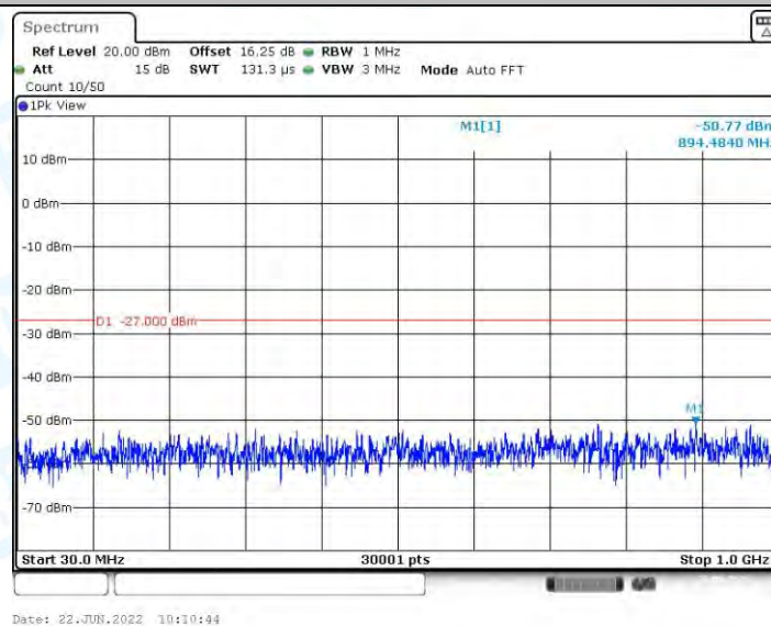
11N40MIMO_Ant2_5310_30~1000
