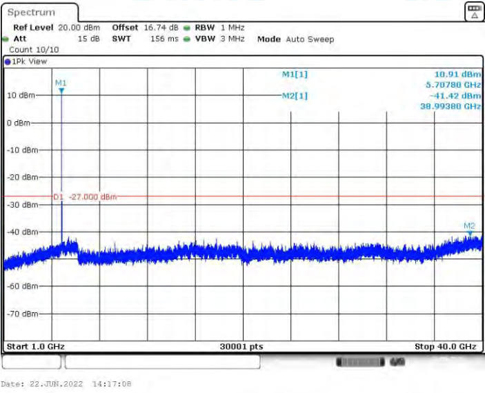
11AC20MIMO_Ant2_5700_1000~40000
