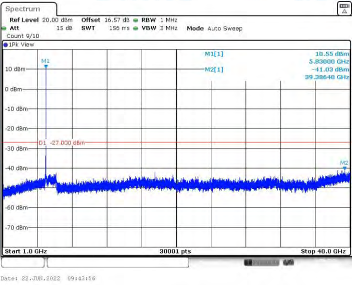
11N20MIMO_Ant2_5825_1000~40000
