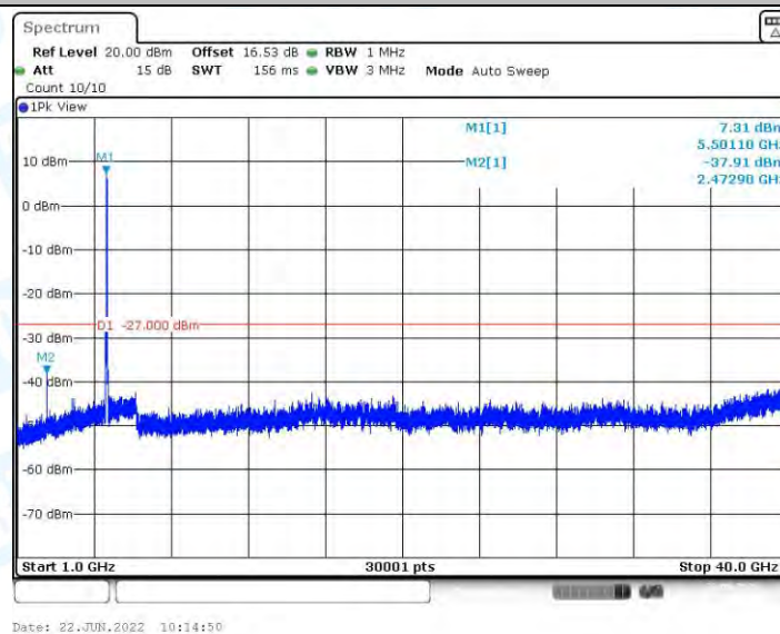
11N40MIMO_Ant1_5510_1000~40000
