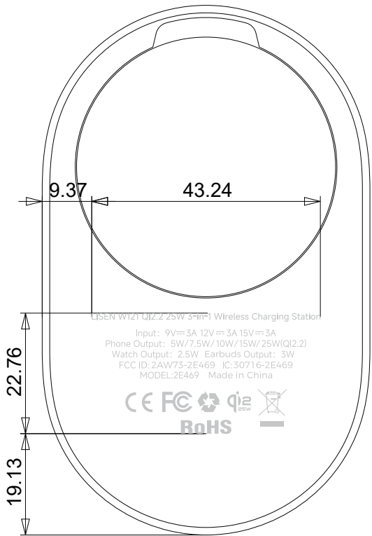
手机充位置背面
