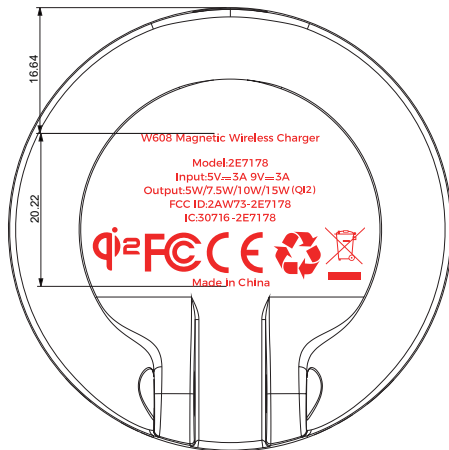
镭雕位置示意
