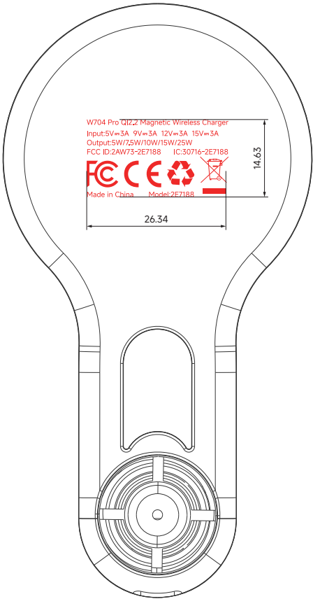
丝印内容位置示意
