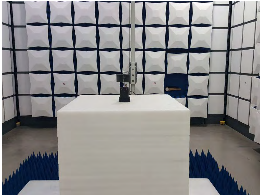
Above 1000MHz
