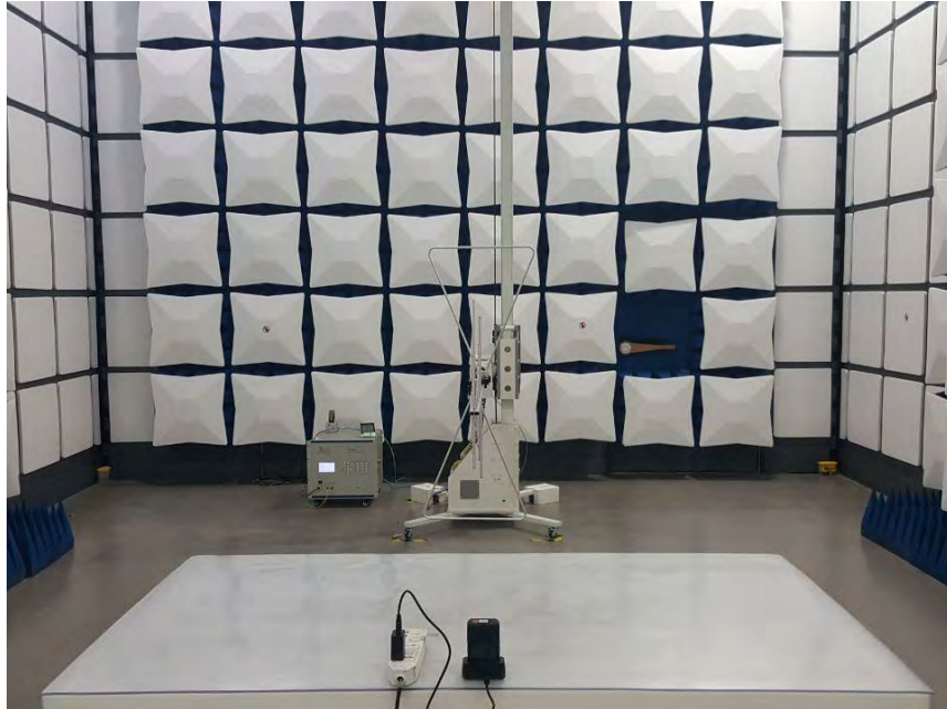
30MHz-1000MHz
