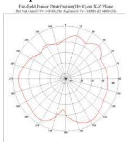
XZ-plane
