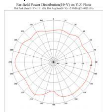
YZ-plane
