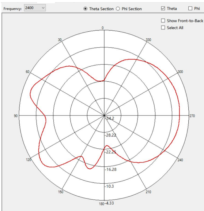
Vertical:2400MHz
