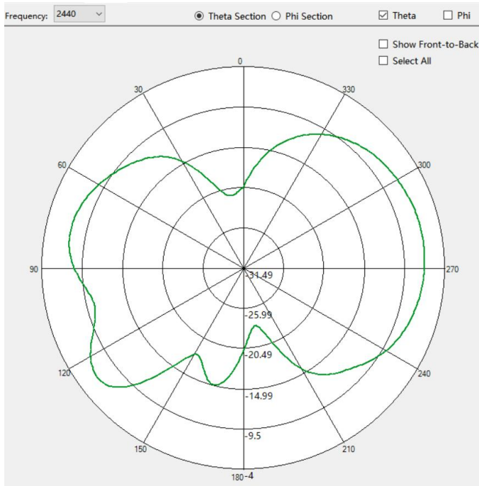
Vertical:2440MHz
