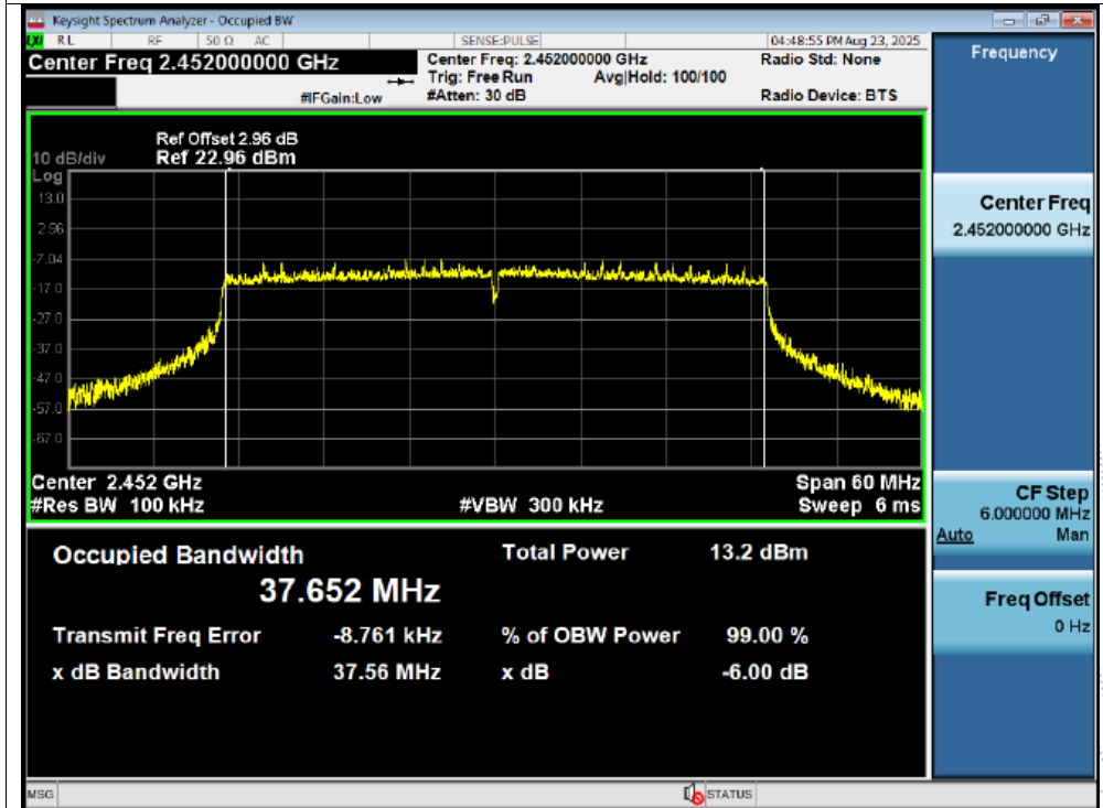
-6dB Bandwidth NVNT ax40 2452MHz Ant1
