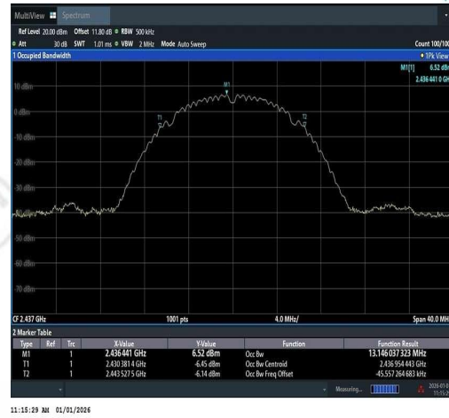
11B-Ant1-2437
