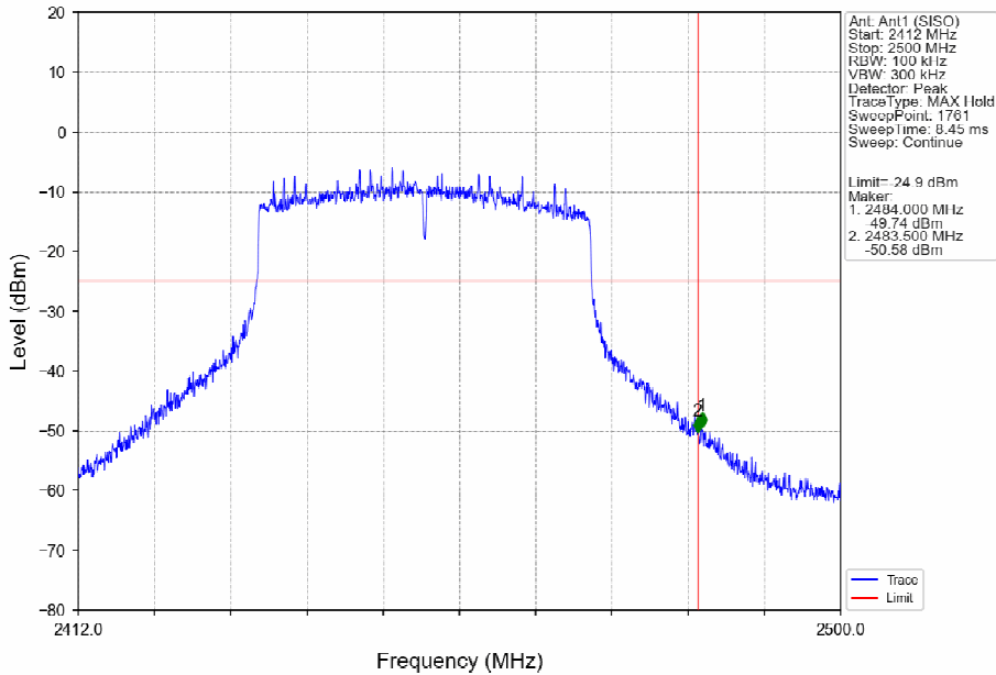
802.11ax(HEW40)_HCH_2452MHz_SU_/_Ant1 (SISO)_NTNV
