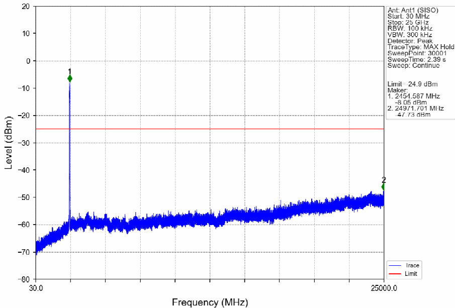
802.11ax(HEW40)_HCH_2452MHz_SU_/_Ant1 (SISO)_NTNV
