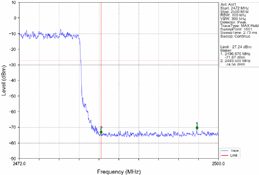
Pi/4DQPSK_2DH5_HOPP_Ant1_NTNV
